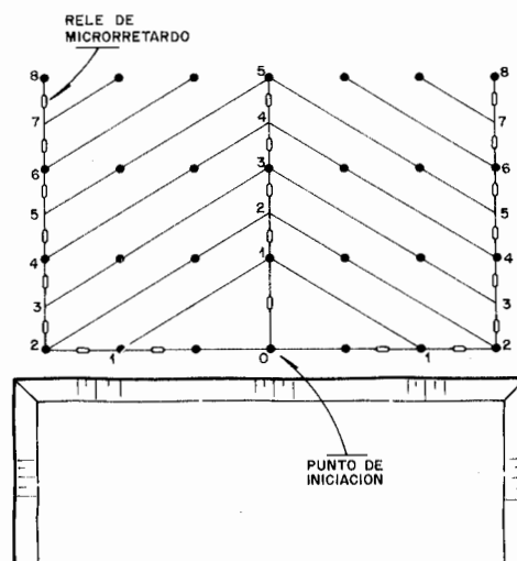
Figura 21.4. Esquema rectangular con secuencia de encendido en «V1».
