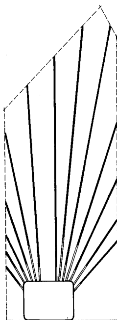
Figura 24.15. Explotación por subniveles con barrenos en abanico.
