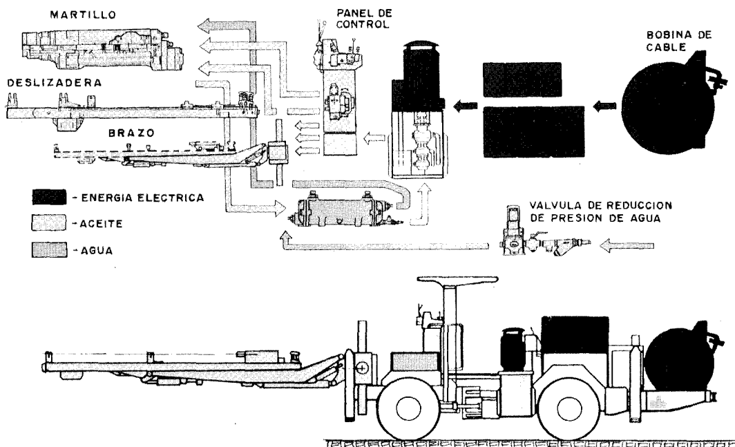
Figura 2.19. Componentes principales de un jumbo (Tamrock).
