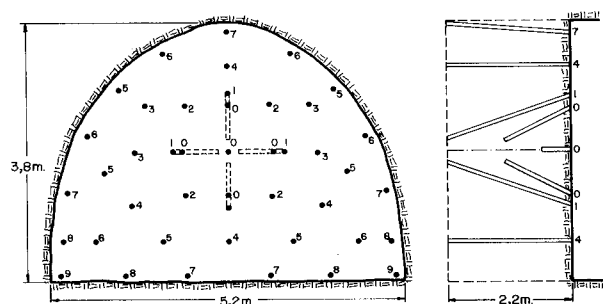
Figura 22.27. Voladura con cuele instantáneo piramidal.
