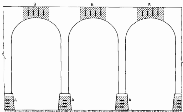
Figura 31.14. Zonas de voladura en un puente de mampostería.
