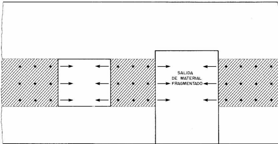
Figura 31.18. Perforación de un muro de ladrillos (Langa).
