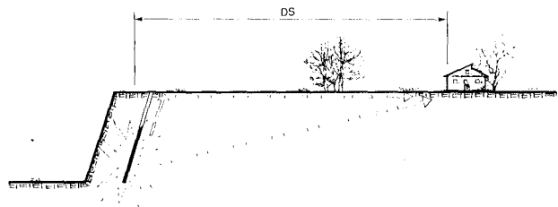
Figura 33.24. Distancia de la voladura al punto de registro.
