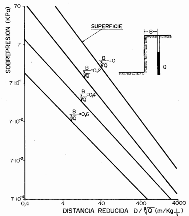
Figura 33.27. Predicción de la sobrepresión aérea a partir de la geometría y carga de las voladuras.
