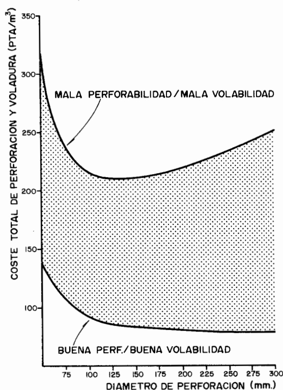
Figura 32.5. Evolución de los costes totales de perforación y voladura en función del diámetro de perforación.
