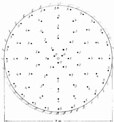
Figura 23.7. Método de barrenos paralelos.
