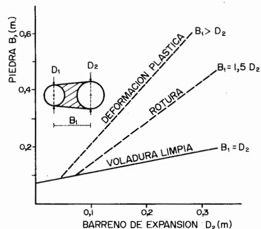
Figura 22.6. Resultados de las voladuras para diferentes distancias de los barrenos cargados a los vacíos y diámetros de éstos.
