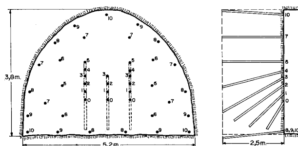
Figura 22.26. Voladura con cuele en abanico al piso.
