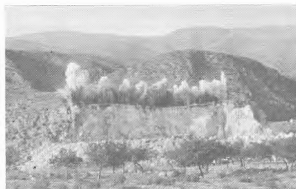
Foto 20.1. Voladura en banco de una cantera.
