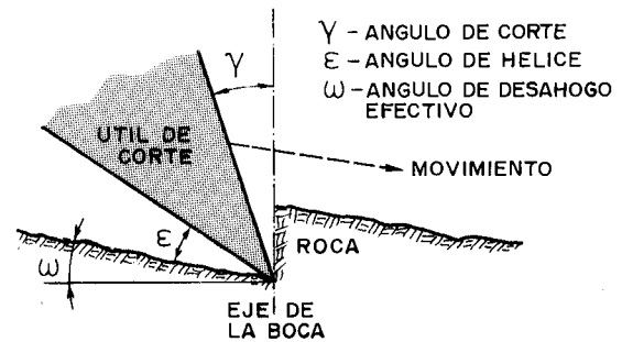
Figura 6.8. Trayectoria de un punto de la boca (Fairhurst, 1964).
