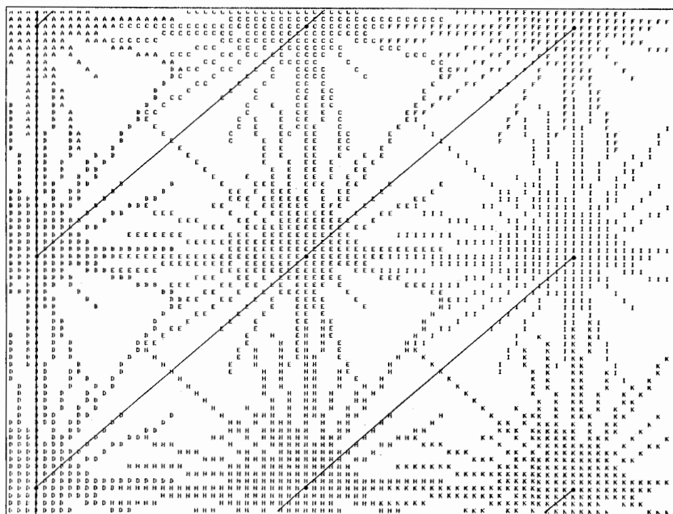
Figura 32.15. Representación gráfica de las grietas originadas alrededor de cada barreno para un esquema y secuencia de encendido determinados.
