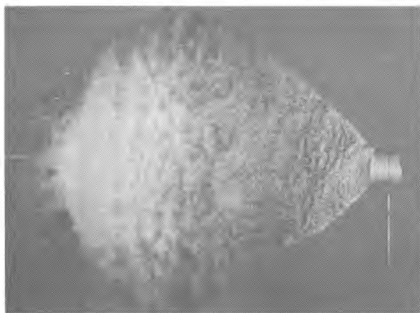
Foto 9.1. Detonación de una carga sin confinar (Nitro-Nobel).
