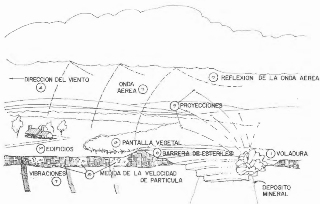
Figura 33.1. Perturbaciones originadas por las voladuras de rocas.
