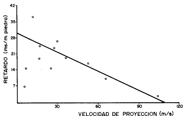
Figura 27.19. Correlación del retardo medio entre filas con la velocidad de los fragmentos de roca proyectados.
