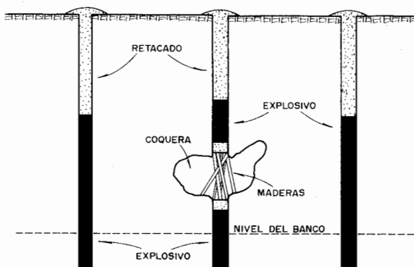
Figura 18.13. Sistema de carga en un barreno que intersecta una gran coquera (Hagan y Reid).
