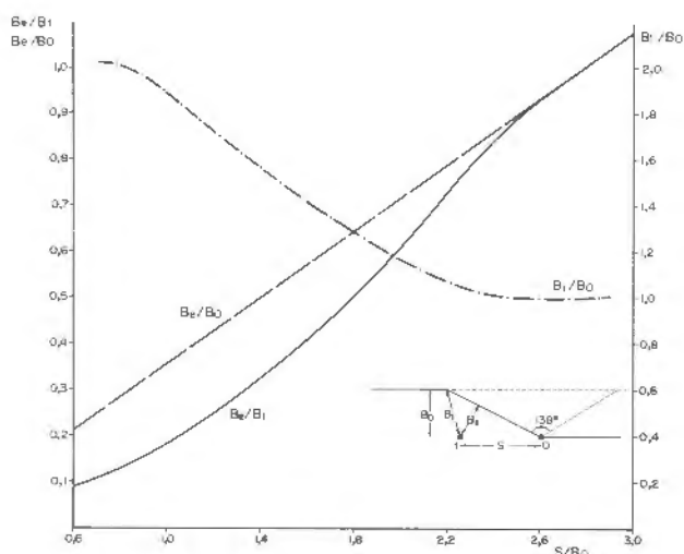
Figura 27.4. Variación de las relaciones de la piedra con el espaciamiento entre barrenos.
