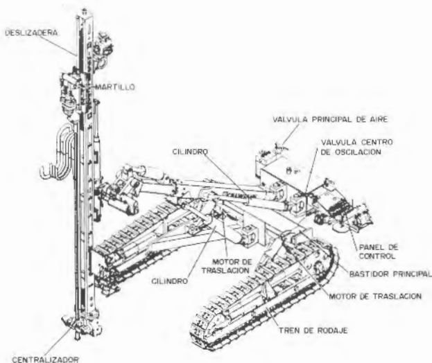
Figura 2.30. Carro de orugas neumático (Ingersoll-Rand).
