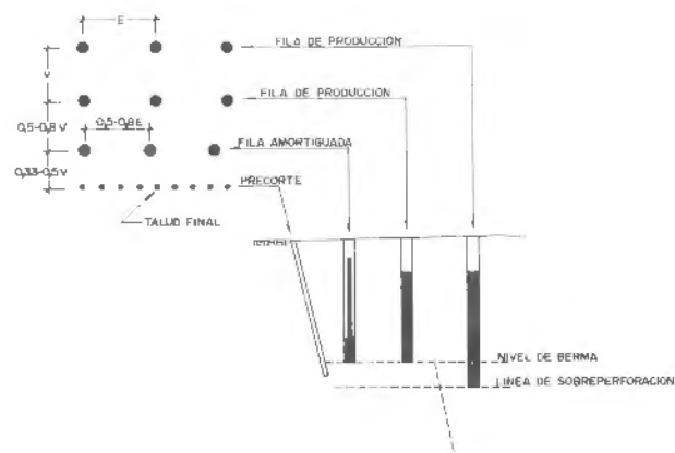
Figura 25.22. Diseño de voladura de destroza próxima a la línea de precorte.
