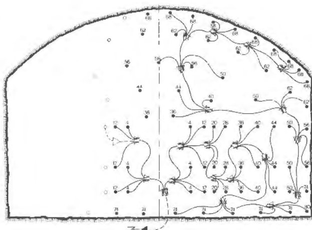
Figura 13.2. Esquema de encendido con detonadores Nonel y conectores.
