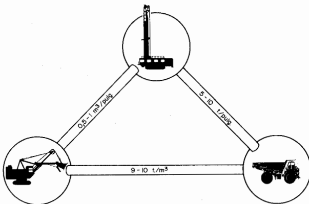
Figura 19.4. Triángulo de dimensionamiento de los equipos de perforación, carga y transporte.
