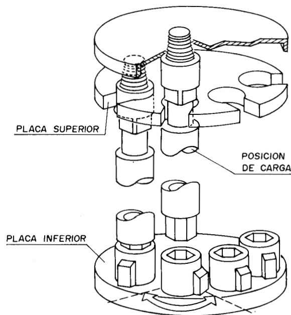
Figura 4.7. Cambiador de barras de tipo revólver.
