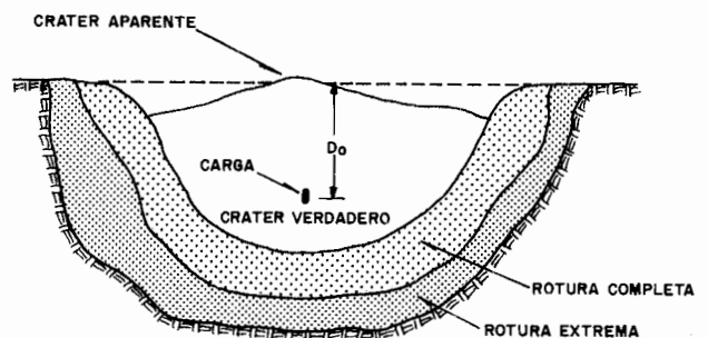
Figura 24.3. Zonas de un cráter.
