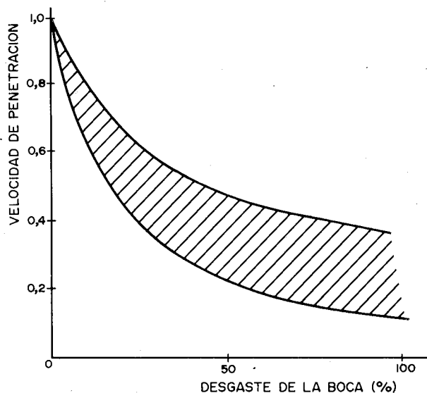
Figura 4.18. Efecto del desgaste de la boca sobre la velocidad de penetración.
