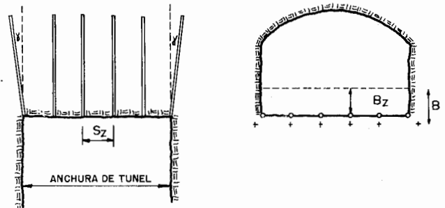
Figura 22.15. Geometría de los barrenos de zapatera.
