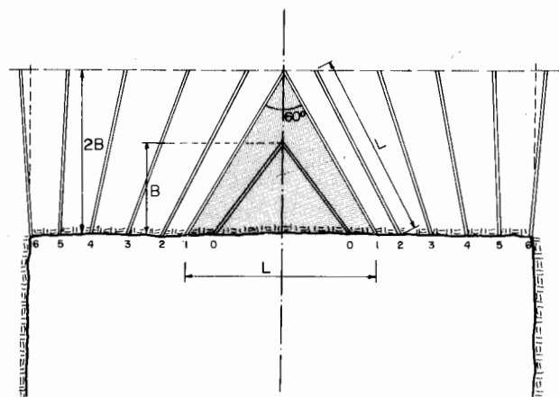
Figura 22.24. Voladura con cuele en cuña.
