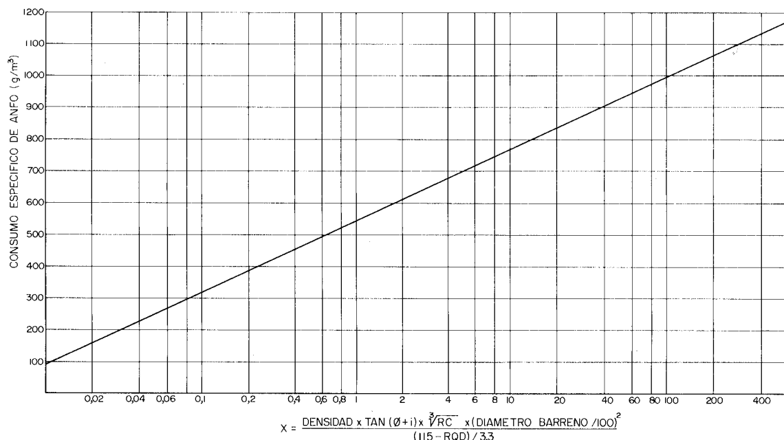
Figura 18.2. Cálculo del Consumo Específico de explosivo en función de diversos parámetros geomecánicos del macizo rocoso.
