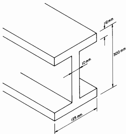
Figura 31.23. Dimensiones del perfil metálico.
