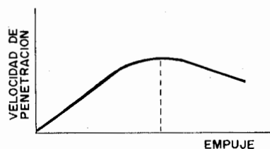
Figura 2.4. Influencia del empuje sobre la velocidad de penetración.
