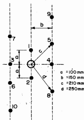
Figura 22.14. Cuele Fagersta.
