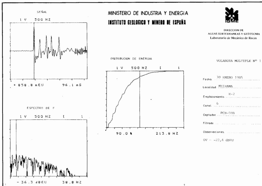
Figura 33.29. Ejemplo de registro de vibraciones obtenido en una voladura para una componente.
