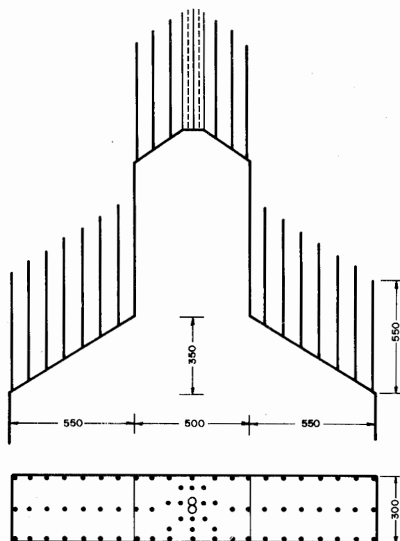
Figura 22.30. Secuencia de avance para explotación por cámaras y pilares.
