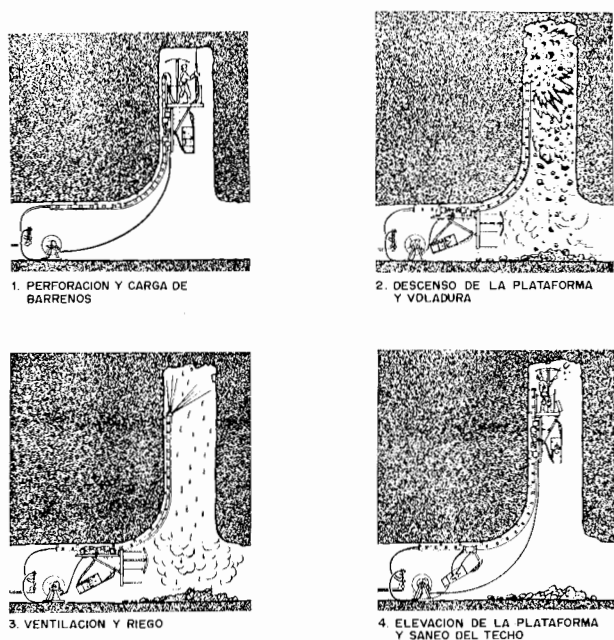
Figura 7.7. Ciclo de trabajo con plataforma Alimak.
