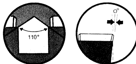
Figura 3.23. Afilado de pastillas.
