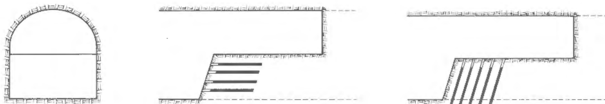
Figura 22.2. Banqueo vertical u horizontal en un túnel con avance en dos secciones.
