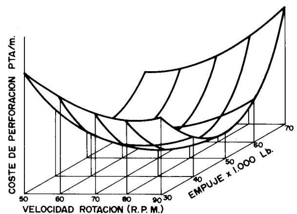
Figura 18.6. Efecto del empuje y la velocidad de rotación sobre el costo de perforación.
