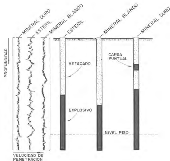
Figura 18.11. Diagrama de la velocidad de penetración y distribución de carga en los tipos de roca de la Fig. 18.10 (Hagan y Reid).
