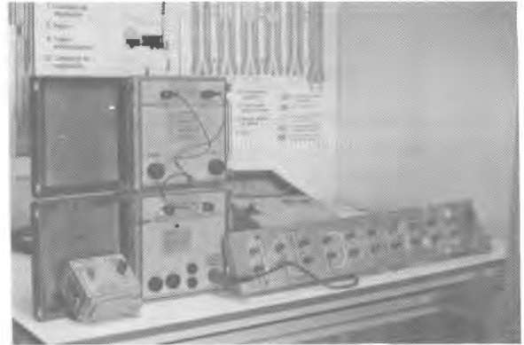
Foto 13.6. Explosor secuencial.
