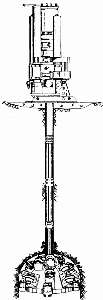
Figura 7.11. Perforación de una chimenea con Raise Boring Estándar.
