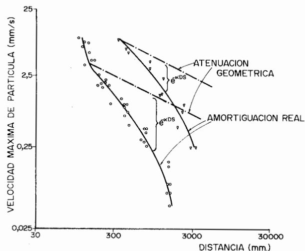
Figura 33.23. Leyes de propagación de las vibraciones con amortiguaciones geométricas y atenuaciones inelásticas exponenciales.
