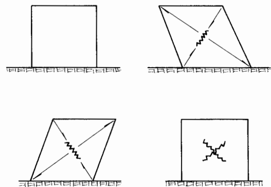
Figura 33.37. Mecanismo de formación de las grietas en «X».
