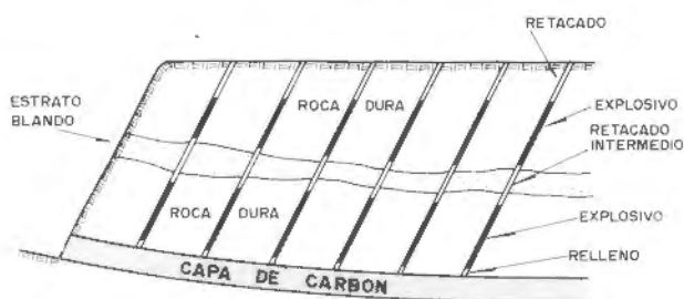
Figura 18.9. Localización del techo de la capa de carbón y empleo de retacados intermedios al nivel de una intercalación blanda.
