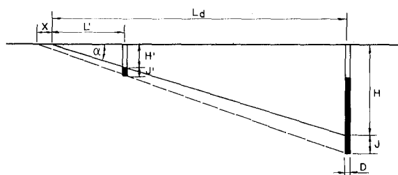
Figura 21.11. Esquema longitudinal de una rampa.
