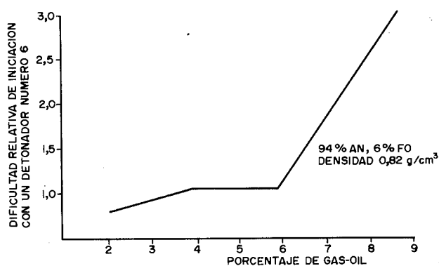
Figura 11.5. Sensibilidad del ANFO a la iniciación.
