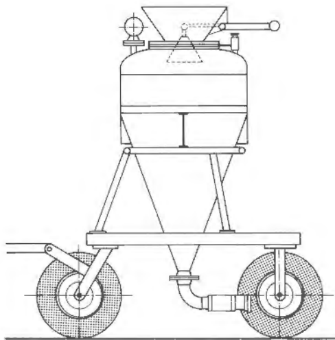
Figura 15.3. Esquema de una cargadora neumática.
