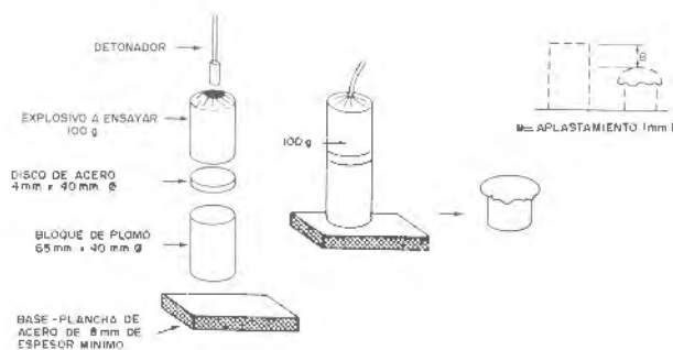
Figura 10.3. Ensayo Hess.
