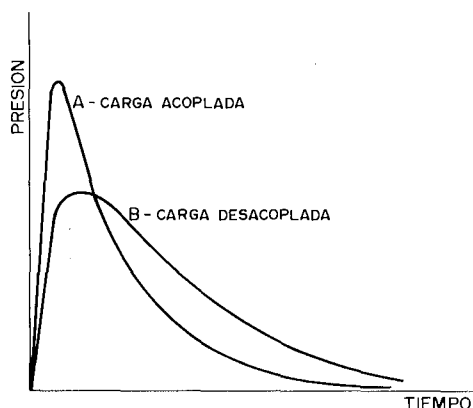
Figura 19.22. Curvas Presión - Tiempo con o sin desacoplamiento de las cargas.
