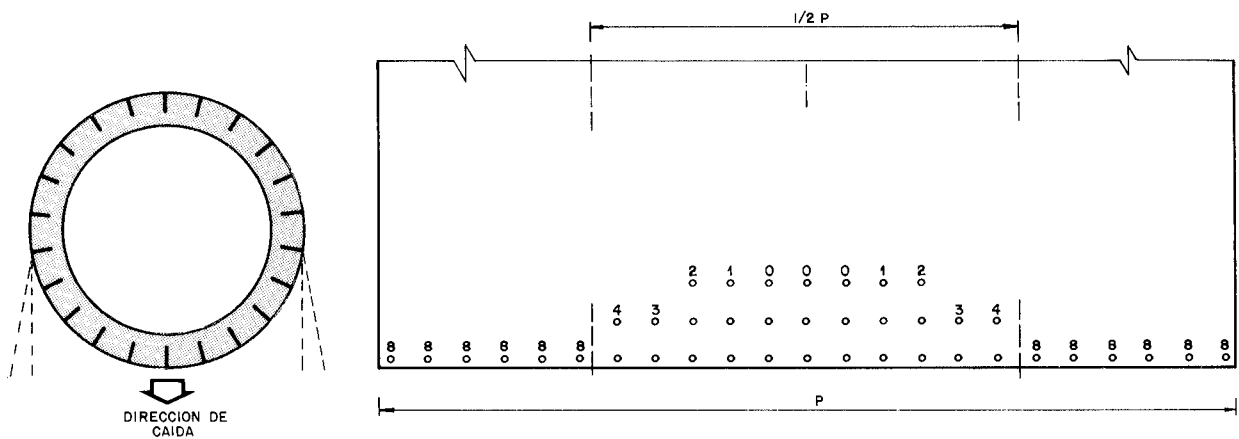
Figura 31.10. Demolición de una chimenea con caída reducida.
