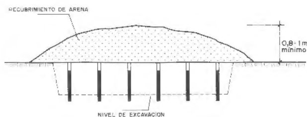
Figura 34.7. Protección de una voladura en zanja mediante una cubierta de arena.
