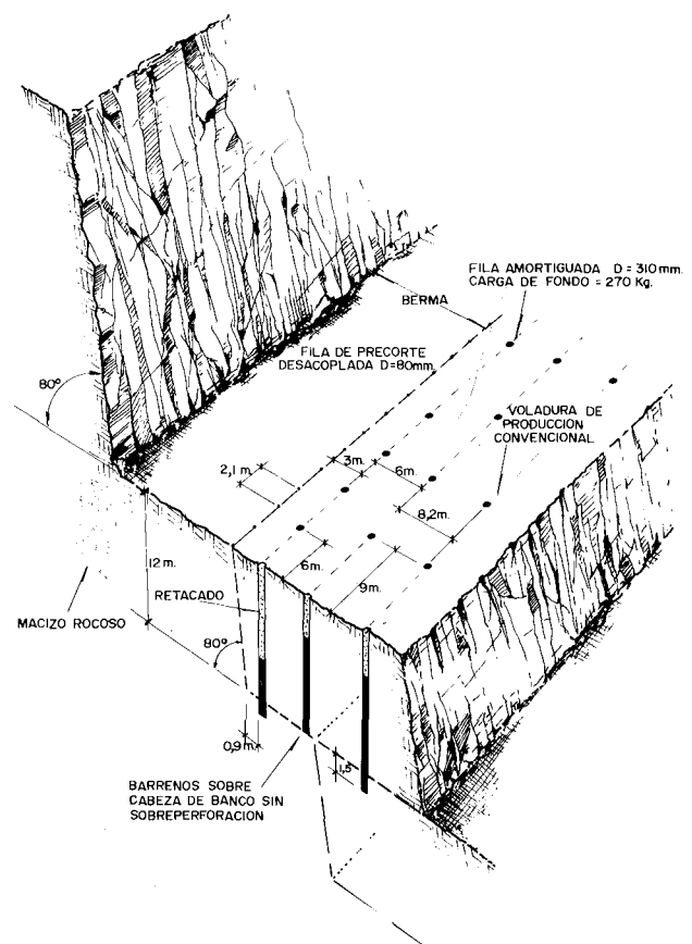
Figura 25.3. Ejemplo de voladura de precorte.
