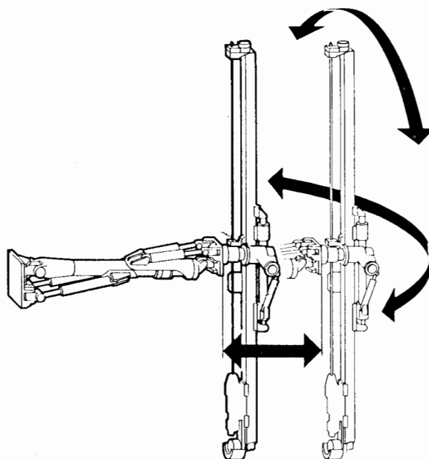
Figura 2.23. Brazo extensible con giro en línea (Atlas Copco).
