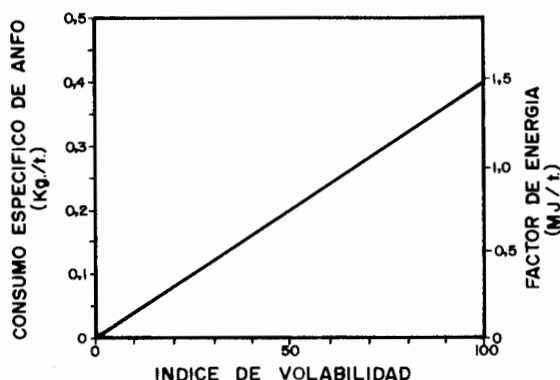
Figura 18.3. Cálculo de Consumos Específicos o Factores de Energía a partir del Índice de Volabilidad.
