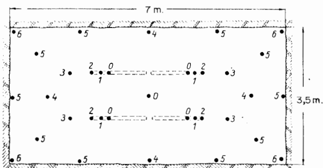
Figura 23.3. Esquema de perforación en pozo de sección rectangular.
