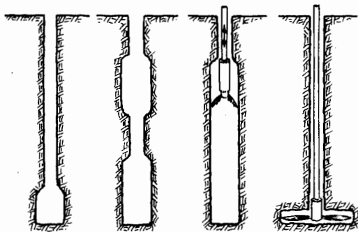
Figura 7.16. Ensanchamiento de barrenos.
