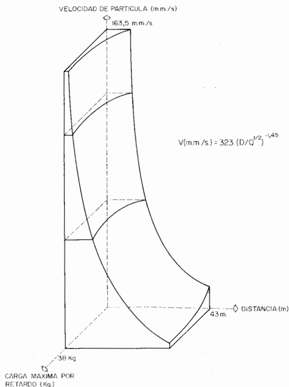
Figura 33.19. Representación tridimensional de una ley de propagación de vibraciones.
