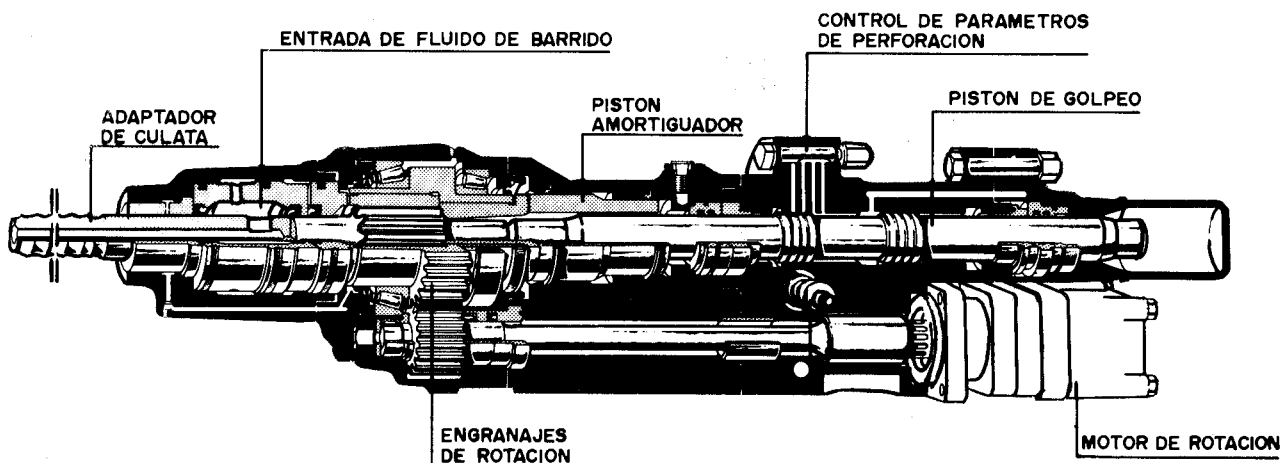
Figura 2.8. Sección de un martillo hidráulico (Atlas Copco).
