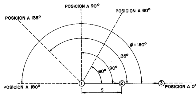
Figura 33.6. Posiciones relativas de los puntos de registro. (Wiss y Linehan).
