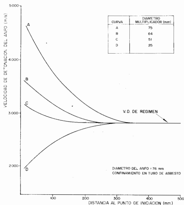
Figura 14.2. Efecto del diámetro del iniciador sobre la velocidad inicial del ANFO (Junk, 1972).
