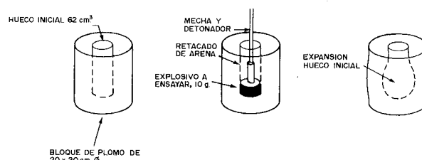
Figura 10.1. Ensayo Traulz.
