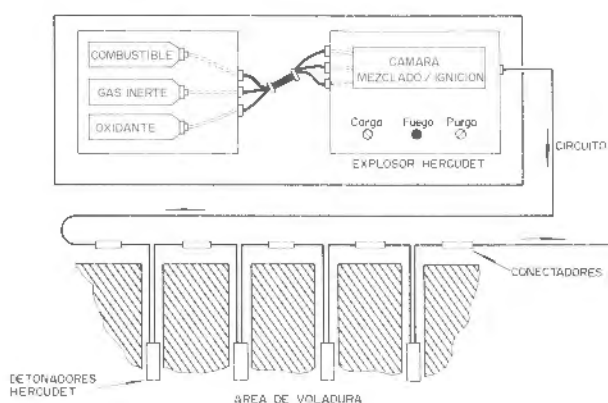
Figura 13.4. Esquema de circuito con detonadores Hercudet.
