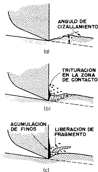
Figura 6.2. Secuencia de corte (Fish y Barker, 1956).
