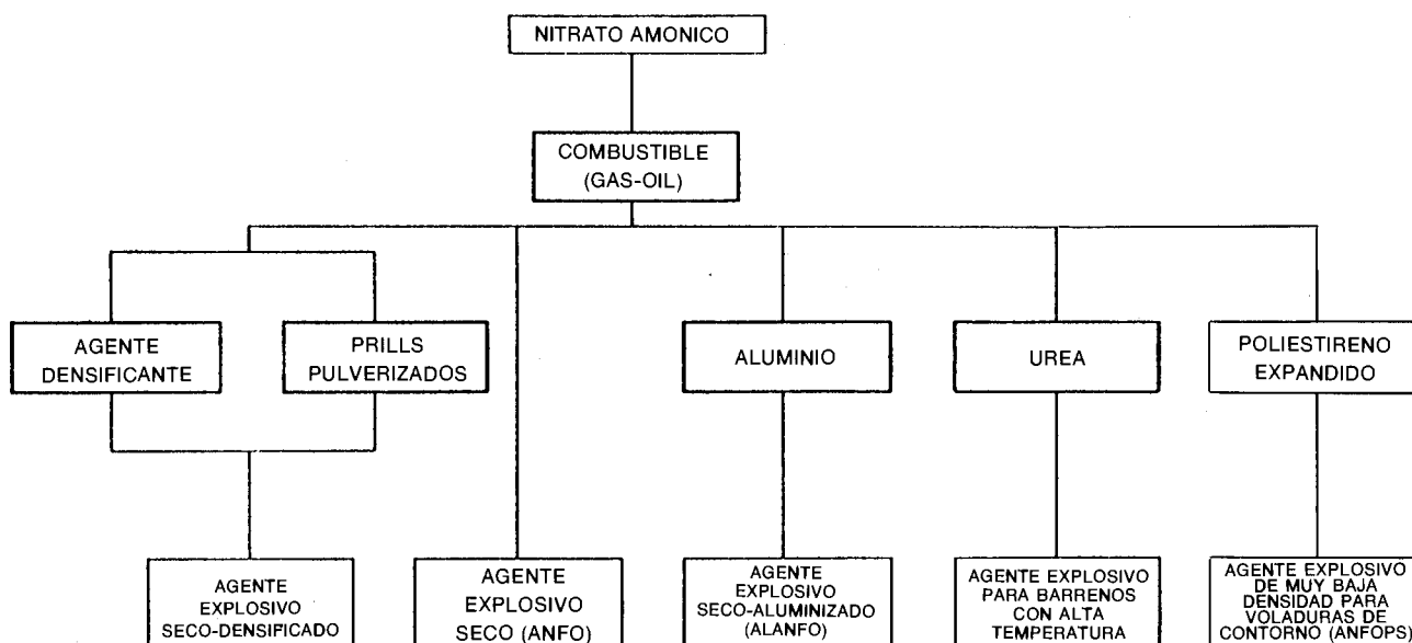
Figura 11.1. Agentes explosivos secos con base Nitrato Amónico.
