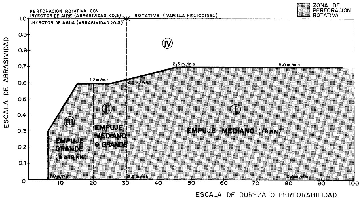
Figura 6.6. Clasificación de las rocas según su perforabilidad y abrasividad (Eimco-Secoma).
