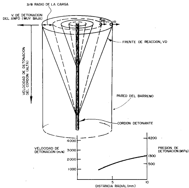
Figura 14.5. Efecto de la detonación de un cordón situado en el eje de un barreno sobre la velocidad de detonación del ANFO.
