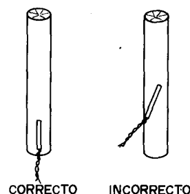
Figura 14.14. Cebado de cartucho con detonador eléctrico.
