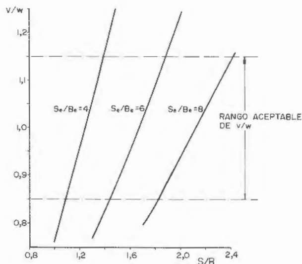
Figura 27.10. Relaciones geométricas de los esquemas rectangulares en «V» con dos frentes libres.
