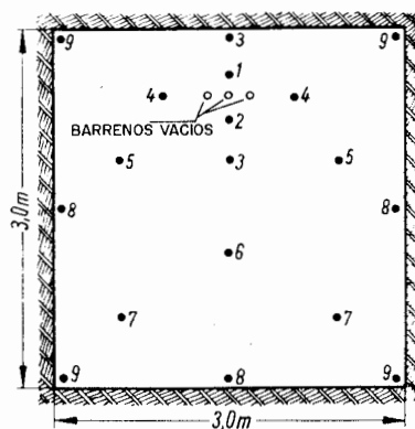
Figura 23.13. Esquema de disparo con barrenos paralelos.
