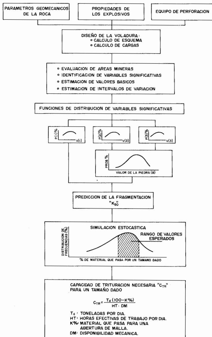
Figura 32.16. Modelo probabilístico de la fragmentación para la selección de la trituradora primaria.
