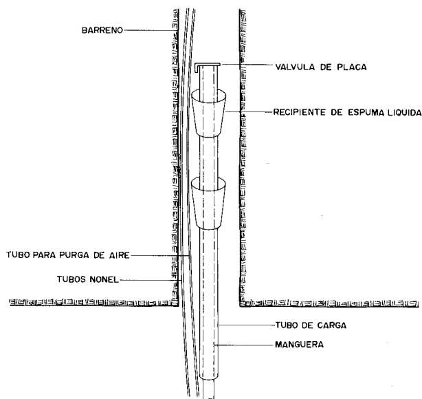
Figura 15.12. Cierre de espuma de poliuretano.
