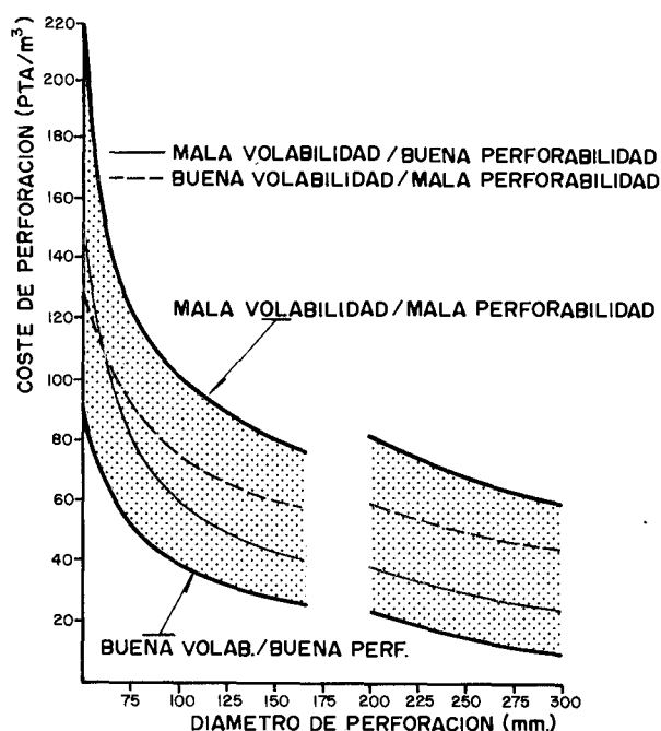
Figura 32.3. Costes de perforación por m^3 de roca volada.
