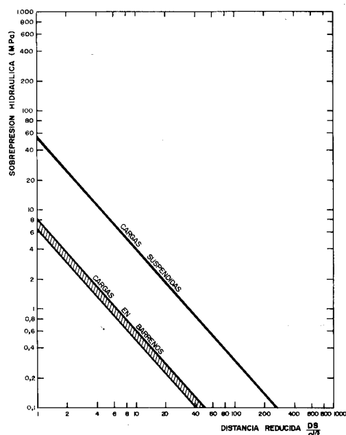
Figura 26.7. Sobrepresión hidráulica producida por cargas suspendidas de TNT dentro del agua y confinadas en barrenos.
