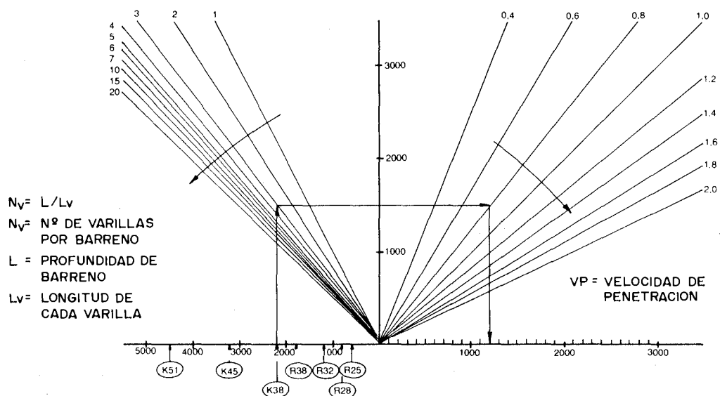
Figura 3.14. Ejemplo de cálculo de vida en servicio del varillaje (Kometa).
