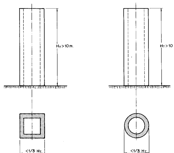
Figura 31.12. Tipos de torres.
