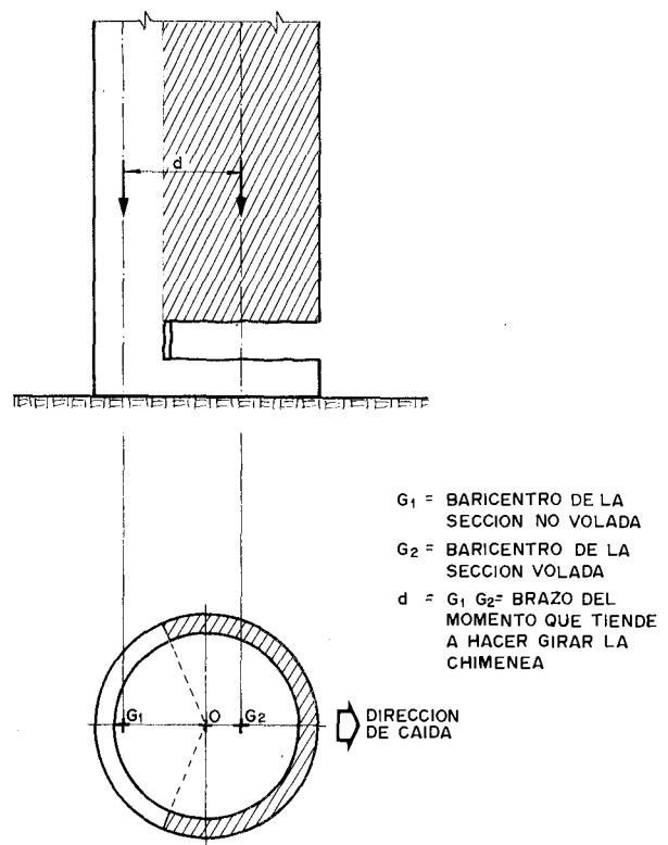
Figura 31.7. Método de demolición de una chimenea.
