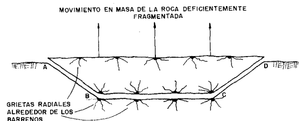
Figura 27.1. Desplazamiento de la roca en una voladura instantánea de una fila (Hagan, 1975).
