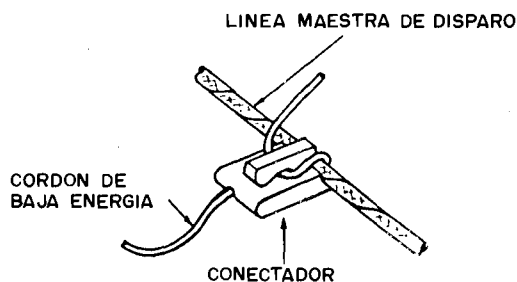
Figura 13.1. Conector de plástico en cordón detonante de muy baja energía.
