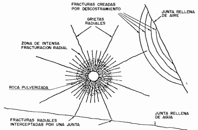
Figura 16.3. Agrietamiento radial y rotura por reflexión de la onda de choque.
