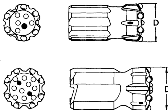
Figura 3.11. Bocas retráctiles.
