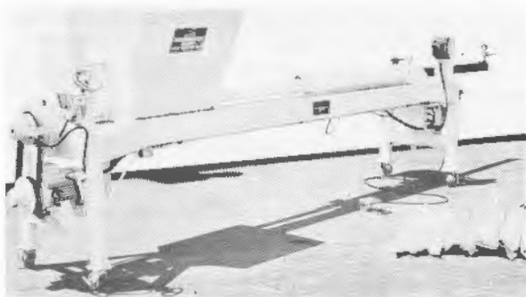
Foto 15.5. Encartuchadora de ANFO (Amerind MacKissic, Inc.).
