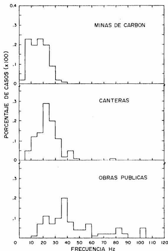
Figura 33.2. Frecuencias dominantes en operaciones de arranque con voladuras (Dowding et al., 1980).
