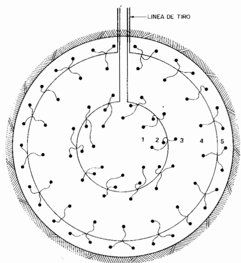
Figura 23.9. Anillos de conexión en una voladura en pozo.
