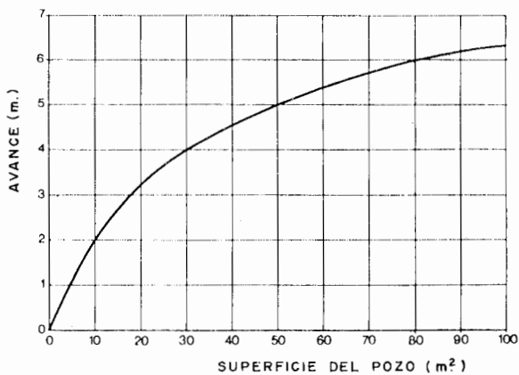
Figura 23.5. Profundidad de las pegas en función de la sección de los pozos.
