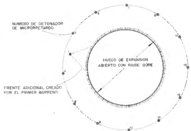
Figura 19.15. Voladura de una chimenea (Hagan).
