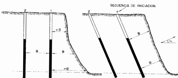
Figura 19.7. Perforación inclinada vs. Perforación vertical.
