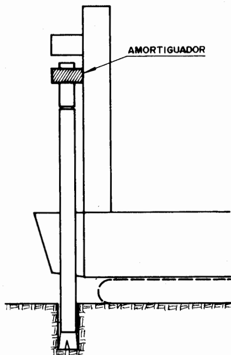
Figura 4.11. Posición de un amortiguador de impactos.
