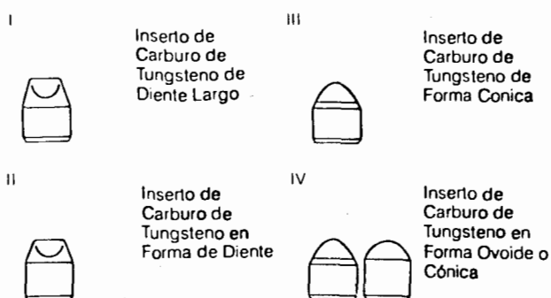
Figura 5.6. Clases de insertos según los tipos de triconos.
