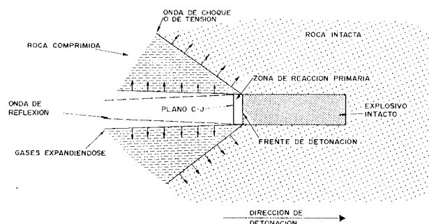
Figura 9.2. Proceso de detonación de una carga explosiva.
