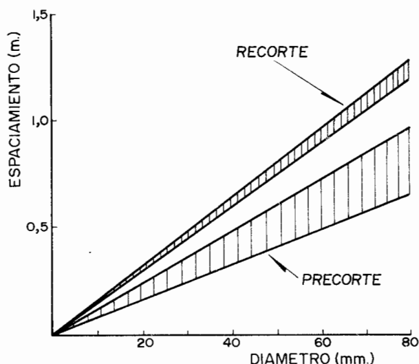
Figura 25.16. Valores recomendados del espaciamento en función del diámetro de perforación para precorte y recorte.
