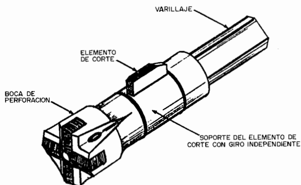
Figura 25.26. Accesorios de perforación para la creación de entalladuras en los barrenos de contorno.
