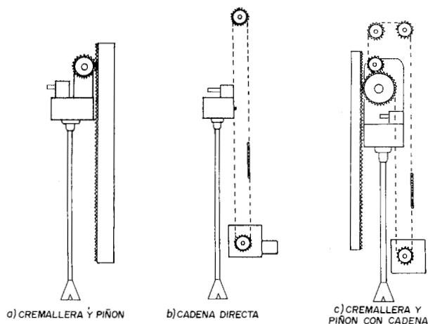
Figura 4.5. Sistemas de elevación y empuje.
