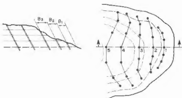
Figura 21.14. Ejemplo de voladura de nivelación.
