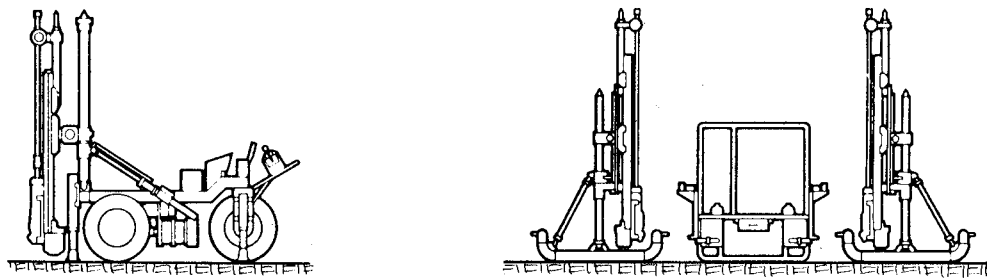
Figura 2.25. Vagón de perforación y equipo sobre patín para la ejecución de barrenos largos (Atlas Copco).
