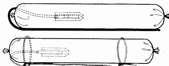
Figura 14.4. Cartuchos-cebo con multiplicador Detaprime (Du Pont).
