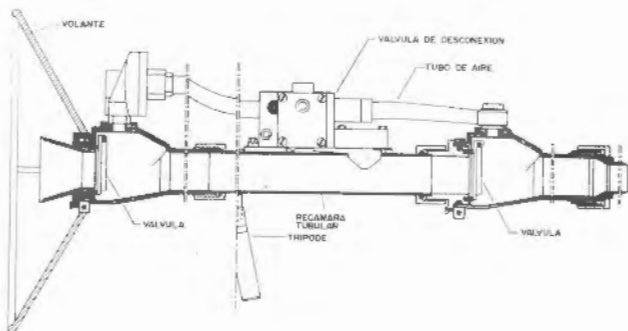
Figura 15.1. Cargadora neumática.
