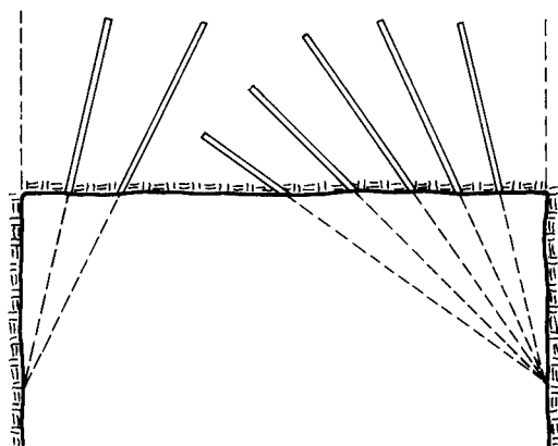
Figura 22.25. Cuele en abanico horizontal.
