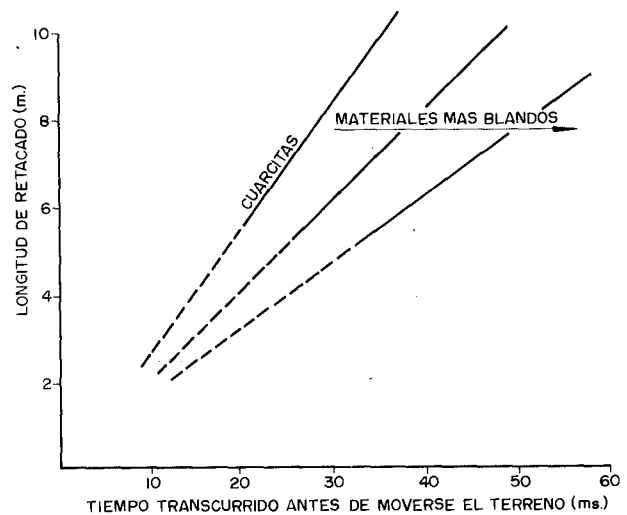
Figura 27.15. Tiempo transcurrido antes de comenzar el movimiento del techo del banco con barrenos de 229 a 381 mm.
