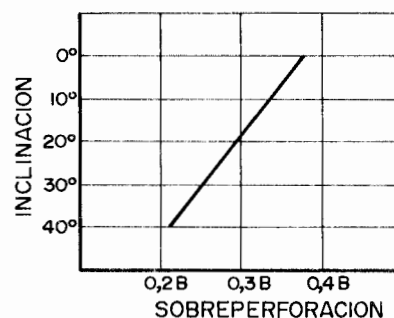
Figura 19.10. Reducción de la sobreperforación con la inclinación de los barrenos.
