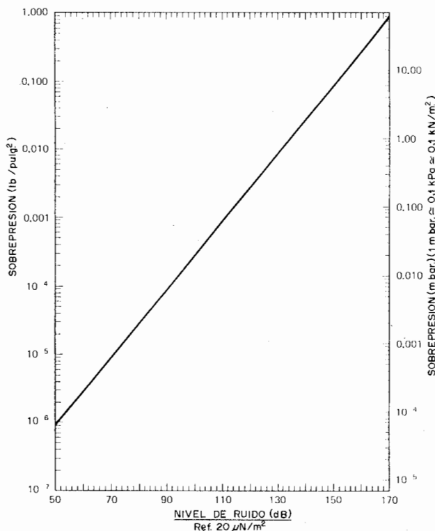
Figura 33.25. Abaco de conversión de sobrepresión a nivel de ruido (Sisking et al., 1980).
