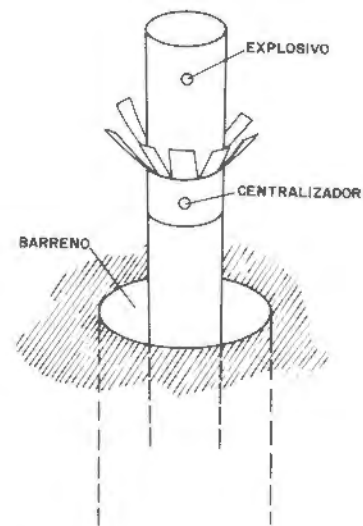
Figura 13.23. Elemento centralizador de cargas de explosivo.
