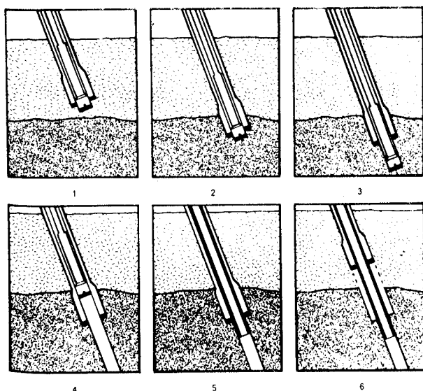
Figura 7.2. Operaciones en el sistema OD.
