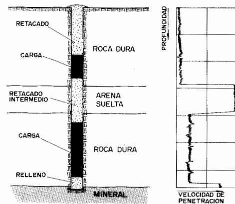
Figura 18.7. Formaciones con resistencias variables (Hagan y Reid).
