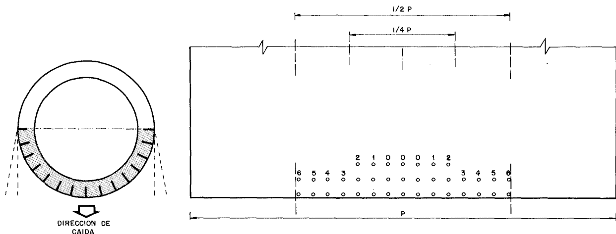
Figura 31.8. Perforación de una chimenea de mampostería.
