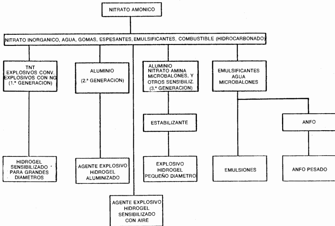
Figura 11.10. Agentes explosivos acuosos producidos a partir del NA.
