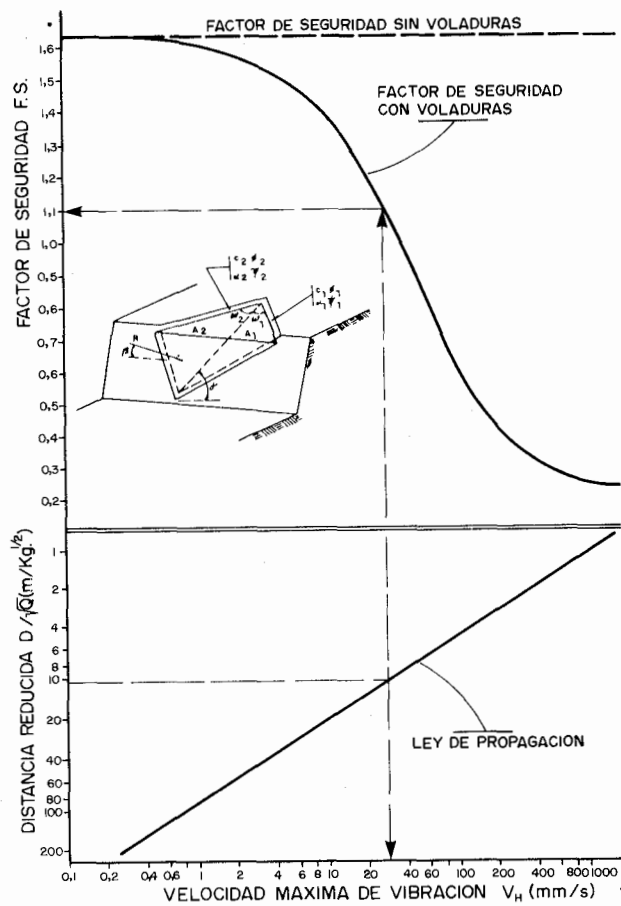
Figura 33.44. Variación del Factor de Seguridad para un bloque de una rotura en cuña en función de la Distancia Reducida.
