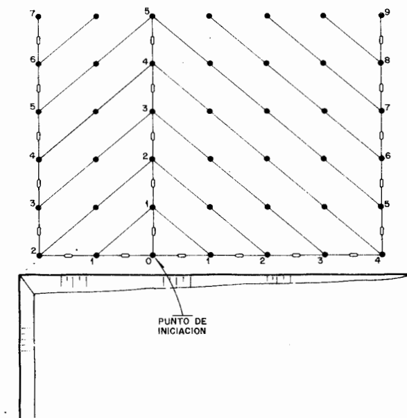
Figura 21.7. Secuencia de encendido en «V» con salida paralela a la traza.
