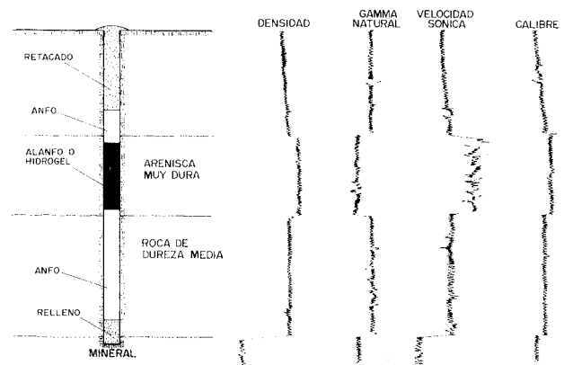
Figura 18.5. Ejemplo de diagramas obtenidos y distribución de cargas de explosivo en presencia de un nivel de roca dura (Hagan y Gibson).
