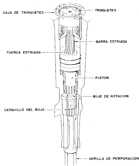
Figura 2.6. Perforadora con rotación por mecanismo de barra estriada.
