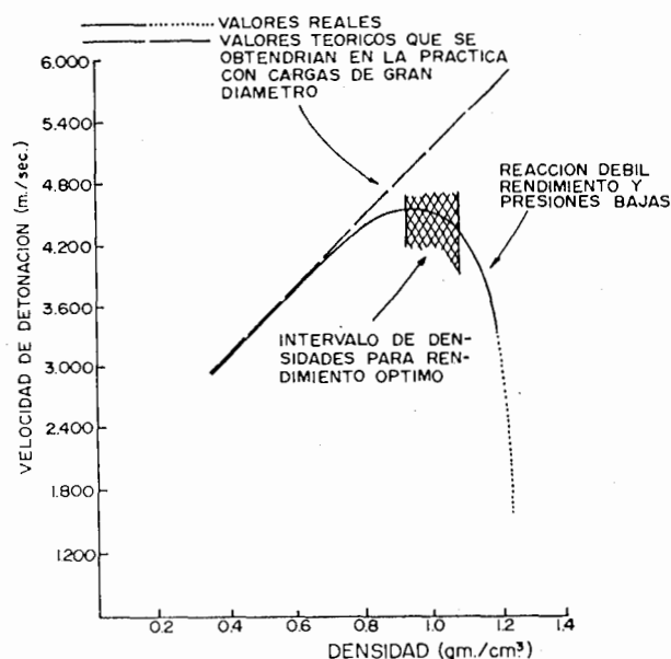
Figura 10.8. Velocidad de detonación del ANFO en función de la densidad.
