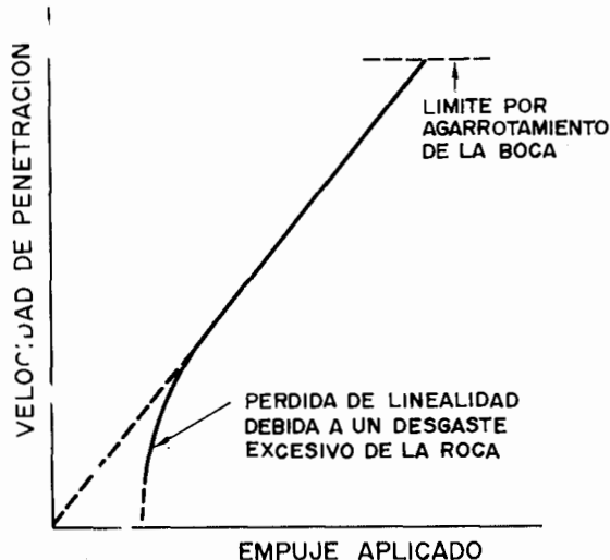
Figura 6.5. Relación entre el empuje y la velocidad de penetración (Fish y Baker, 1956).
