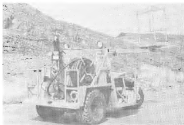
Foto 15.7. Equipo de carga para el avance de galerías (Scoopemóvil - CIL, Inc.).
