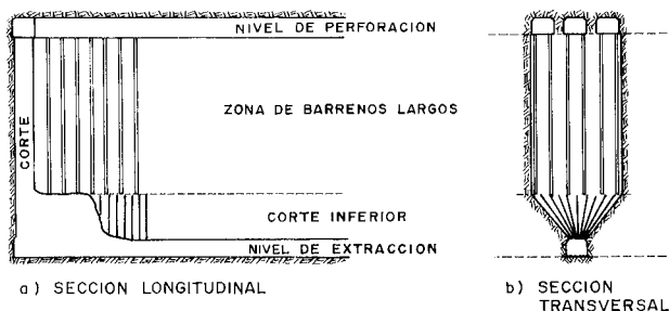
Figura 24.12. Secciones representativas del método de barrenos largos.
