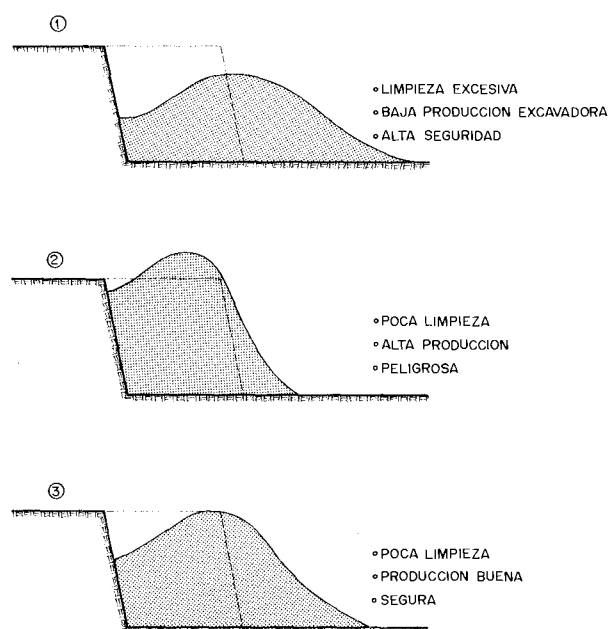
Figura 28.2. Diferentes geometrías de la pila de escombro.
