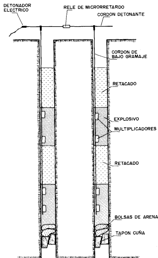
Figura 24.14. Seccionado de cargas.
