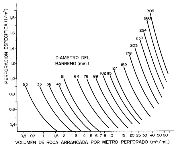
Figura 19.27. Relación entre el rendimiento de arranque y la perforación específica.
