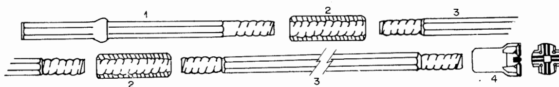
Figura 3.1. Sarta de perforación.
