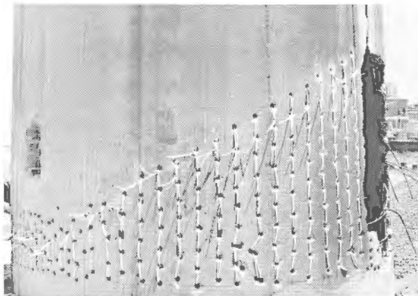
Foto 31.4. Esquema de voladura con cordón detonante de una chimenea de hormigón de reducido espesor. (Cortesía de CAVOSA).
