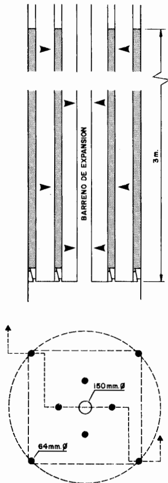
Figura 23.15. Esquema de perforación y secuencia de encendido en chimenea con barreno central de gran diámetro.
