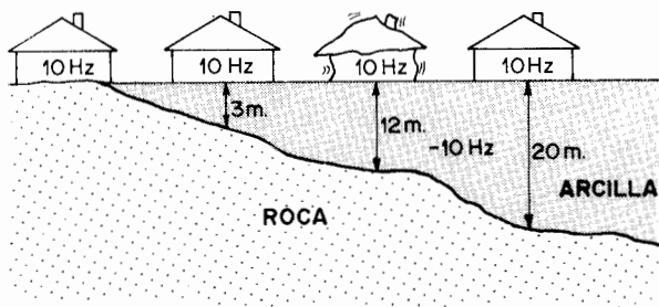
Figura 33.32. Efectos amplificadores cuando la frecuencia natural del edificio coincide con la frecuencia dominante del terreno (Clark et al.).
