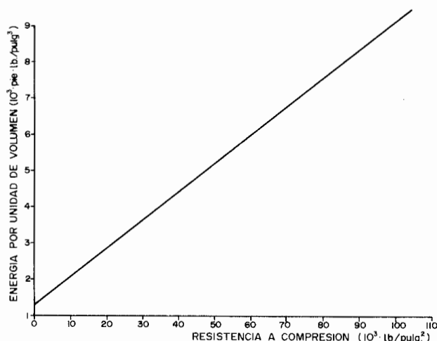
Figura 4.20. Energía de perforación en función de la resistencia a compresión.
