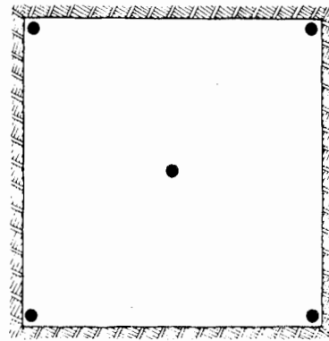
Figura 23.16. Esquema de perforación en el método del cuele cráter.
