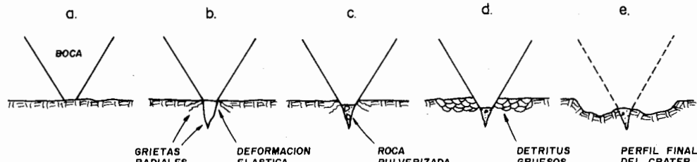
Figura 2.2. Fases de formación de una indentación. (Hartman, 1959).
