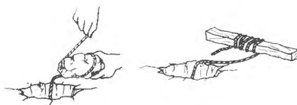
Figura 35.12. Sujeción del extremo del cordón detonante para evitar la caída de éste dentro de los barrenos.
