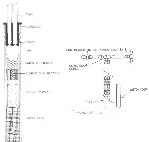
Figura 13.3. Detonador Hercudet y piezas de conexión de tubos.
