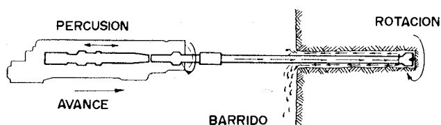
Figura 2.1. Acciones básicas en la perforación rotopercutiva.
