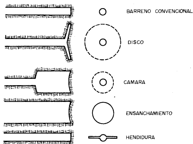
Figura 7.19. Modificación de la geometría de los barrenos perforados con chorro de agua.
