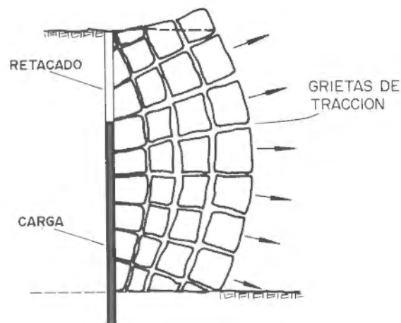
Figura 16.7. Mecanismo de rotura por flexión.
