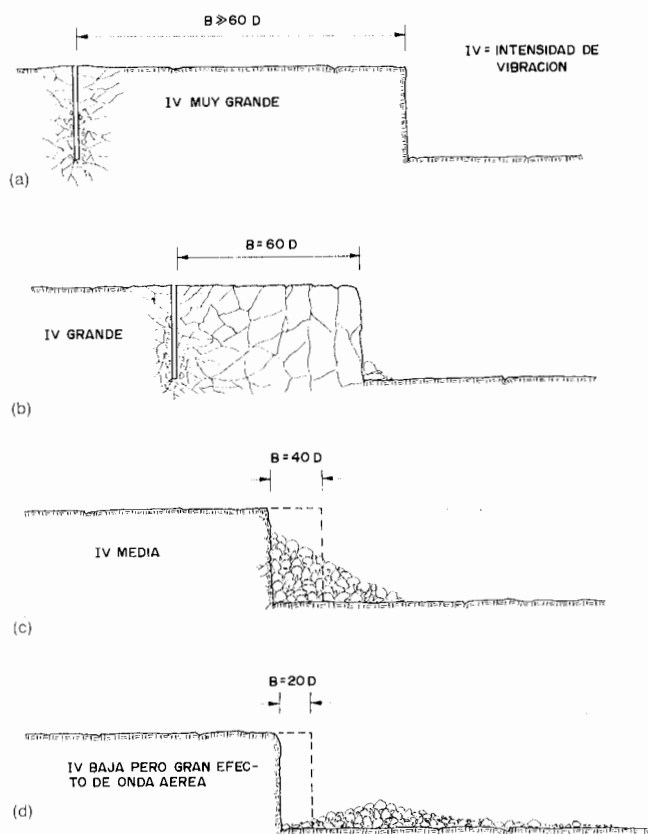
Figura 33.9. Efectos de una carga explosiva según la dimensión de la piedra.
