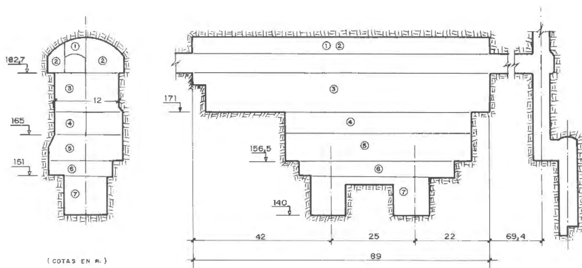
Figura 24.21. Fases de excavación de Aldeadávila II. (Cortesía de Iberduero, S. A.).
