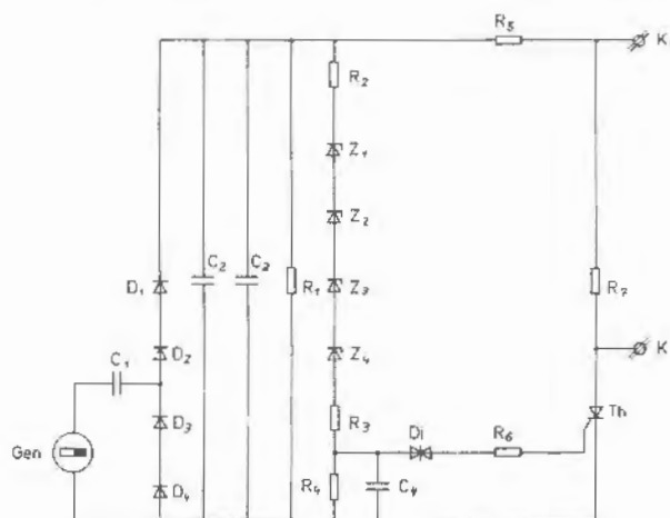
Figura 13.18. Esquema eléctrico de explosor de condensadores.
