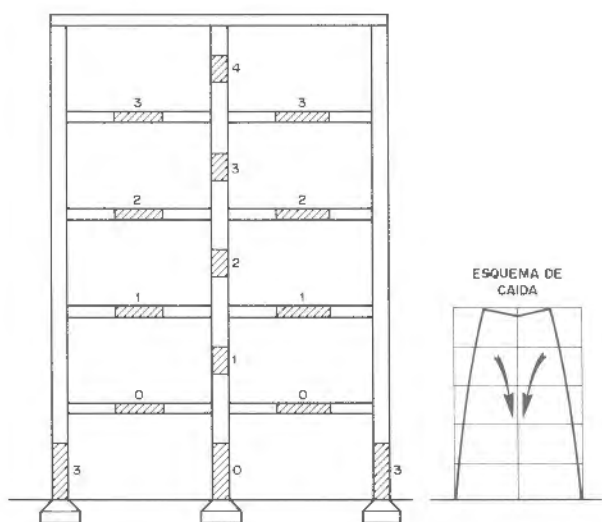
Figura 31.22. Demolición de un edificio con desplome.
