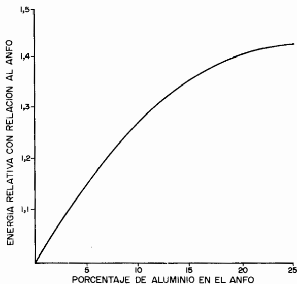
Figura 11.9. Efecto del Aluminio sobre la Energía desarrollada con respecto a una misma cantidad de ANFO.
