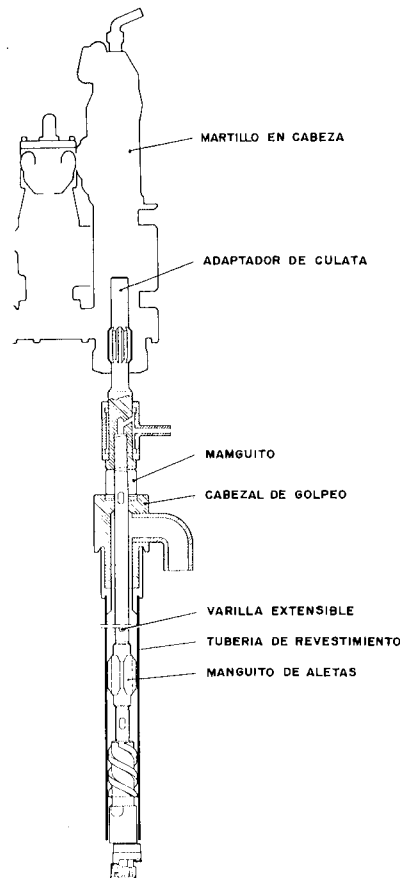
Figura 7.4. Método ODEX con martillo en cabeza (Atlas Copco).
