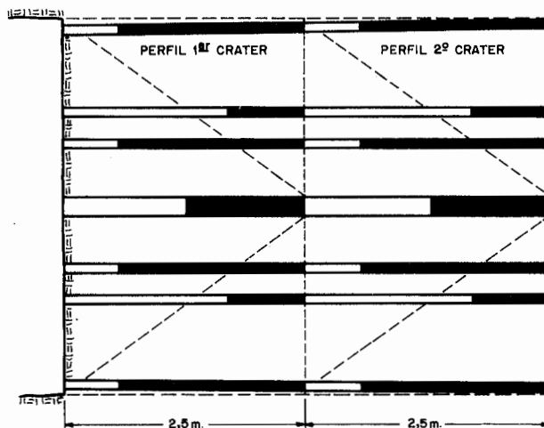
Figura 22.23. Doble cuele cráter usando barrenos centrales de 200 mm.
