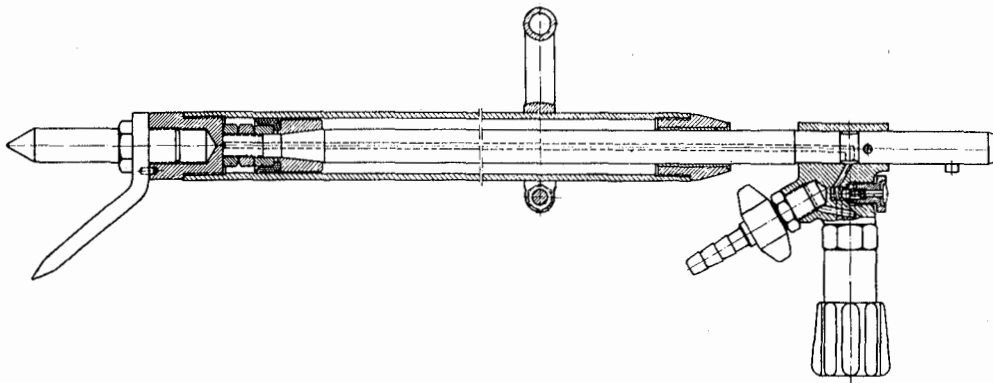
Figura 2.15. Sección de un empujador neumático (Padley & Venables).
