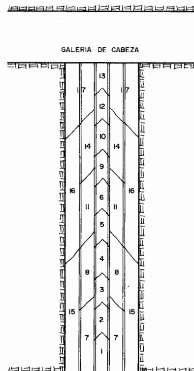
Figura 23.14. Secuencia de avance de una chimenea.
