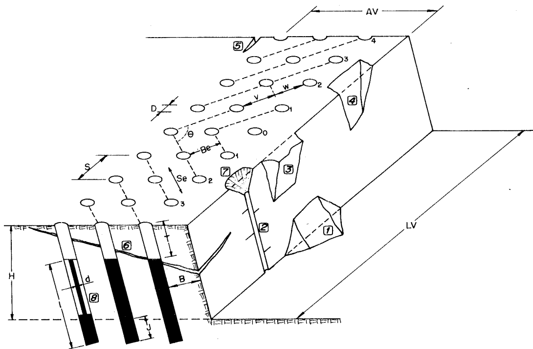
Figura 19.1. Esquema de una voladura en banco.
