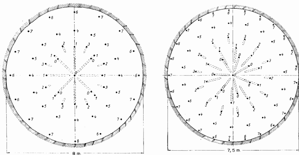
Figura 23.4. Esquemas de perforación con cueles cónicos.
