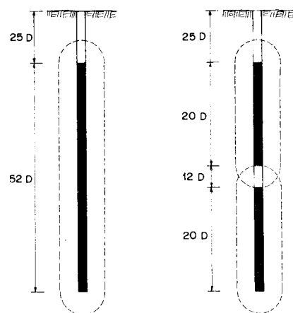
Figura 19.19. Columnas de cargas continuas y espaciadas.
