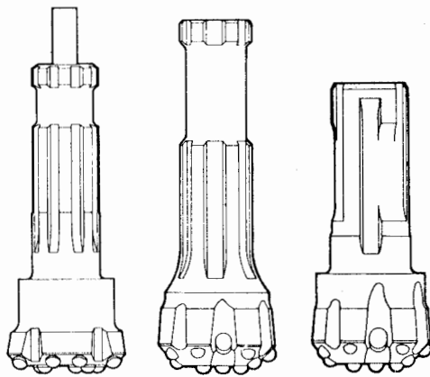
Figura 3.13. Bocas de martillo en fondo.
