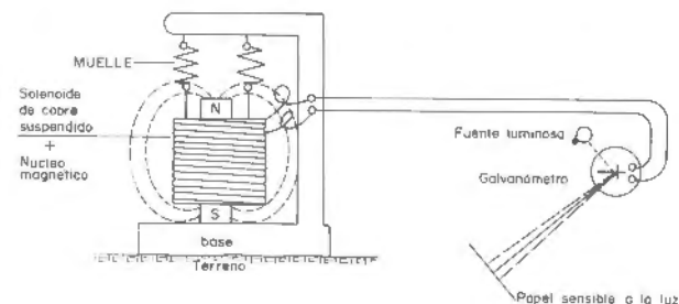
Figura 33.16. Esquema de captador de velocidad.
