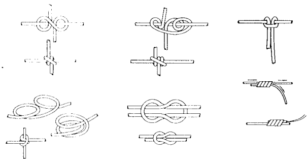
Figura 13.11. Empalmes con cordón detonante.
