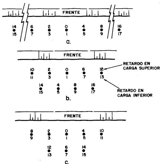
Figura 33.47. Voladuras con cargas seccionadas dentro de los barrenos.
