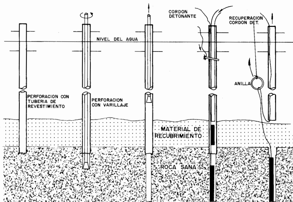
Figura 26.5. Carga de los barrenos.
