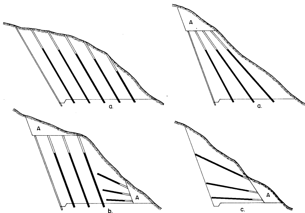
Figura 21.2. Tipos de excavaciones a media ladera.
