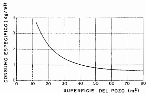
Figura 23.6. Consumo específico de explosivo en función de la sección de los pozos.
