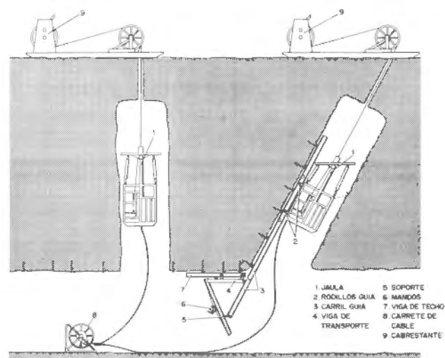
Figura 7.10. Jaula Jora en chimenea vertical e inclinada (Atlas Copco).
