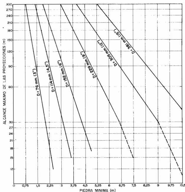
Figura 34.5. Alcances máximos de proyecciones procedentes de frentes verticales en bancos de granito con explosivos tipo ANFO.
