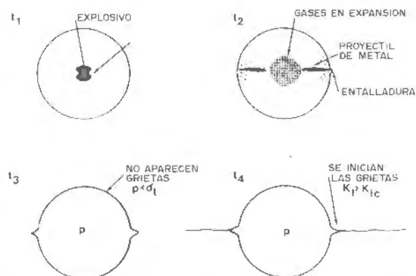
Figura 25.24. Fases de actuación de las cargas de acoplamiento lineal (Bjarnholt y otros).
