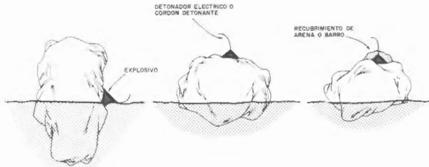
Figura 29.2. Taqueo con cargas superficiales.
