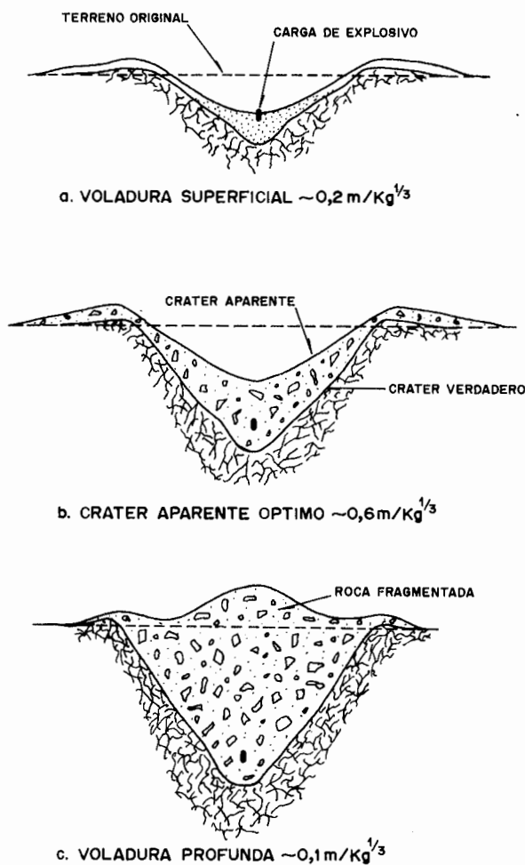
Figura 24.2. Efecto de la profundidad de la carga sobre la geometría del cráter.
