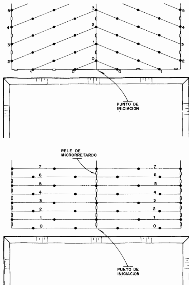
Figura 21.6. Esquemas triangulares con secuencia de encendido en «V» y en línea.
