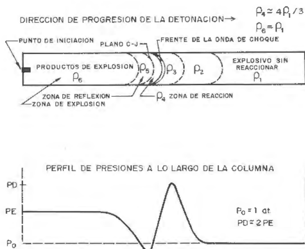
Foto 9.1. Detonación de una carga sin confinar (Nitro-Nobel).
