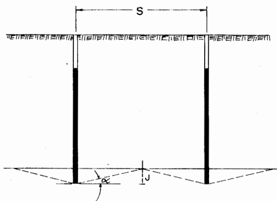
Figura 19.9. Sobreperforación mínima necesaria.
