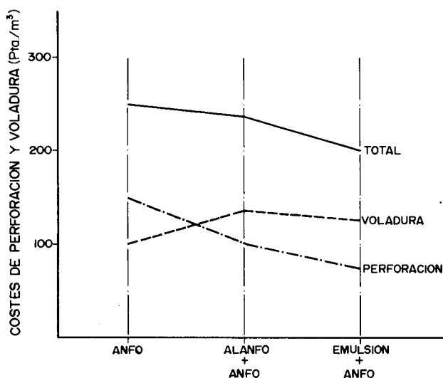
Figura 12.2. Costes relativos de perforación y voladura en rocas duras para distintas alternativas de carga.
