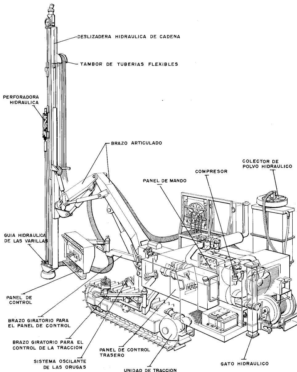
Figura 2.34. Carro hidráulico (Atlas Copco).
