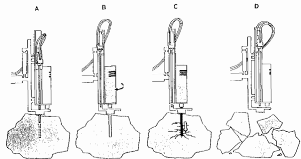
Figura 29.4. Cañón de agua Crac 200 (Atlas Copco).
