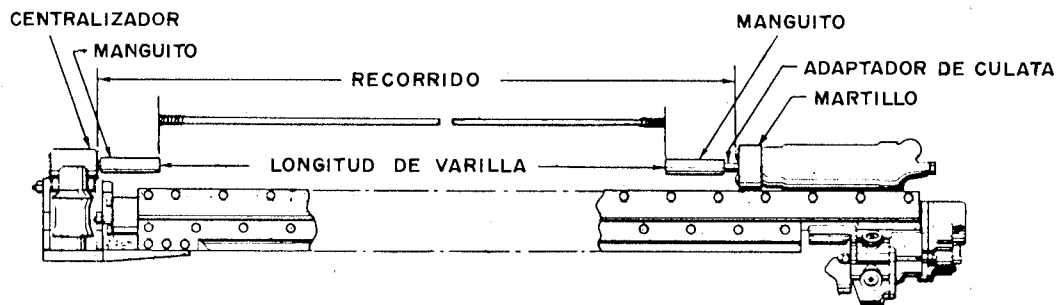
Figura 2.17. Deslizadera de tornillo (Padley & Venables).
