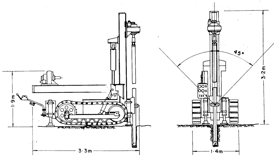
Figura 2.27. Equipo subterráneo de perforación con martillo en fondo (Ingersoll Rand).
