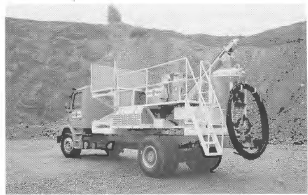
Foto 15.2. Cargadora de ANFO sobre vehículo (Nitro-Nobel).
