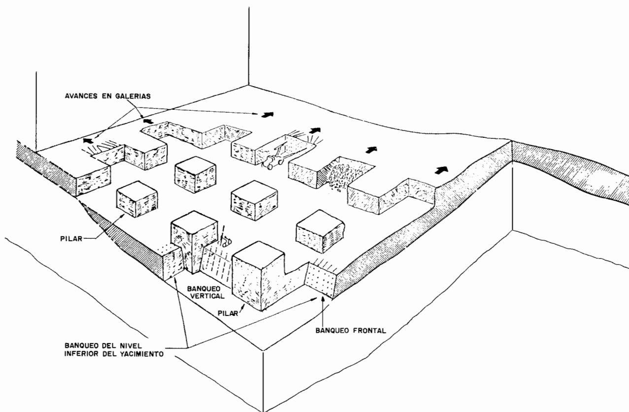
Figura 24.17. Método de explotación por cámaras y pilares.
