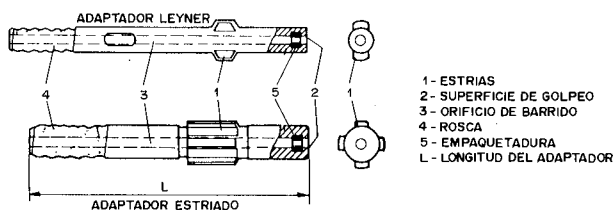
Figura 3.3. Adaptadores de culata (Tamrock).
