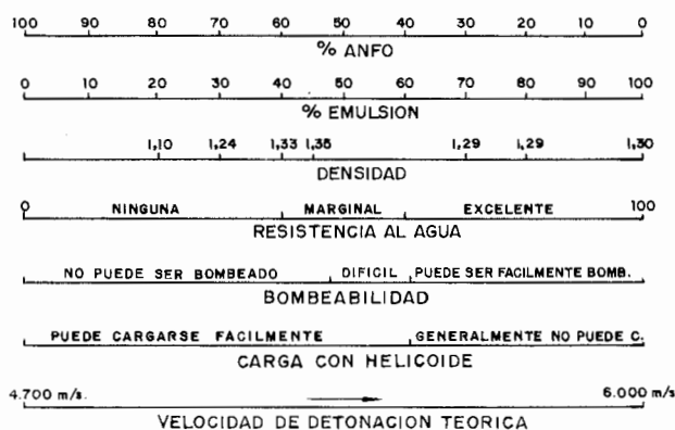
Figura 11.16. Características de carga y resistencia al agua de diferentes tipos de ANFO Pesado (Du Pont, 1986).
