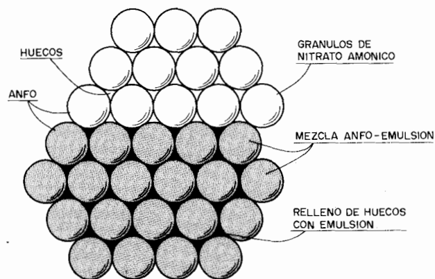
Figura 11.15. Estructura del ANFO Pesado.
