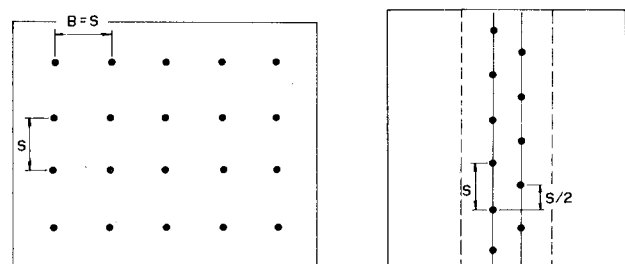
Figura 31.5. Esquemas de perforación de losas.
