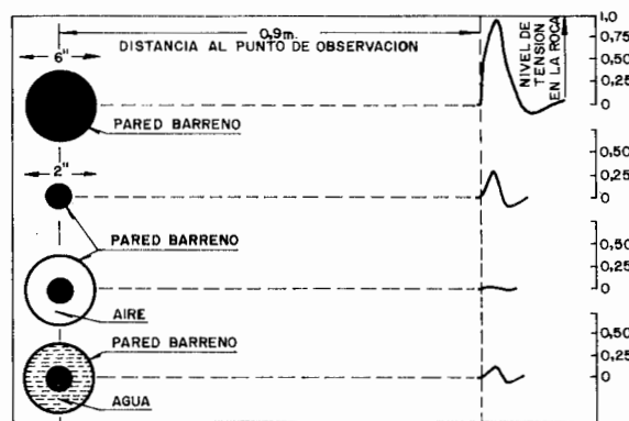
Figura 25.14. Tensiones dinámicas en la roca para distintas condiciones de carga (Day y Webster).
