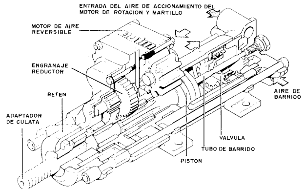
Figura 2.7. Vista seccionada de una perforadora neumática con mecanismo de rotación independiente (Compair-Holman).
