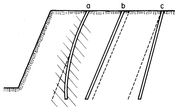
Figura 19.28. Desviaciones de los barrenos y errores en la perforación.
