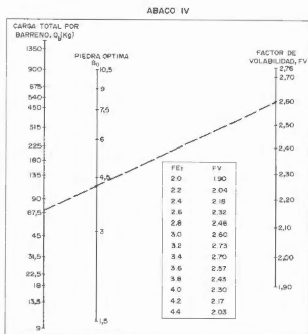
Figura 20.8 Abaco IV.
