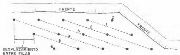
Figura 27.9. Desfase relativo entre filas.
