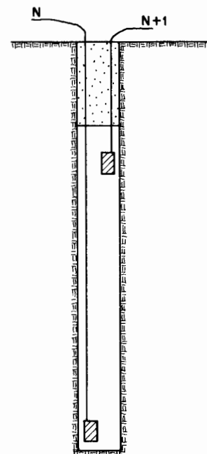
Figura 14.11. Esquema de seguridad con cebado en fondo.
