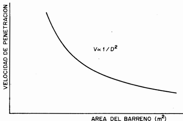
Figura 4.19. Variación de la velocidad de penetración con el diámetro.
