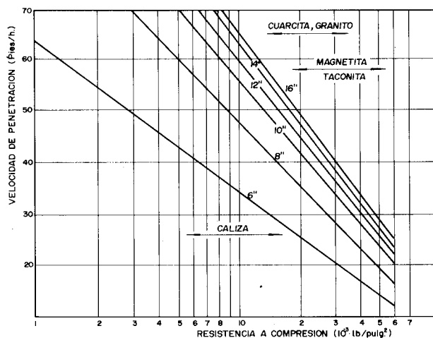
Figura 4.24. Estimación de la Velocidad de Penetración a partir de la Resistencia a Compresión (Bauer y Calder).
