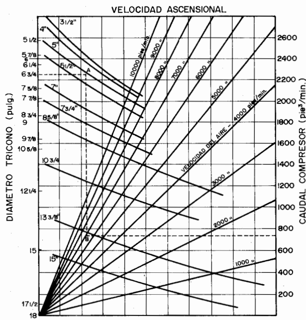
Figura 4.8. Dimensionamiento de las barras.
