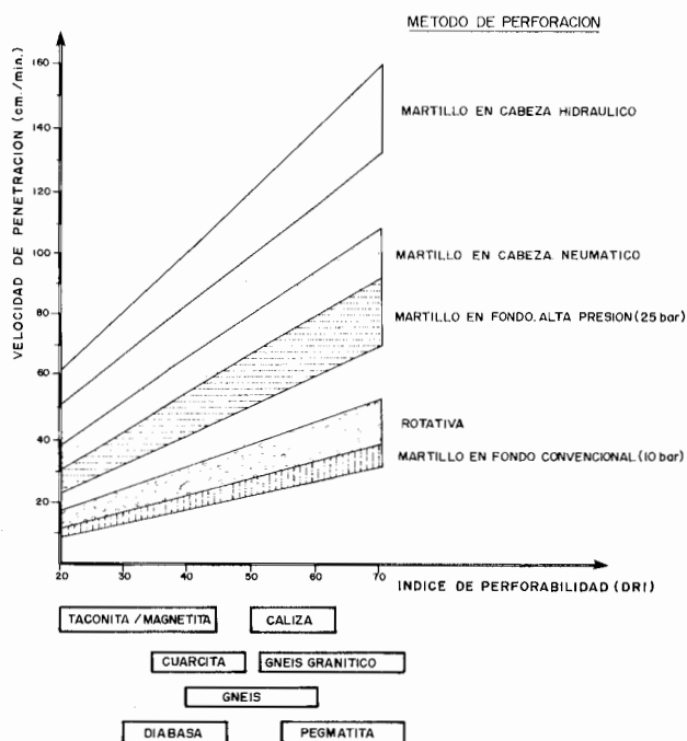
Figura 2.44. Velocidades de penetración obtenidas en diferentes condiciones de trabajo.
