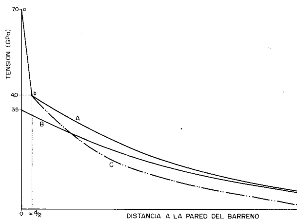
Figura 16.1. Variación de la tensión de pico con la distancia al eje del barreno (Hagan).
