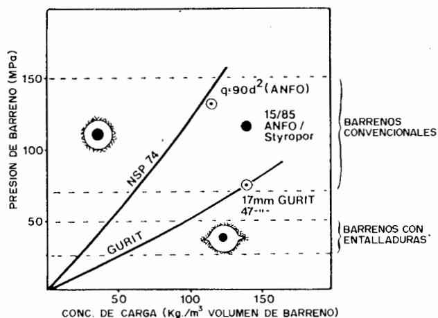
Figura 25.25. Mejora del rendimiento de las cargas de los barrenos con entalladura (Bjarnholt y otros).
