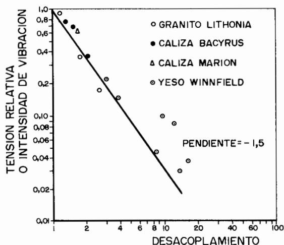
Figura 33.10. Influencia del desacoplamiento en la intensidad de las vibraciones.
