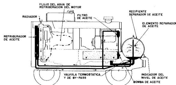
Figura 8.2. Compresor portátil (Ingersoll-Rand).
