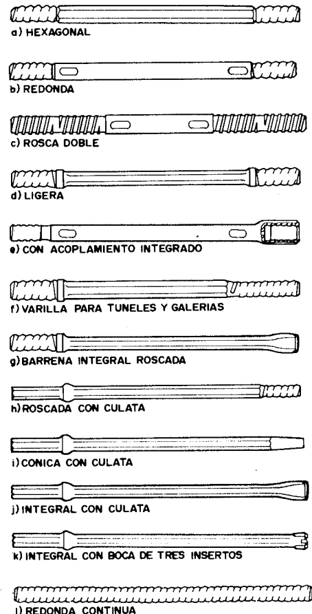
Figura 3.6. Tipos de varillas.
