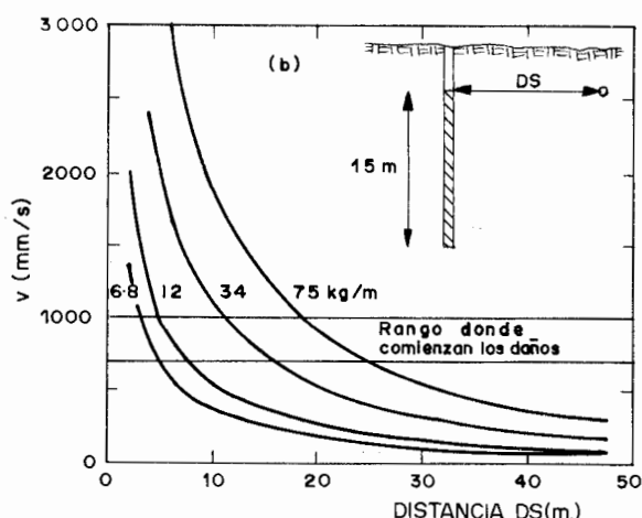
Figura 33.22. Barrenos de gran diámetro y longitud cargados con ANFO (Holmberg y Persson).
