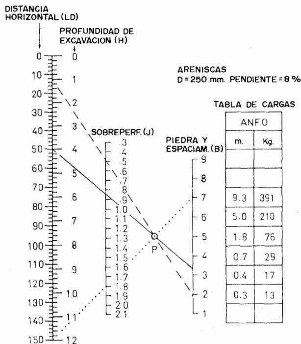
Figura 21.12. Abaco de cálculo (Chung).
