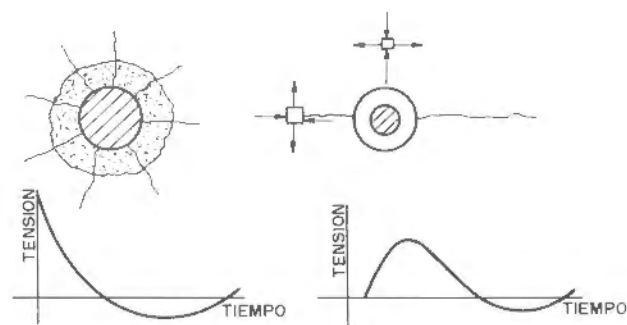
Figura 25.10. Efecto del desacoplamiento sobre la curva tensión-tiempo.
