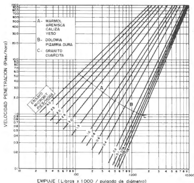
Figura 4.23. Determinación de la velocidad de penetración a partir de ensayos Microbit.
