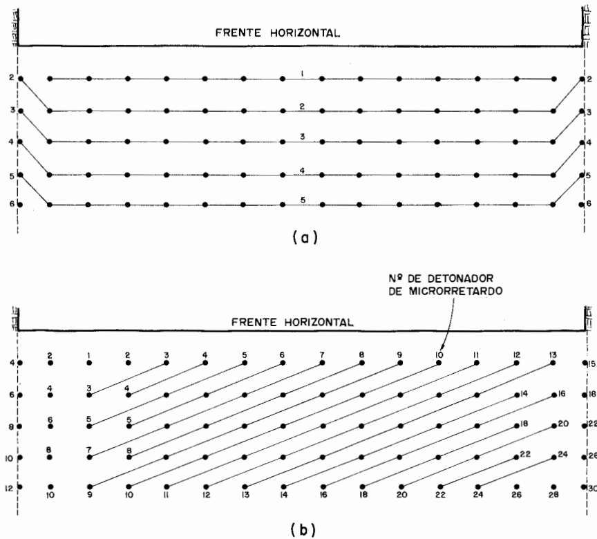
Figura 27.11. Voladuras en banco horizontal (a) sobreexcavación importante (b) sobreexcavación pequeña.
