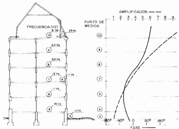
Figura 33.33. Factores de amplificación de un edificio (Clark et al.).
