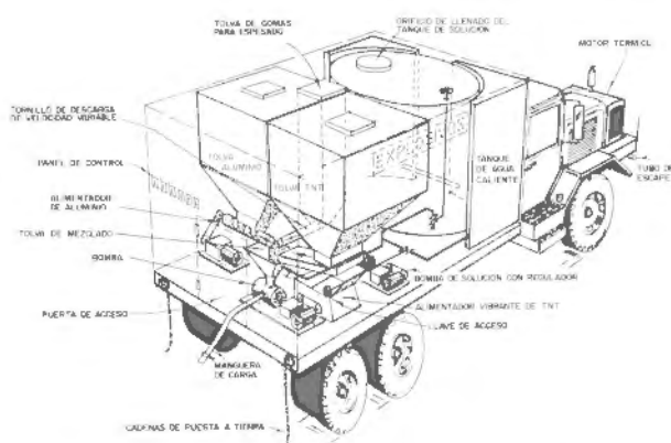
Figura 15.8. Camión mezclador-cargador (Ireco Inc.).
