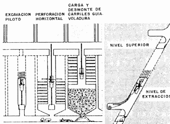
Figura 7.9. Método de explotación de yacimientos estrechos e inclinados.
