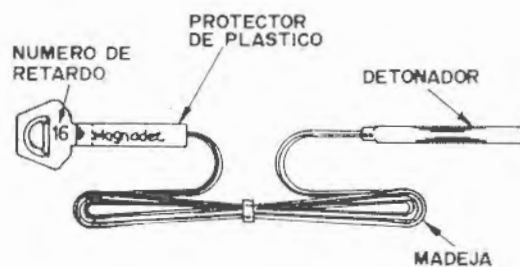
Figura 13.17. Detonador Magnadet.
