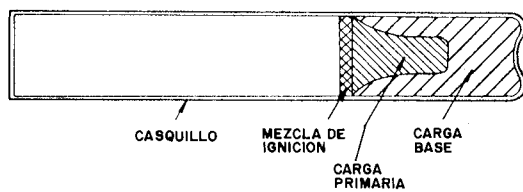
Figura 13.8. Detonador ordinario.
