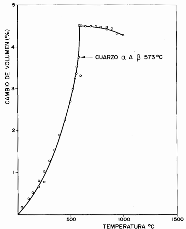
Figura 7.13. Dilatación térmica volumétrica del cuarzo (Dane, 1942).
