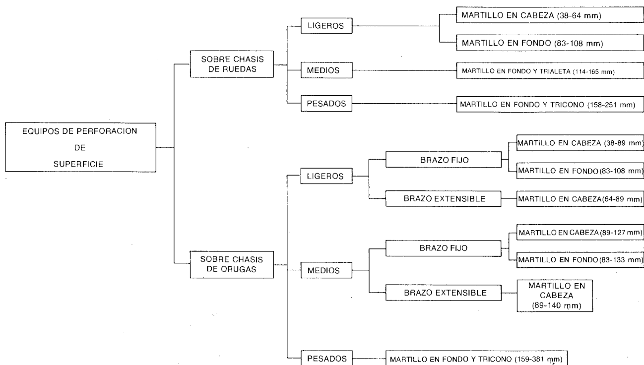
Figura 2.28. Sistemas de montaje de perforadoras de superficie.
