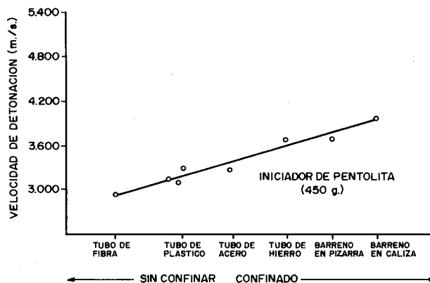
Figura 11.8. Variación de la velocidad de detonación con el confinamiento.
