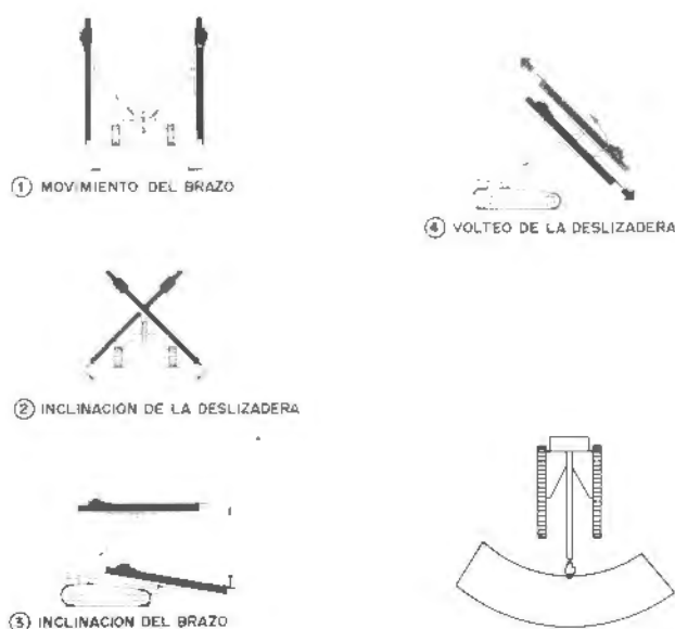
Figura 2.32. Movimientos del brazo y deslizadera.
