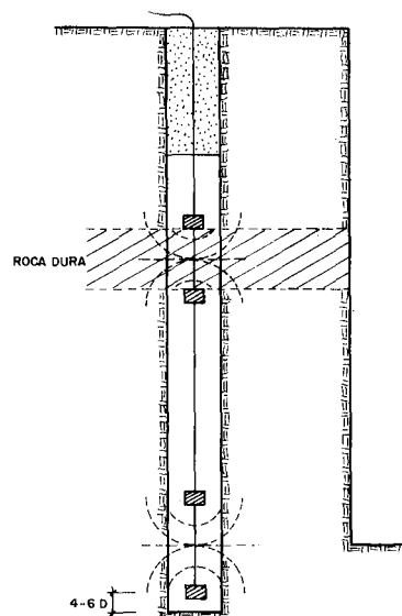
Figura 14.13. Aplicaciones del cebado múltiple a una voladura en banco.
