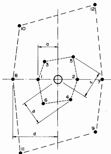
Figura 22.12. Cuele y contracuele de doble espiral.
