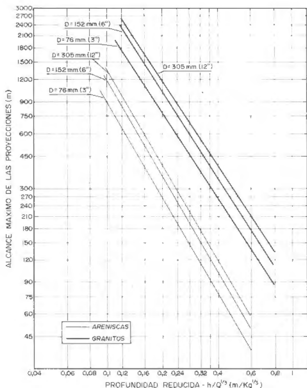
Figura 34.6. Alcances máximos de proyecciones procedentes de las superficies de los bancos de granitos y areniscas con explosivos tipo ANFO.
