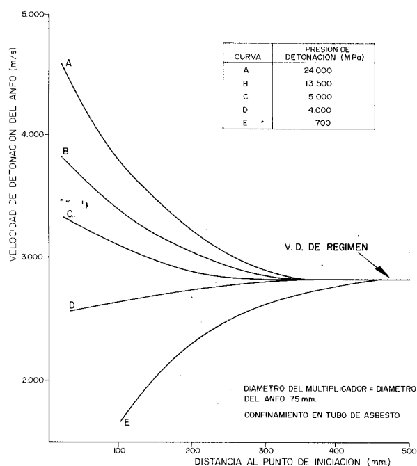
Figura 14.1. Efecto de la presión de detonación del iniciador sobre la velocidad inicial del ANFO (Junk, 1972).
