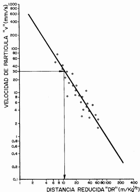
Figura 33.30. Ley de propagación ajustada.
