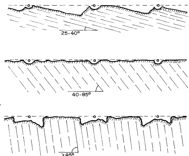
Figura 25.8. Influencia de los ángulos formados por la estratificación sobre las leyes de propagación de las vibraciones.
