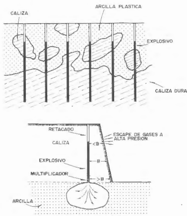
Figura 17.3. Casos típicos de cambios litológicos con contacto entre rocas competentes y materiales plásticos (Hagan).
