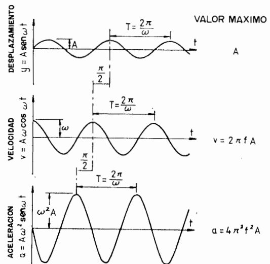
Figura 33.13. Movimiento ondulatorio sinusoidal.
