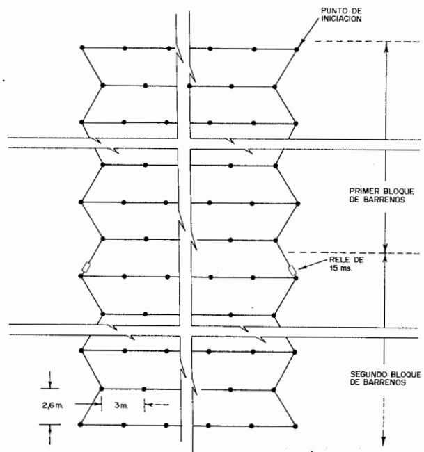
Figura 21.17. Prevoladura disparada con cordón detonante de bajo gramaje y relés de microrretardo.
