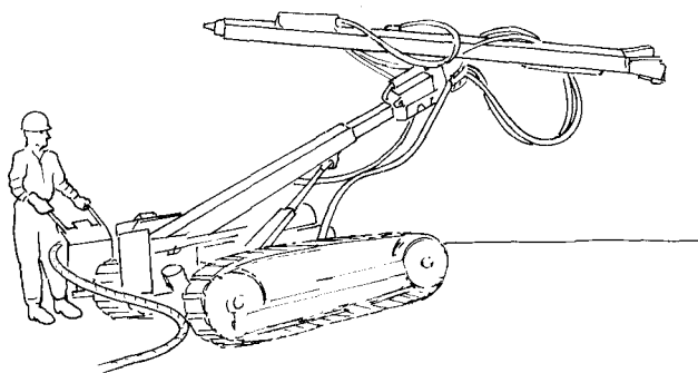
Figura 35.6. Posición de las deslizaderas durante los desplazamientos de las perforadoras.
