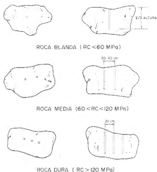
Figura 29.6. Fragmentación de bolas entre 1 y 2 m 3 con cementos expansivos.
