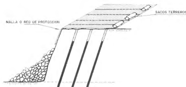
Figura 34.8. Protección de voladura en banco.
