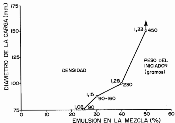
Figura 11.18. Variación de la sensibilidad del ANFO Pesado con el porcentaje de emulsión de la mezcla (Bamptfield y Morrey, 1984).
