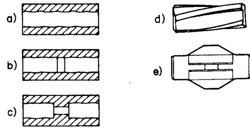
Figura 3.9. Tipos de manguitos.
