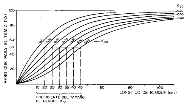
Figura 32.10. Determinación del Coeficiente del Tamaño de Bloque « K_{50} » del material fragmentado.
