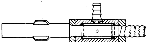
Figura 3.4. Adaptador con barrido lateral.
