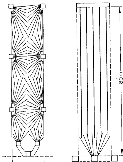
Figura 24.11. Esquemas de perforación en los métodos de Cámaras por Subniveles Convencional y de Barrenos Largos.
