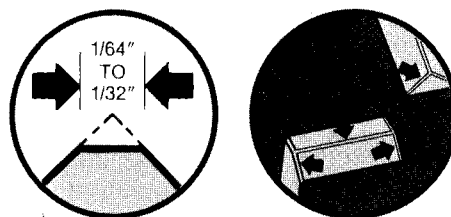
Figura 3.25. Biselado de aristas.
