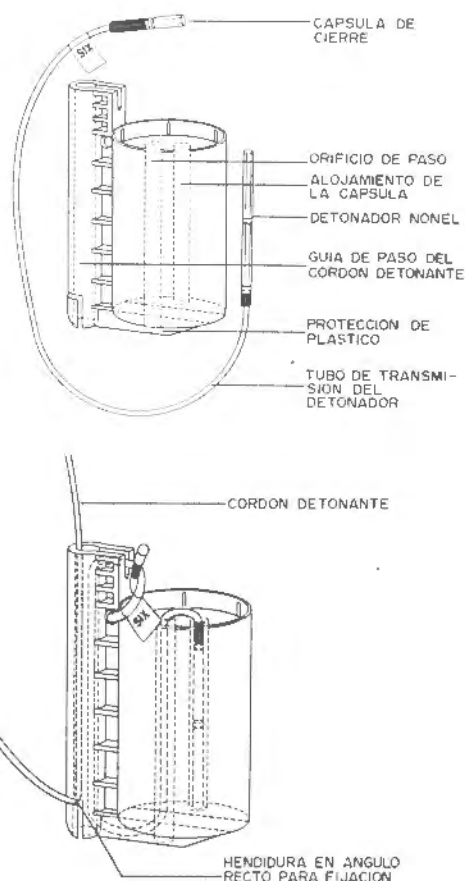
Figura 13.5. Elementos y ensamble de un multiplicador temporizado Slider.
