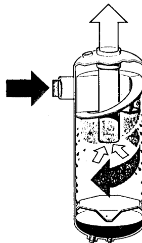
Figura 8.4. Separador de humedad (Atlas Copco).
