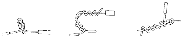
Figura 13.16. Conexiones recomendadas en los circuitos eléctricos.
