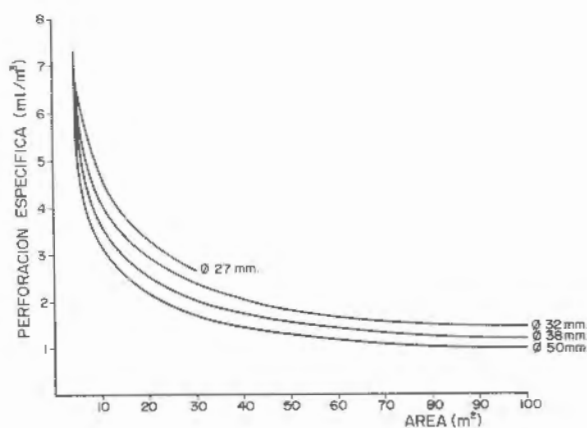
Figura 22.19. Perforación específica en función del área del túnel y diámetro de perforación.
