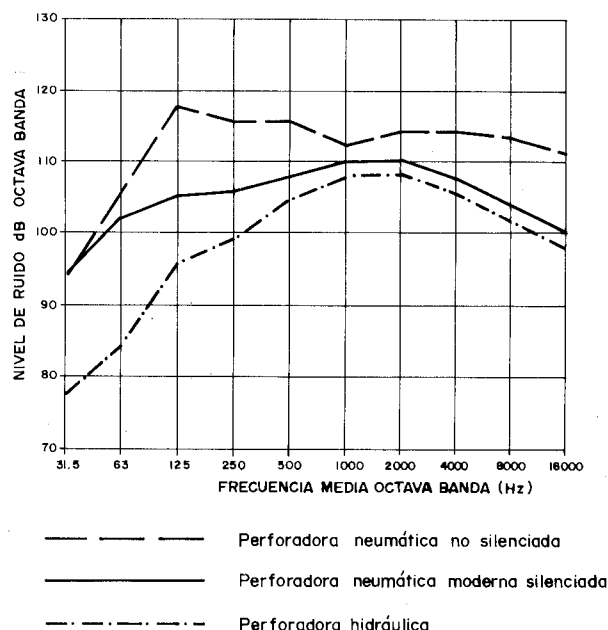
Figura 2.10. Menor nivel de ruido producido por las perforadoras hidráulicas.
