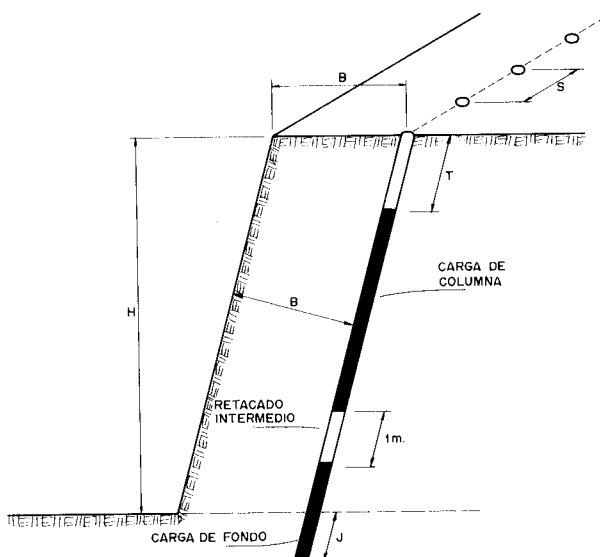
Figura 20.1. Esquema de voladura para producción de escollera.
