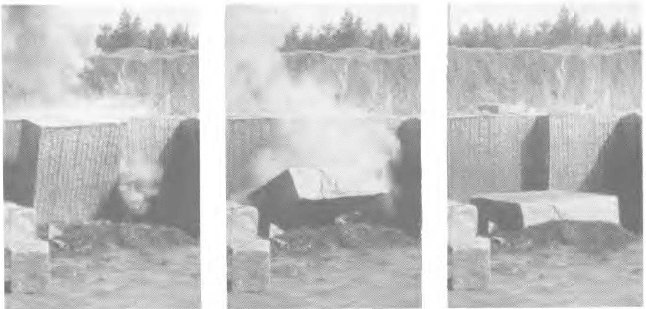
Foto 25.6. Arranque con voladura de un bloque de granito. (Cortesía de OY Forcit AB).
