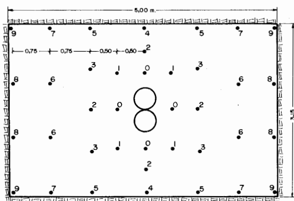
Figura 22.29. Esquema de perforación con cuele cilíndrico constituido por dos barrenos de gran diámetro.
