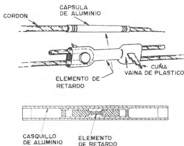
Figura 13.6. Tipos de relés de microrretardo de superficie.
