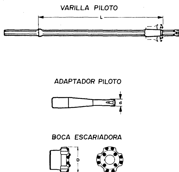
Figura 3.12. Boca de escariar, varilla piloto y adaptador piloto.
