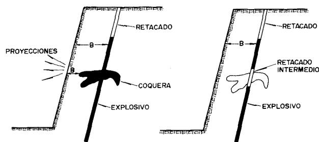
Figura 17.1. Ejecución correcta de la carga de un explosivo a granel en un terreno con coqueras.
