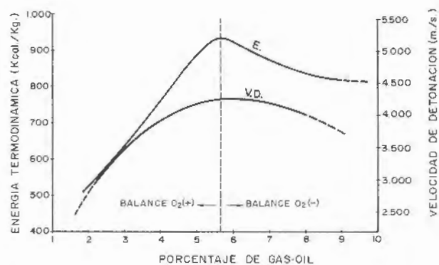
Figura 11.2. Variación de la Energía termodinámica y Velocidad de detonación del ANFO con el contenido de gas-oil.
