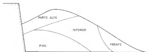
Figura 28.3. Zonas de una pila de escombro.
