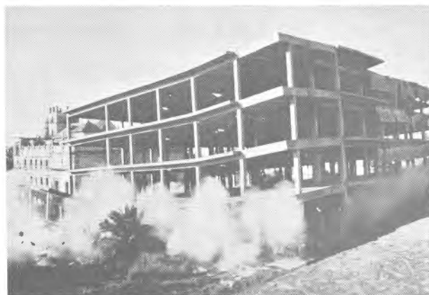
Foto 31.7. Demolición de la estructura de un edificio de hormigón. (Cortesía de CAVOSA).
