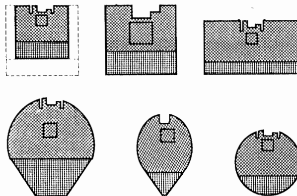
Figura 7.8. Diferentes configuraciones de plataformas.
