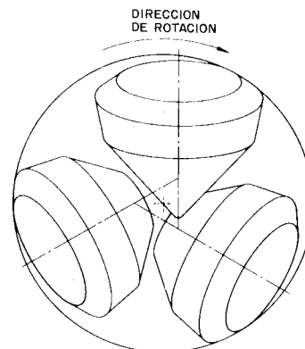
Figura 5.4. Descentramiento (Hughes Tool Co.).
