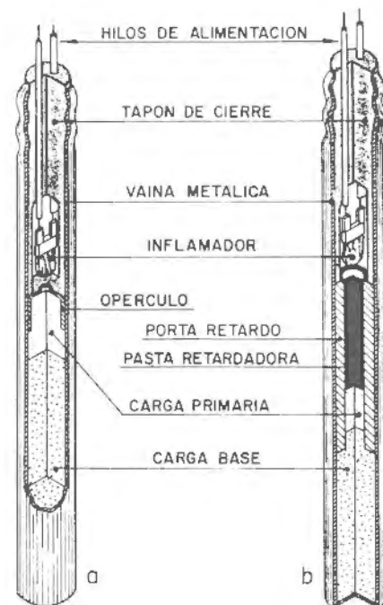
Figura 13.12. Detonadores eléctricos. Instantáneos y Temporizados.
