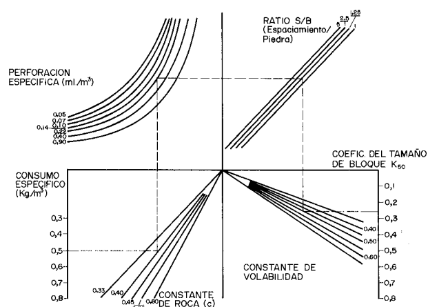
Figura 32.8. Nomograma para la determinación del tamaño de bloque.
