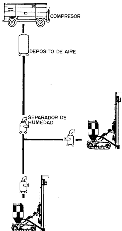
Figura 8.5. Sistema de distribución de aire comprimido.
