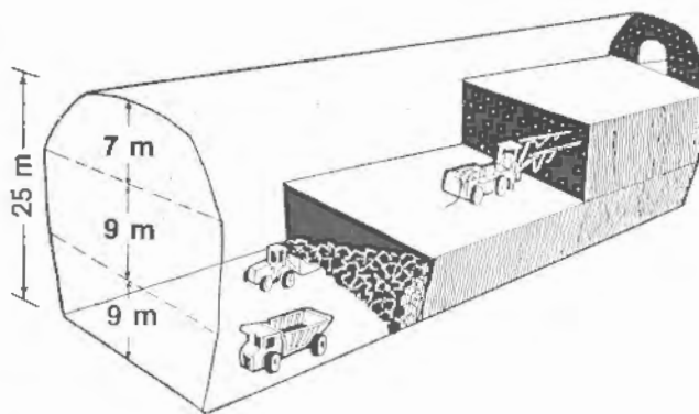
Figura 24.23. Excavación de una cámara con dos bancos y perforación horizontal con jumbo.
