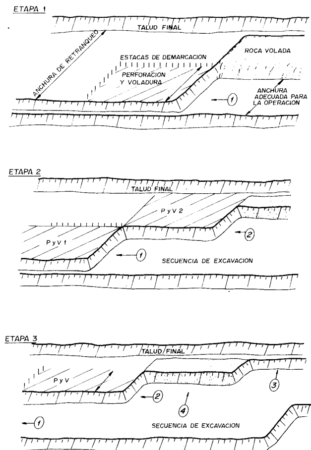
Figura 30.3. Secuencia de avance en las proximidades de un talud final.
