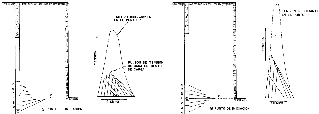
Figura 14.9. Pulsos de tensión registrados en un punto «P» para dos posiciones de cebado en fondo (Hagan, 1974).
