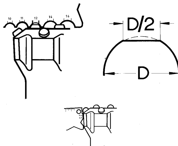
Figura 3.18. Medida del desgaste de botones.
