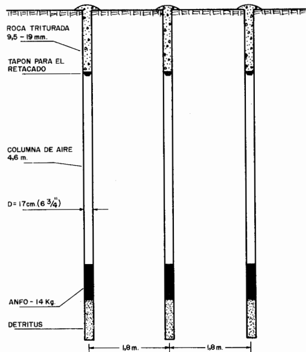
Figura 25.27. Técnica de precorte «ADP» con columnas de aire.
