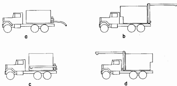
Figura 15.6. Camiones de carga neumática (a) y de tornillo helicoidal (b, c y d).
