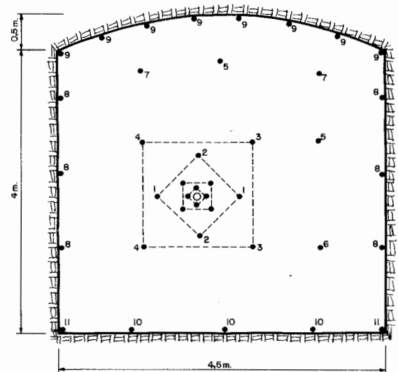
Figura 22.16. Esquema geométrico de la voladura calculada.
