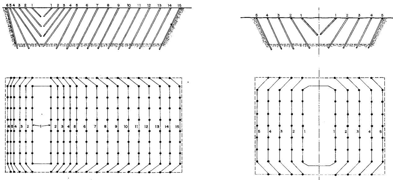
Figura 21.15. Disposición de barrenos en excavaciones alargadas y estrechas.
