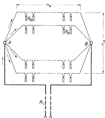
Figura 13.15. Circuito serie-paralelo.
