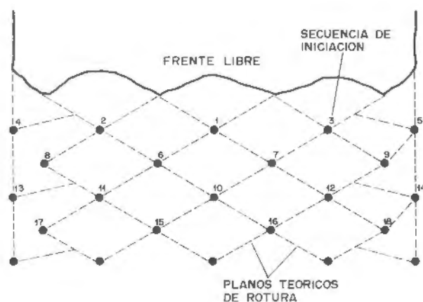
Figura 19.14. Geometría del frente libre y secuencia de encendido.
