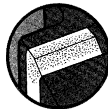
Figura 3.22. Pulido de pastillas.
