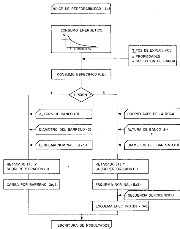
Figura 18.17. Cálculo de esquemas de perforación y cargas de explosivos a partir del I_p (L. Jimeno).
