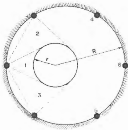
Figura 23.19. Disparo de voladura con hueco central de gran diámetro.
