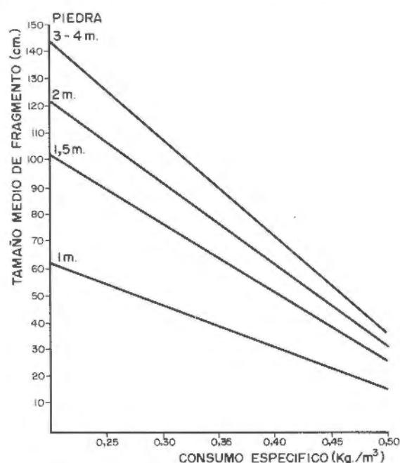
Figura 32.11. Tamaños medios de fragmentos en función de la piedra y el consumo específico de explosivo.
