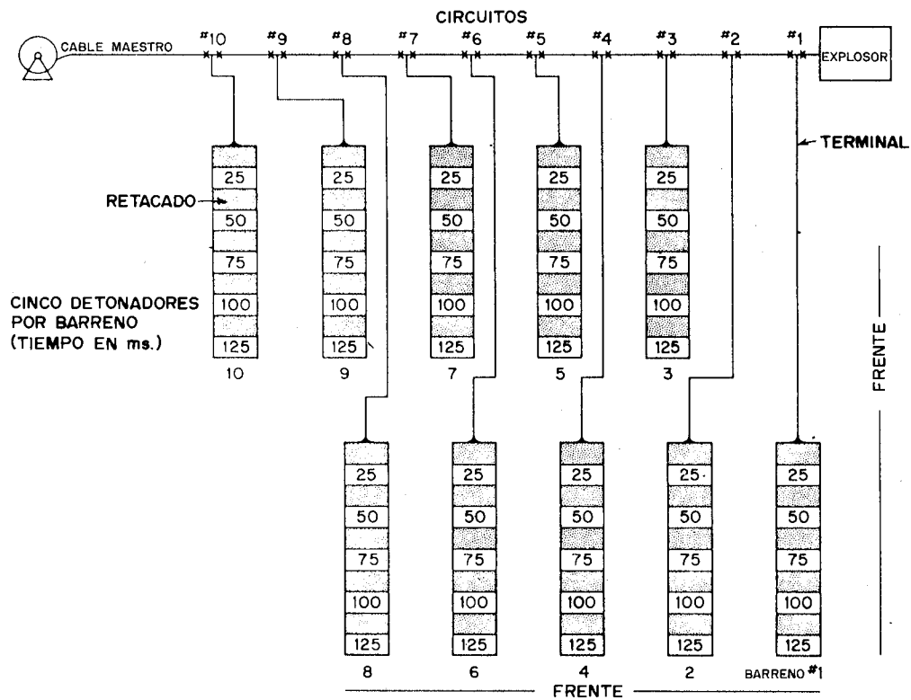
Figura 13.20. Voladura múltiple con cargas secuenciadas dentro de los barrenos.
