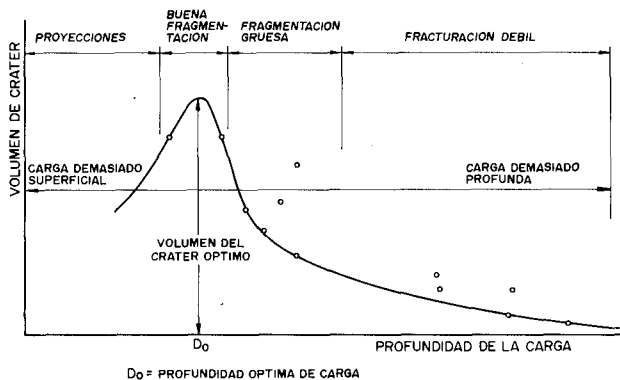
Figura 24.5. Representación de los resultados de voladuras en cráter.
