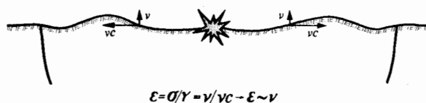
Figura 25.18. Relación entre deformaciones «ε», tensiones «σ», velocidades de partícula «v» y velocidad de propagación de las ondas «VC» (Holmberg y otros).
