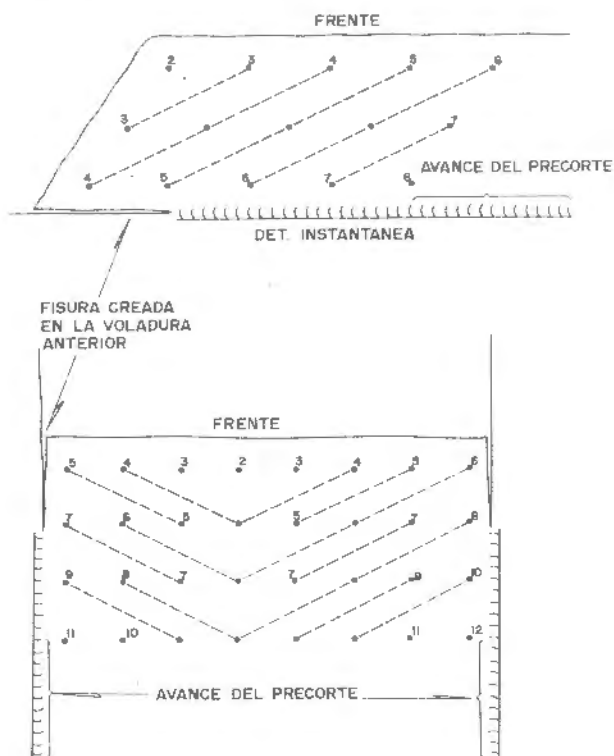
Figura 25.21. Avance de las voladuras de precorte.
