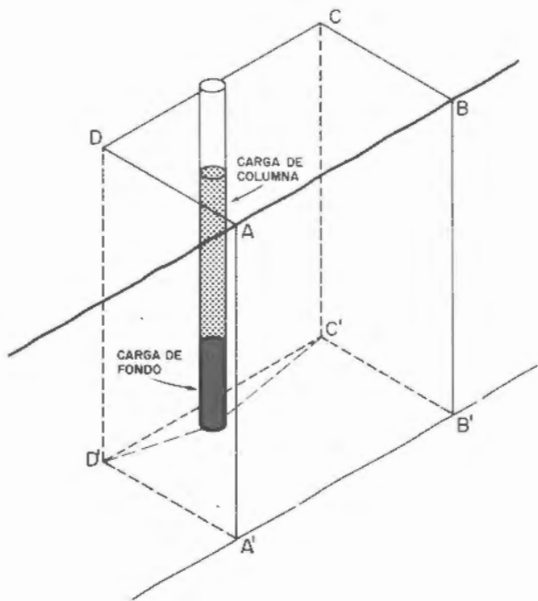
Figura 19.23. Distribución del explosivo en un barreno para fragmentar la roca en una voladura en banco.
