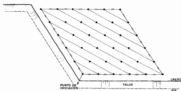
Figura 20.4. Secuencia de encendido «V1» para un esquema cuadrado al tresbolillo.
