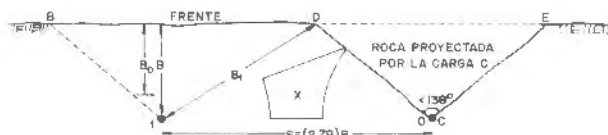
Figura 27.5. Voladura de microrretardo con piedra y espaciamiento mayores que el óptimo (Hagan, 1975).
