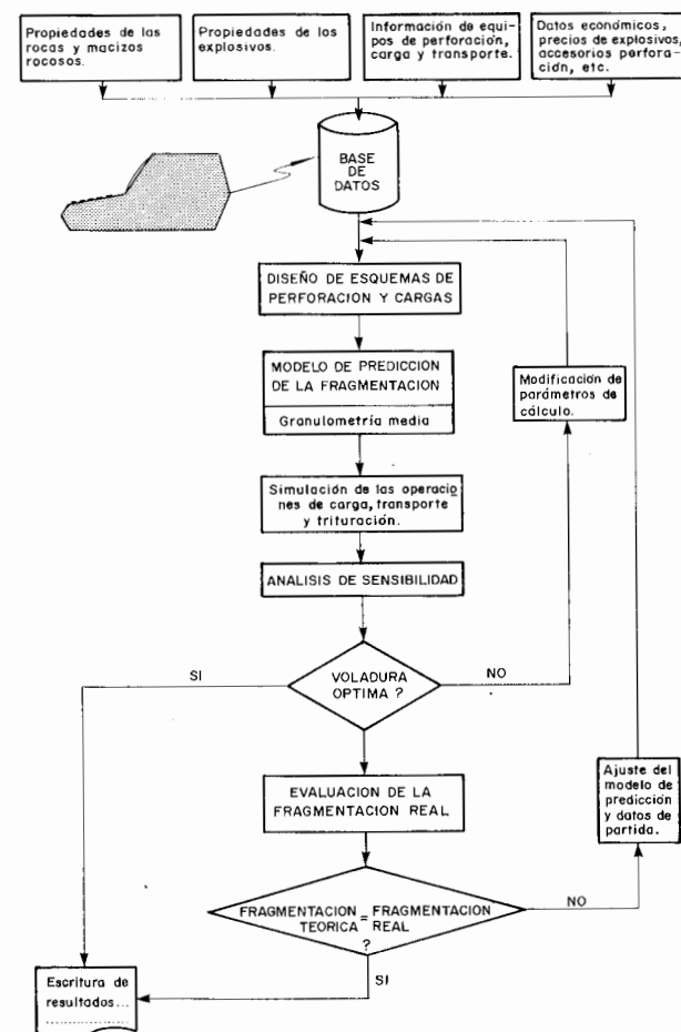
Figura 32.6. Estructura básica del modelo de optimización de costes.
