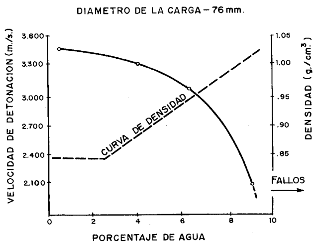
Figura 11.6. Influencia del contenido de agua sobre la velocidad de detonación.
