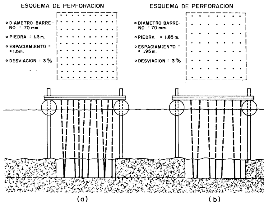
Figura 26.4. Carga manual (a). Carga mecanizada (b).
