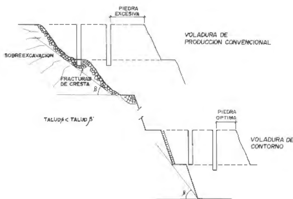
Figura 25.1. Daños provocados en el talud por las voladuras de producción y aplicación de las voladuras de contorno.
