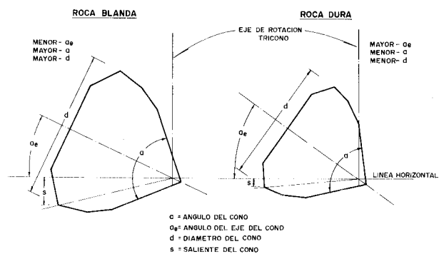
Figura 5.3. Angulos del eje del cono en dos tipos de roca.
