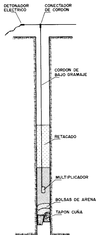
Figura 24.8. Disposición de la carga dentro de un barreno.
