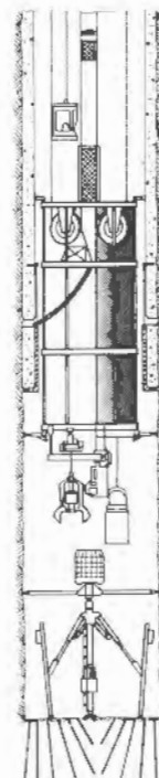
Figura 7.6. Equipo completo de excavación de pozos.
