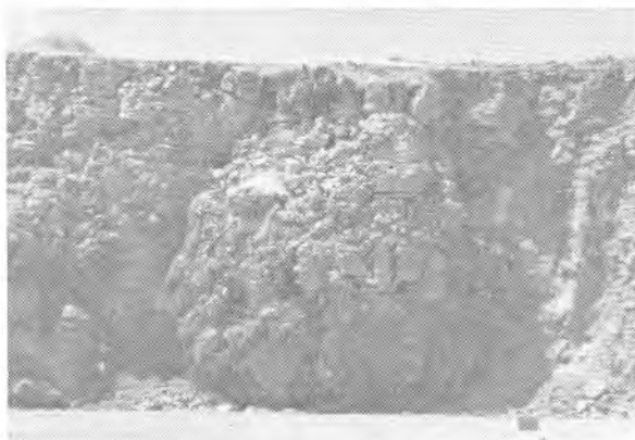
Foto 33.8. Desplazamiento del frente en una voladura de un solo barreno de una campaña vibrográfica.
