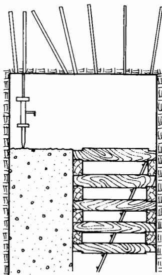
Figura 23.10. Excavación manual de chimeneas.
