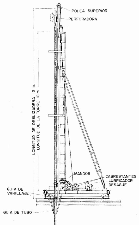
Figura 26.2. Mástil de perforadora (Atlas Copco).
