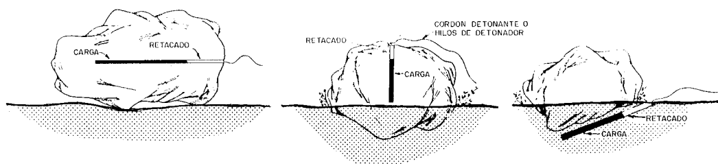
Figura 29.1. Taqueo de bloques con perforación de barrenos.
