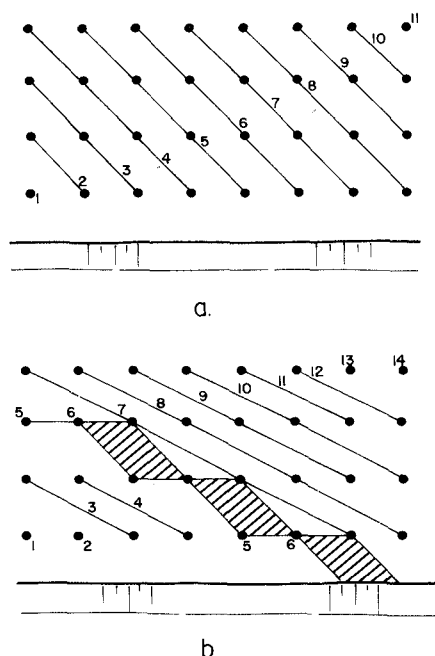
Figura 27.16. Comparación de dos esquemas de voladura múltiple con distintas secuencias de encendido.
