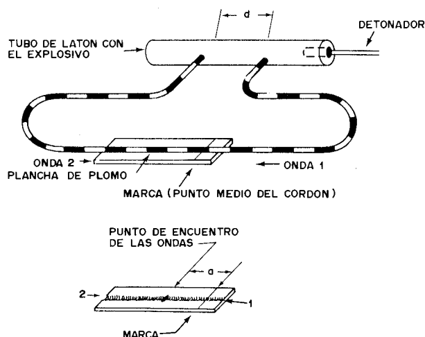
Figura 10.6. Método D'Autriche.
