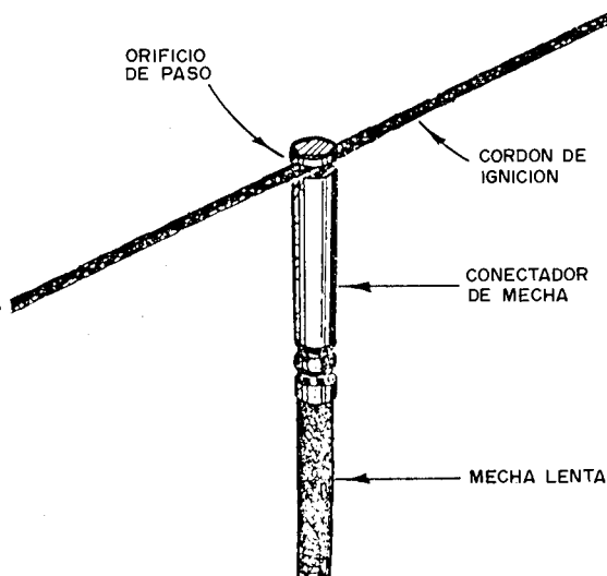
Figura 13.10. Sistema de encendido rápido de mecha de seguridad.
