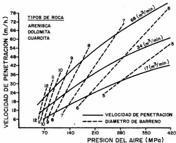
Figura 7.15. Velocidades de penetración con quemadores de aire comprimido.
