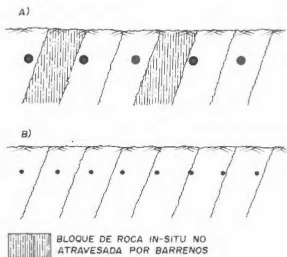
Figura 19.2. Influencia del esquema de perforación y de las discontinuidades en la producción de grandes bloques.
