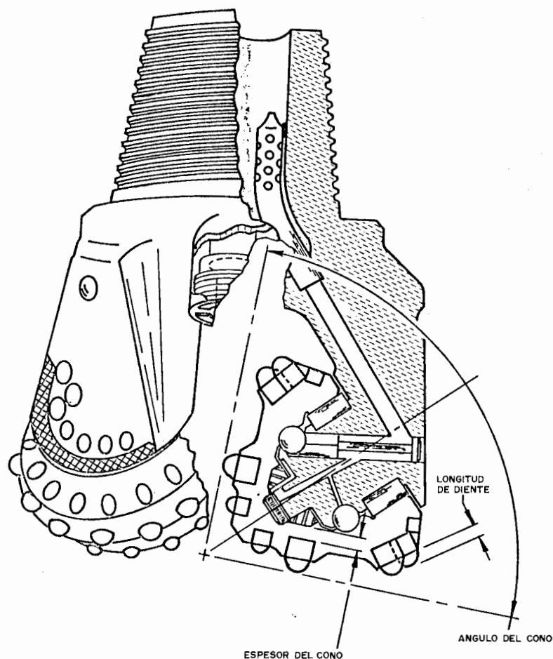
Figura 5.5. Angulo del cono, longitud de diente y espesor del cono (Smith-Gruner).
