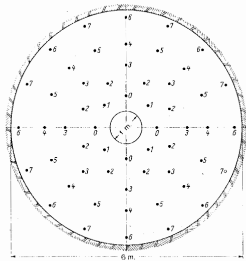
Figura 23.8. Voladura con chimenea central.
