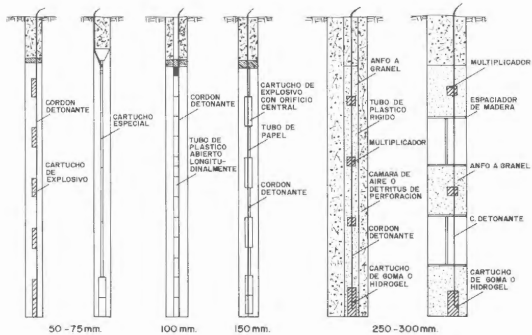
Figura 25.11. Diversos diseños de carga en barrenos de contorno en función del diámetro.
