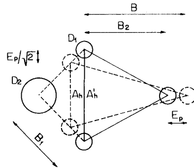
Figura 22.9. Influencia en la desviación de los barrenos.
