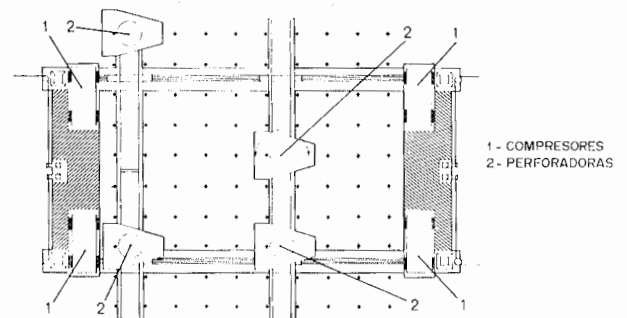
Figura 26.3. Croquis de plataforma autoelevable con bastidor móvil (Atlas Copco).
