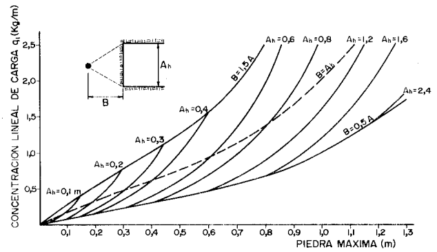
Figura 22.8. Relación entre la concentración lineal de carga y la piedra máxima para diferentes anchuras de hueco (Larsson y Clark).
