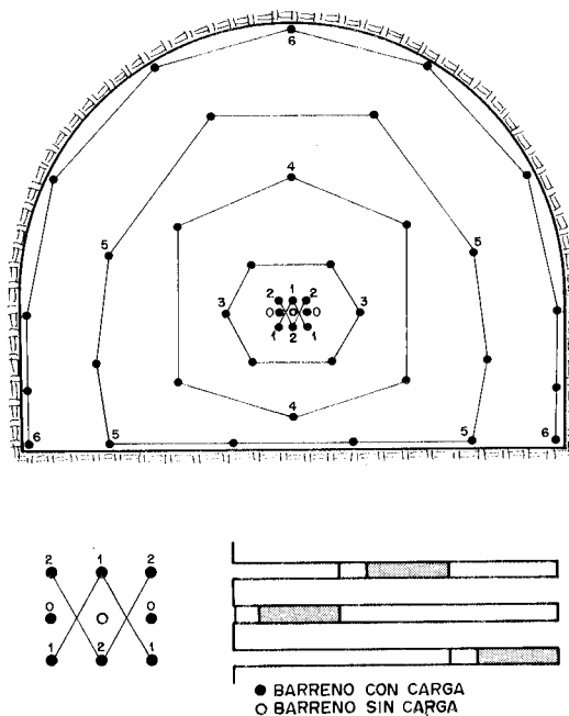
Figura 22.21. Voladura de galería con cuele Sarrois.
