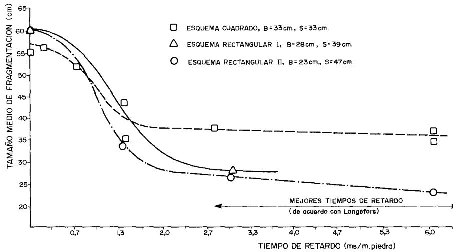
Figura 27.13. Efecto del tiempo de retardo entre barrenos sobre la fragmentación media, para un mismo consumo específico (Bergmann, 1975).
