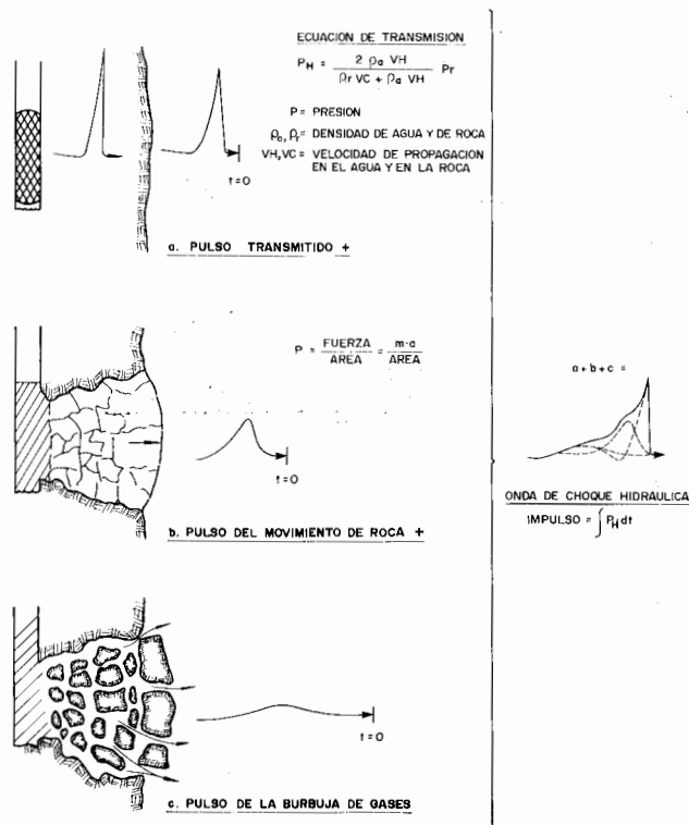
Figura 26.6. Modelo de formación de una onda de choque hidráulica.
