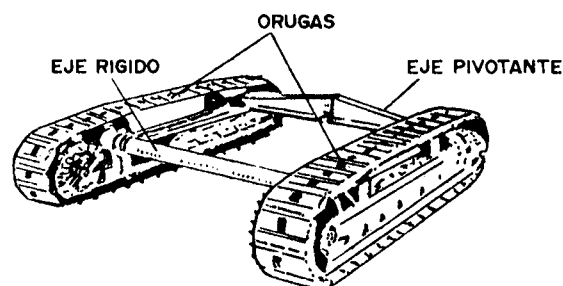
Figura 4.2. Diseño del tren de orugas.
