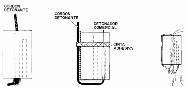
Figura 14.3. Multiplicadores convencionales.
