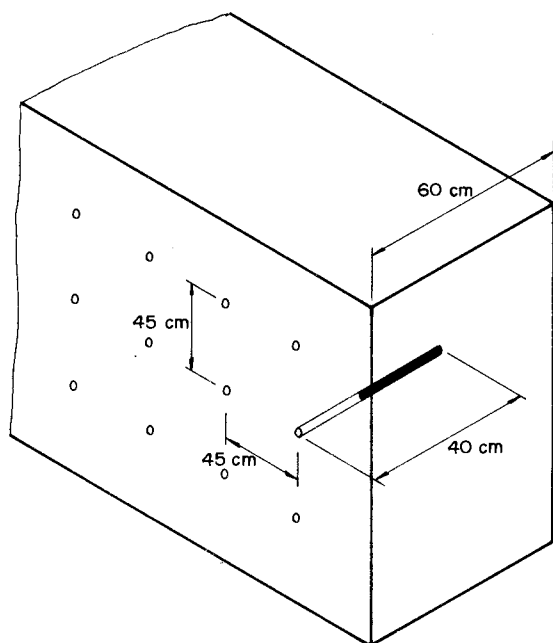
Figura 31.2. Disposición de barrenos en un muro de hormigón.
