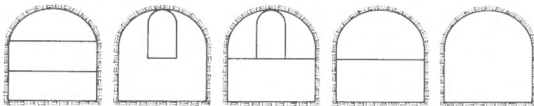
Figura 22.1. Sistemas de avance en la excavación de túneles y galerías.
