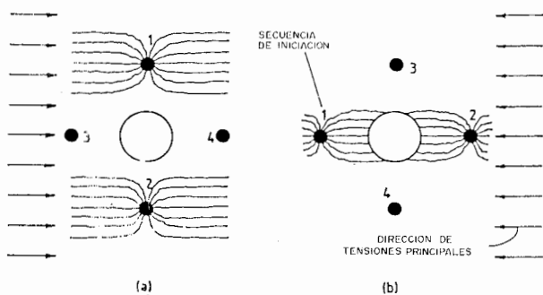
Figura 17.7. Secuencia de iniciación en un cuele con barreno central de diámetro y tensiones residuales horizontales (a) Secuencia incorrecta (b) Secuencia correcta.
