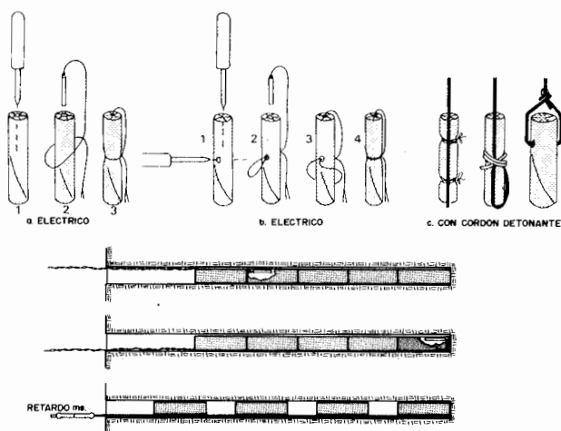
Figura 14.15. Cebado de cartuchos y barrenos.
