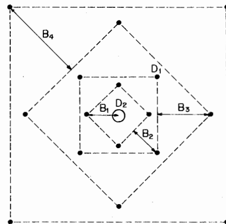
Figura 22.5. Cuele de cuatro secciones.
