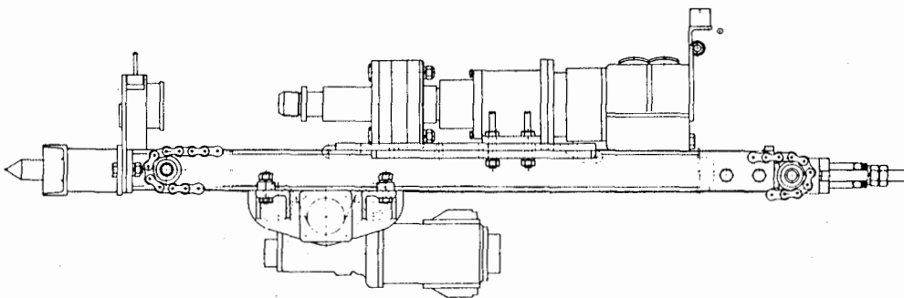
Figura 2.16. Deslizadera de cadena (Padley & Venables).
