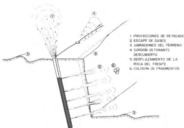
Figura 33.14. Fuentes de onda aérea en las voladuras.
