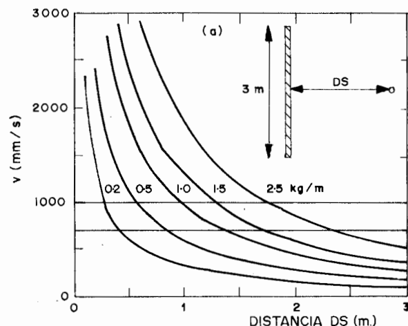
Figura 33.21. Barrenos de pequeño diámetro y longitud cargados con ANFO (Holmberg y Persson).
