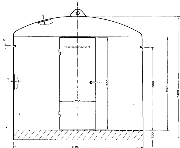
Figura 34.10. Campana de seguridad para protección del artillero.
