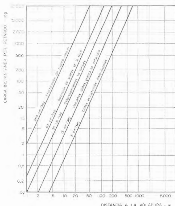
Figura 33.42. Variación de la velocidad de partícula máxima y daños previsibles con la distancia y carga por retardo (Lan-gefors y Kihiström).
