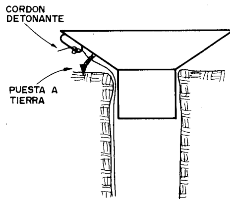
Figura 13.26. Embudo para la carga de explosivos a granel.
