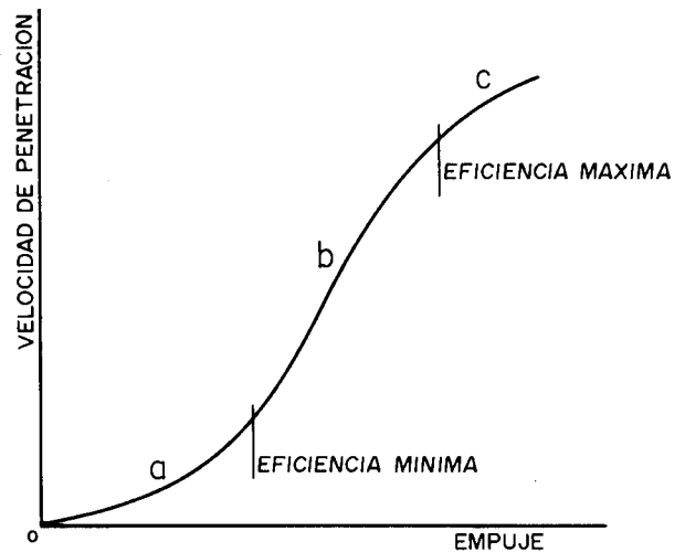
Figura 4.16. Efecto del empuje sobre la velocidad de penetración.
