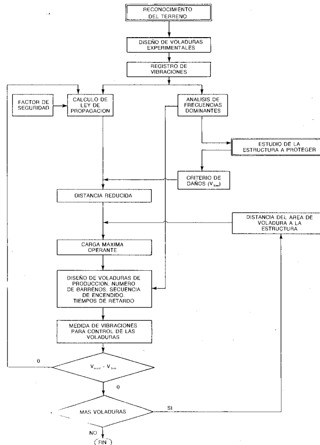
Figura 33.28. Organigrama de ejecución de una campaña vibrográfica.
