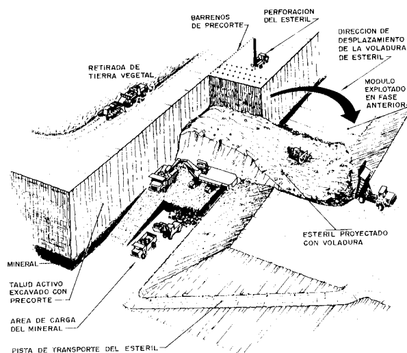
Figura 20.2. Método de explotación con voladuras de máximo desplazamiento.
