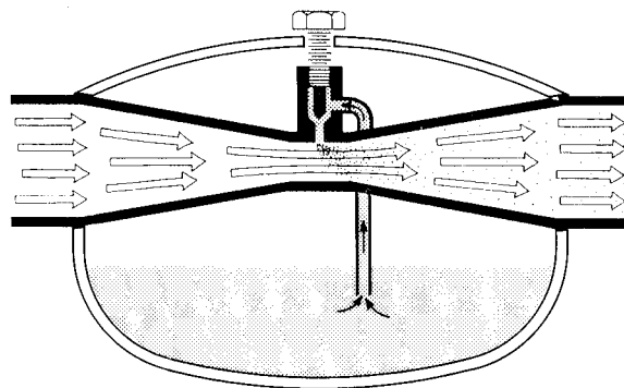
Figura 8.6. Sección de un engrasador.
