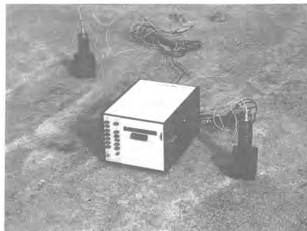
Foto 33.4. Captadores de velocidad de partícula y registrador continuo de papel fotográfico.
