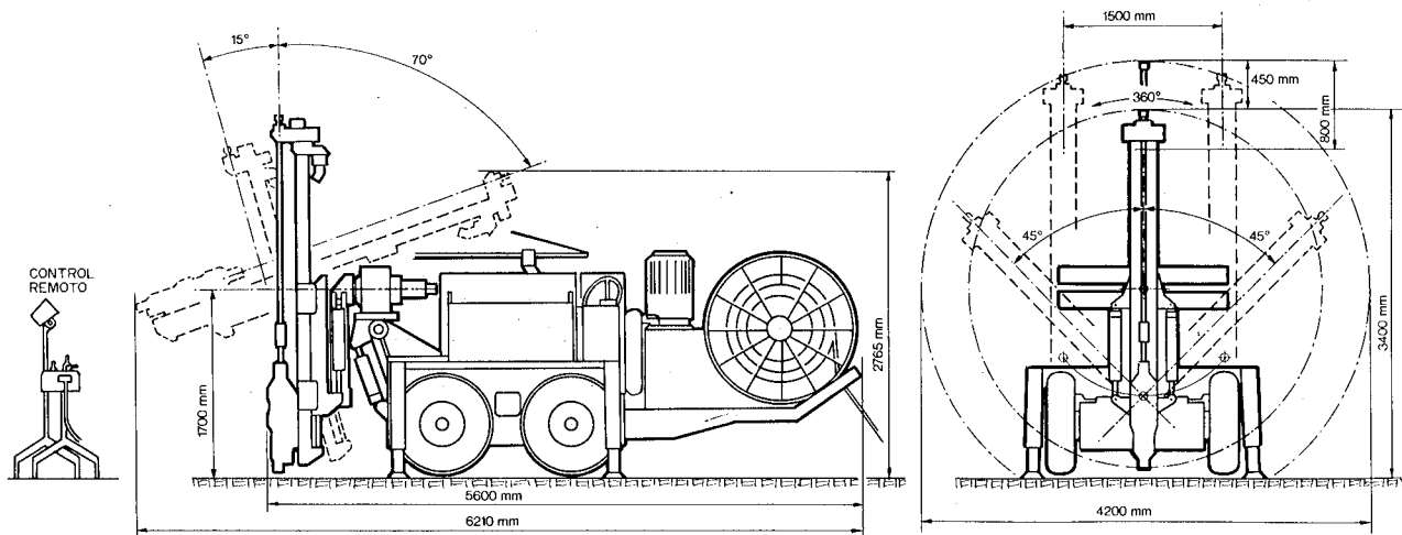
Figura 2.26. Equipo de perforación de barrenos largos montado sobre chasis de neumáticos (Atlas Copco).
