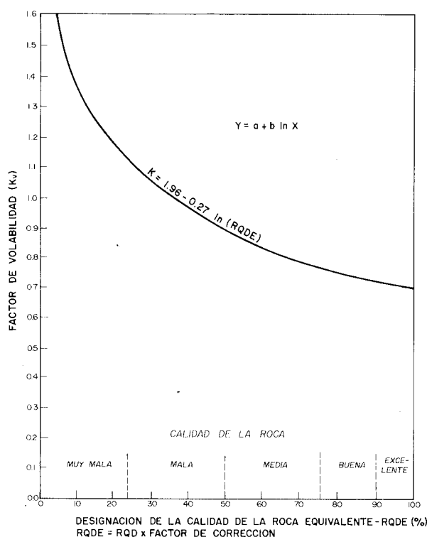
Figura 18.1. Factor de volabilidad ( k_v ) en función del índice de calidad RQDE.
