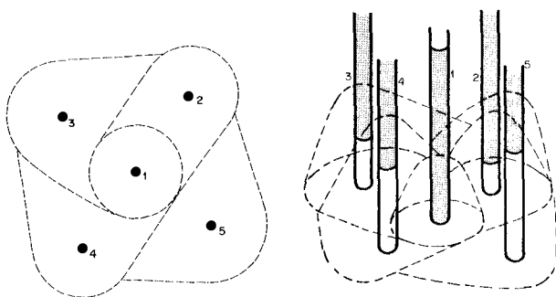
Figura 23.17. Secuencia de encendido y distancia de las cargas a la cara libre.
