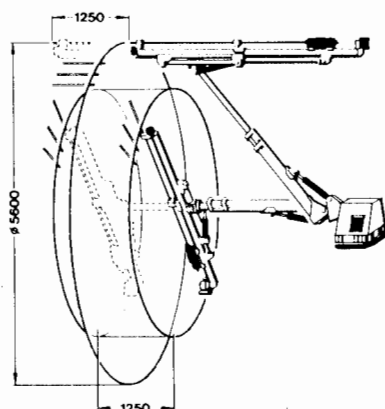
Figura 2.22. Brazo con giro en la base (Atlas Copco).
