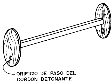
Figura 25.12. Espaciador de madera para cargas de explosivo en barrenos de gran diámetro.
