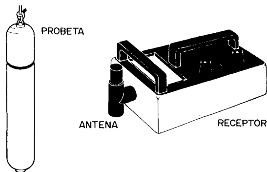
Figura 13.29. Equipo de medida de la piedra.
