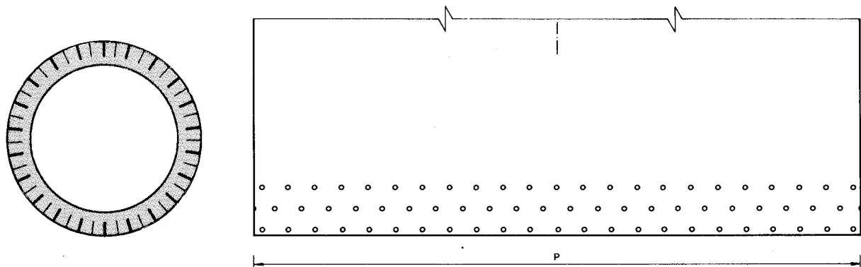
Figura 31.11. Voladura de chimenea con desplome.
