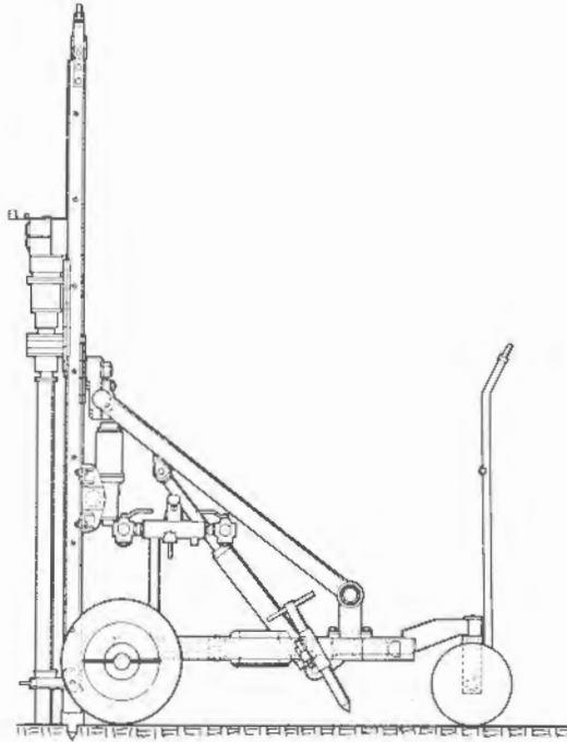
Figura 2.29. Vagón perforador sobre neumáticos.
