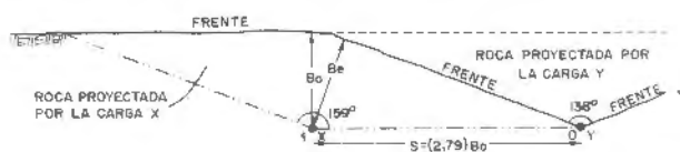
Figura 27.3. Voladura secuenciada con piedra y espaciamiento óptimos (Hagan, 1975).
