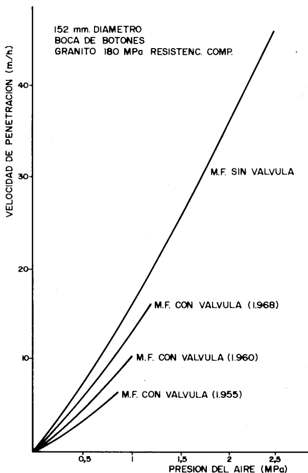
Figura 2.13. Velocidad de penetración para diferentes martillos en fondo y presiones de aire (Ingersoll-Rand).
