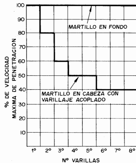
Figura 2.14. Variación de la velocidad de penetración con el número de varillas en los martillos en cabeza y en fondo (Ingersoll-Rand).
