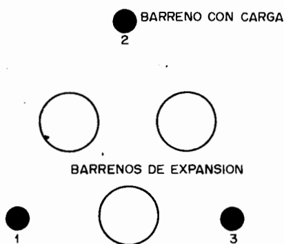
Figura 22.10. Cuele cilíndrico modificado para eliminar la detonación por simpatía y desensibilización dinámica.
