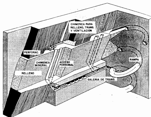
Figura 24.18. Método de explotación por corte y relleno.
