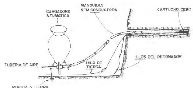
Figura 15.4. Puesta a tierra de una cargadora neumática.
