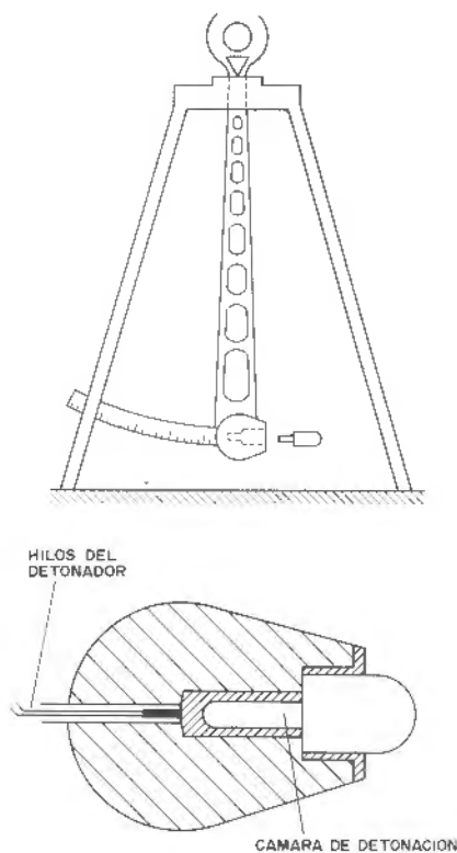
Figura 10.2. Mortero balístico.
