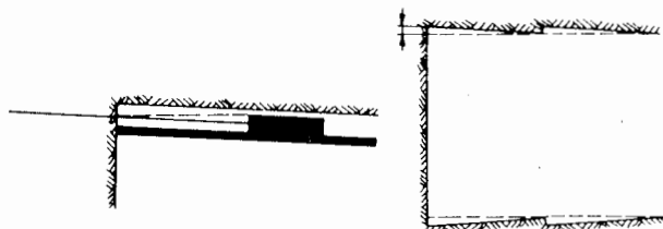
Figura 22.4. Orientación de los barrenos de contorno para mantener el perfil del túnel.
