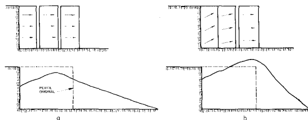
Figura 27.17. Comparación del perfil del material en dos diseños de voladura con distinto retardo entre filas.
