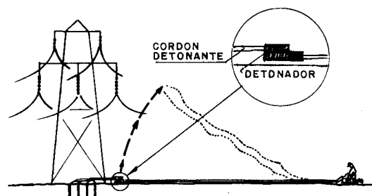
Figura 35.17. Sistema de iniciación recomendado cuando es necesario disparar voladuras en áreas muy próximas a líneas eléctricas.
