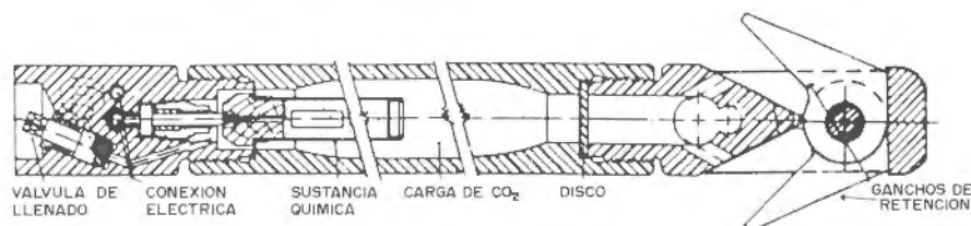
Figura 29.7. Tubo CARDOX.
