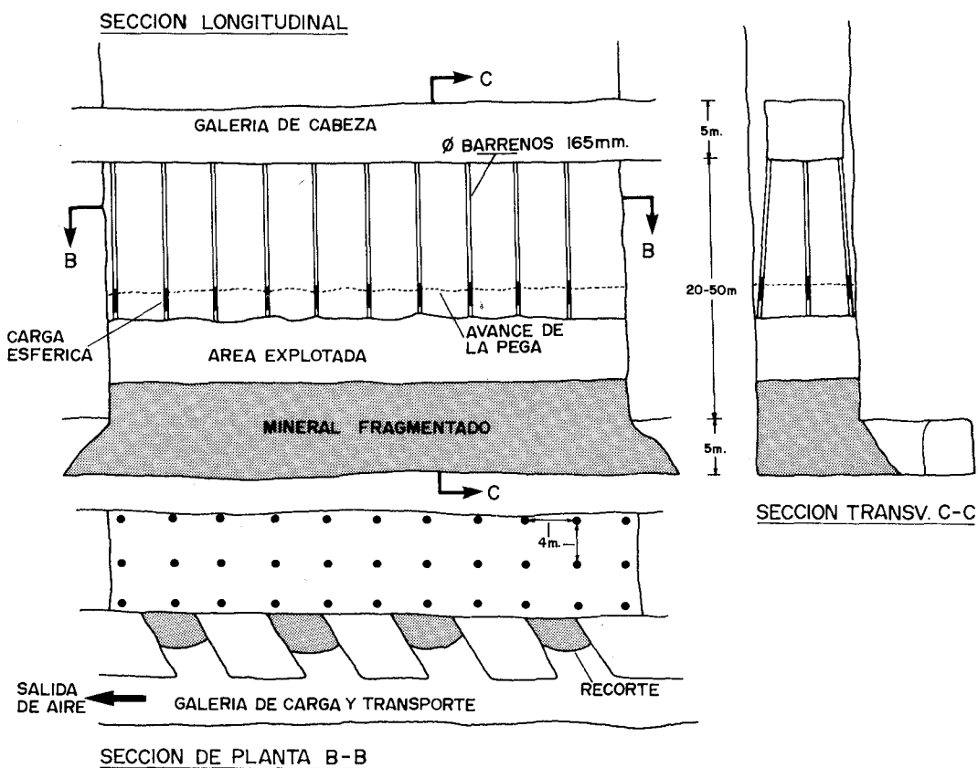
Figura 24.6. Esquema del método de explotación «VCR».
