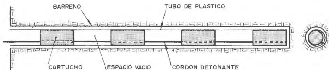
Figura 13.22. Tubo omega.
