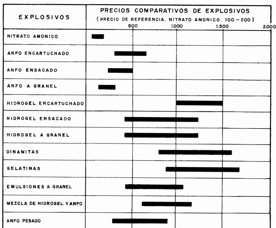
Figura 12.1. Precios comparativos de los explosivos industriales.
