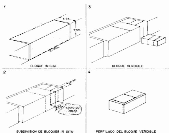
Figura 25.29. Secuencia de arranque de un bloque.
