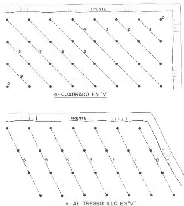
Figura 27.8. Voladura con dos frentes libres.
