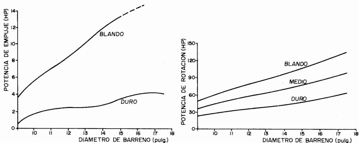
Figura 4.21. Comparación de las potencias de rotación y empuje para diversos tipos de roca.
