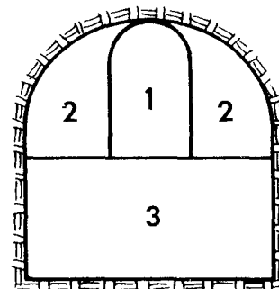
Figura 24.20. Fases de excavación de una cámara pequeña.
