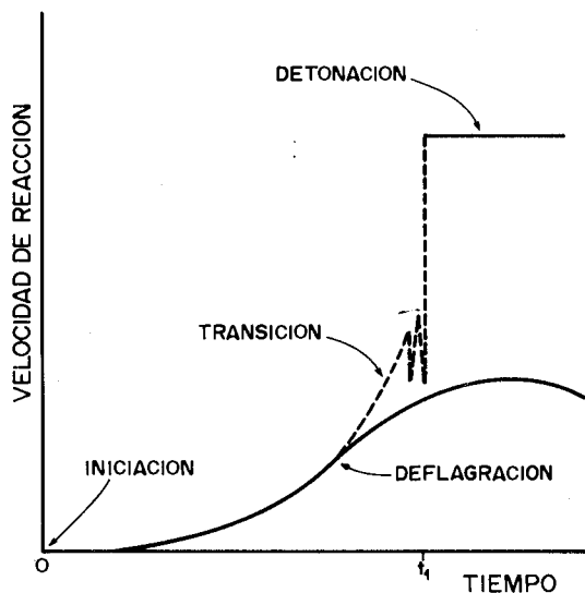
Figura 9.1. Desarrollo de una detonación.
