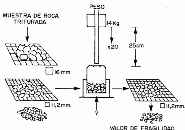
Figura 2.41. Ensayo de friabilidad.
