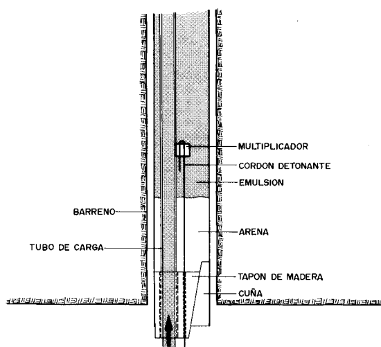
Figura 15.11. Carga entubada y cierre de madera.
