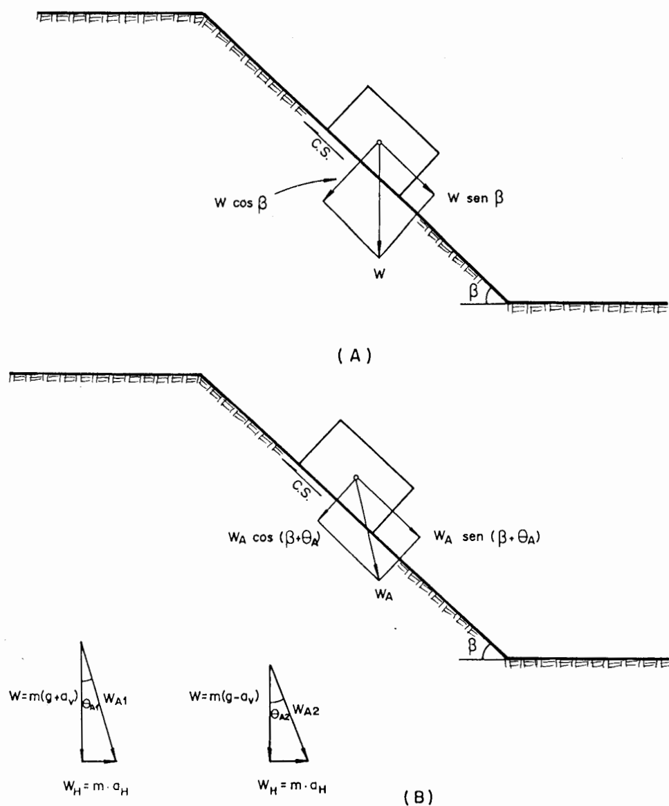
Figura 33.43. Efecto desestabilizador de las vibraciones en un bloque apoyado sobre el talud.
