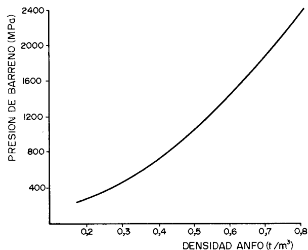
Figura 25.13. Variación de la presión de barreno para distintas mezclas de ANFO de baja densidad.
