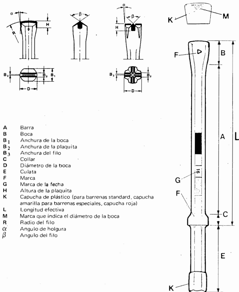
Figura 3.7. Barrenas integrales (Sandvik-Coromant).
