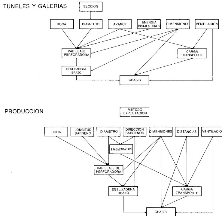
Figura 30.2. Variables que condicionan la selección de equipos de perforación en trabajos subterráneos (Menéndez, F., 1986).
