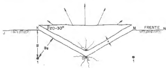
Figura 27.2. Piedra efectiva « B_e » en una voladura secuenciada de una fila (Hagan, 1975).
