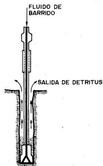
Figura 2.5. Principio de barrido de un barreno.
