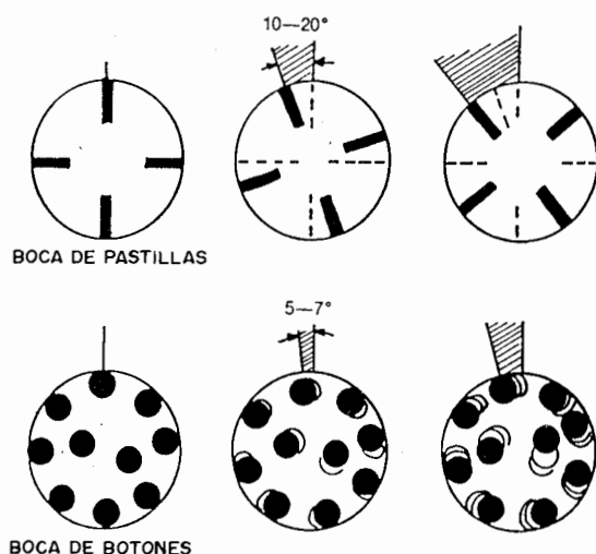
Figura 2.3. Velocidades de rotación para bocas de pastillas y botones.
