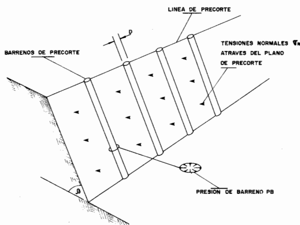
Figura 25.17. Voladura de precorte.
