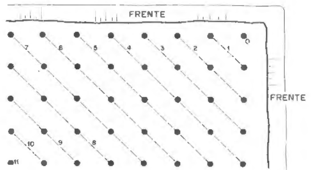
Figura 19.18. Voladura con dos frentes libres.
