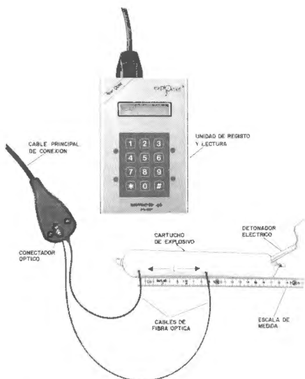
Foto 10.2. Medida de la velocidad de detonación con cronógrafo (Kontinitro A.G.).
