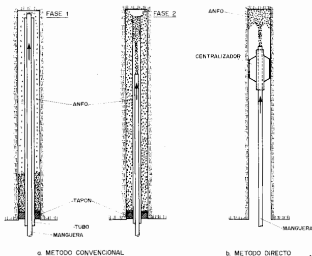
Figura 15.5. Carga neumática de ANFO en barrenos ascendentes.
