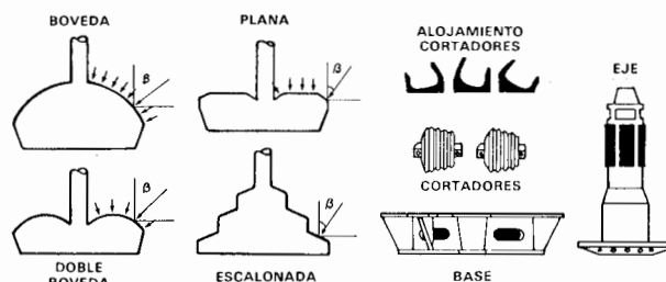
Figura 7.12. Componentes del equipo de escariado.
