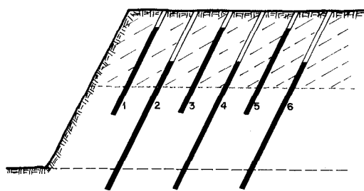
Figura 19.21. Barrenos auxiliares para ayudar a la fragmentación en la parte alta del banco.
