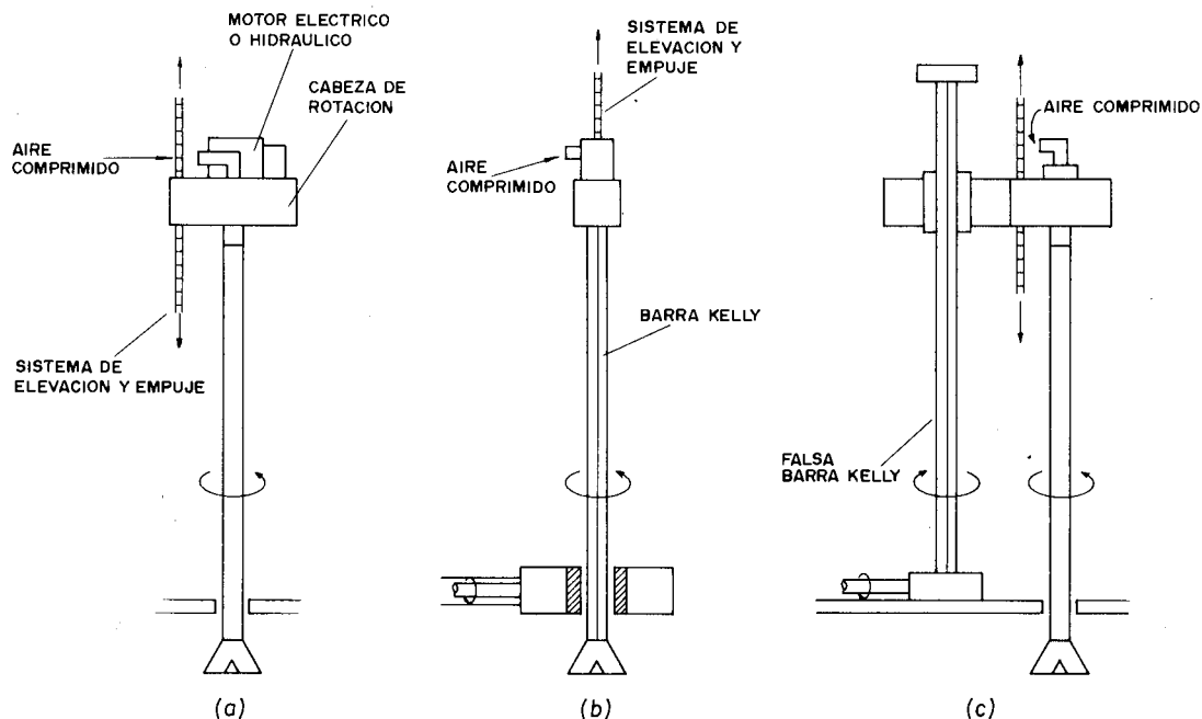
Figura 4.4. Sistemas de rotación: (a) Directo, (b) Mesa de Rotación y (c) Falsa Barra Kelly.
