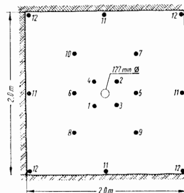
Figura 23.12. Diseño de voladura con barreno central de gran diámetro.
