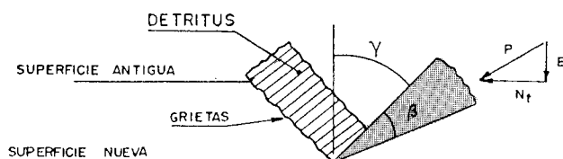
Figura 6.4. Fuerzas que actúan sobre el útil de corte.
