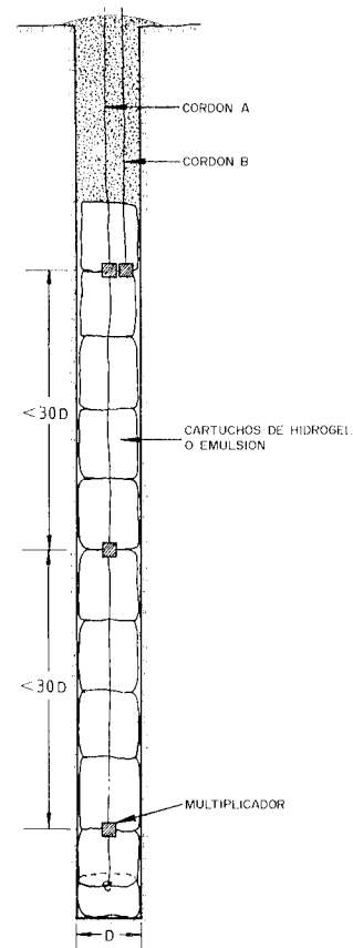
Figura 14.8. Iniciación de hidrógeles o emulsiones encartuchadas.
