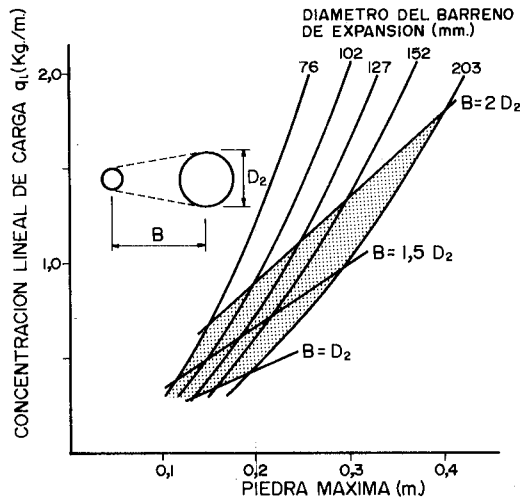
Figura 22.7. Relación entre la concentración lineal de carga y piedra máxima para diferentes diámetros de barrenos de expansión (Larsson y Clark).
