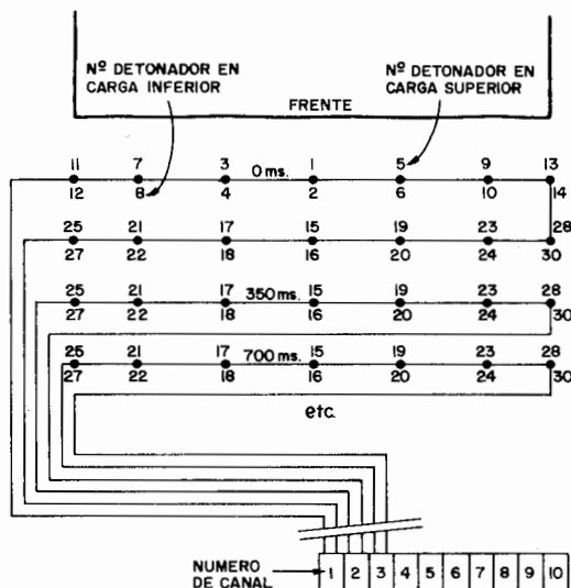
Figura 27.12. Empleo de cargas seccionadas y explosores secuenciales en voladura de bancos verticales con barrenos de gran diámetro.
