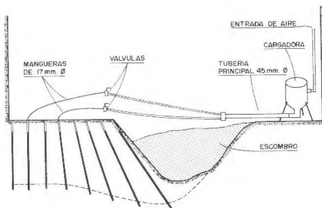
Figura 15.9. Equipo de bombeo de explosivos en la excavación de un pozo.
