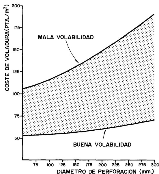
Figura 32.4. Evolución de los costes de voladura sin incluir perforación.
