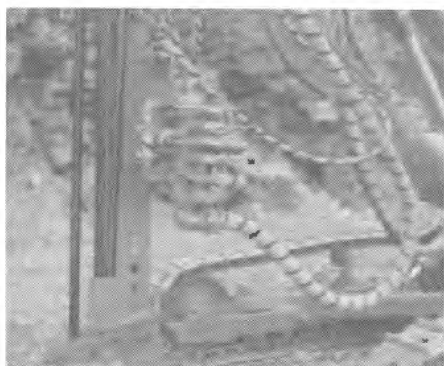
Foto 2.2. Panel de mandos de la perforadora, centralizador y soporte de varillas (Ingersoll-Rand).
