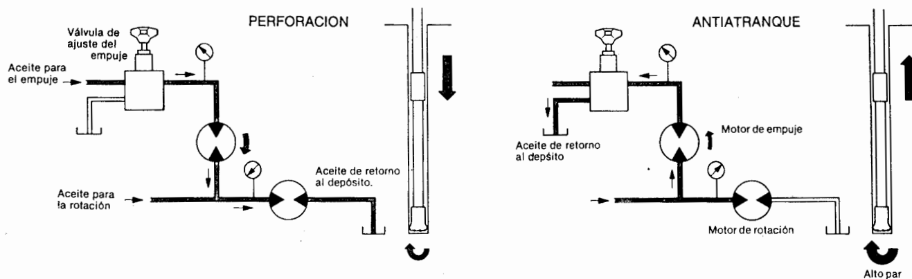
Figura 2.35. Esquema de funcionamiento del sistema antiatranques (Tamrock).
