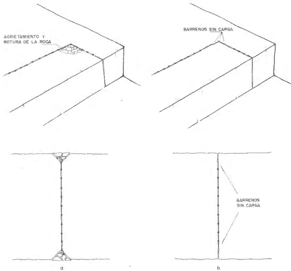
Figura 25.30. Utilización de barrenos guía en la extracción de bloques.
