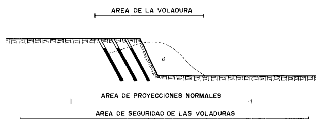
Figura 34.9. Áreas alrededor de las voladuras en función de las proyecciones.
