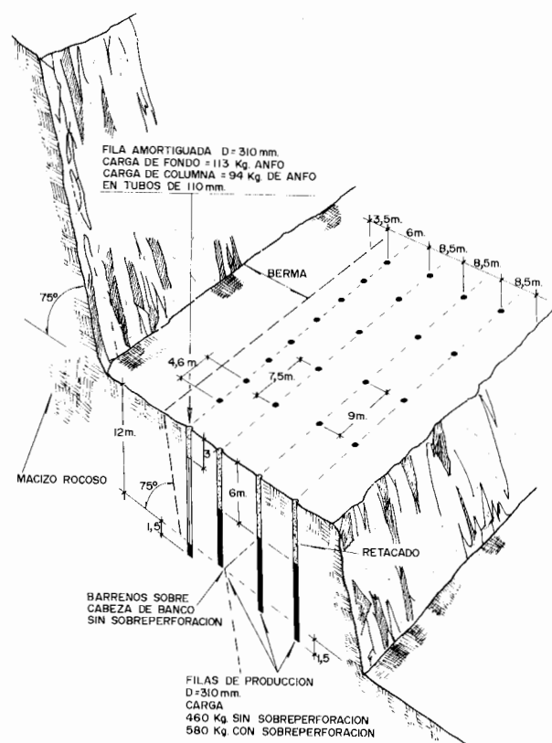
Figura 25.5. Ejemplo de voladura amortiguada.
