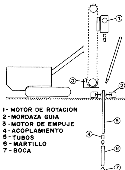
Figura 2.11. Esquema de los componentes de un carro perforador con martillo en fondo.
