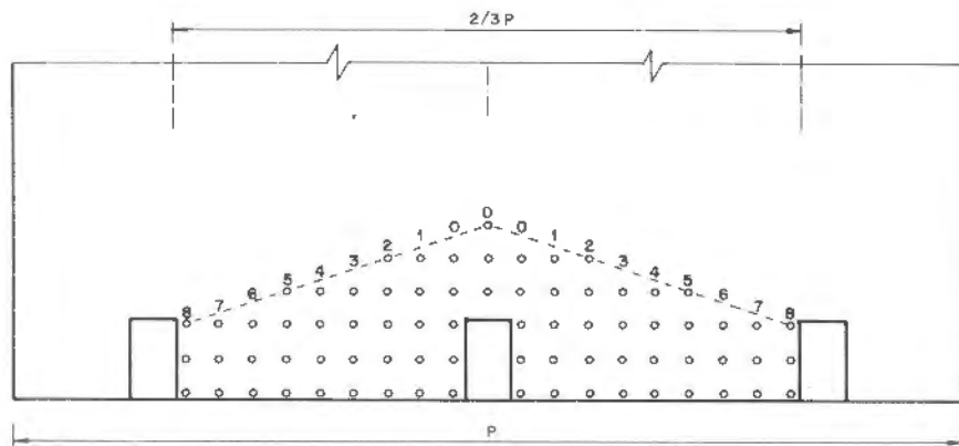
Figura 31.9. Perforación de una chimenea de hormigón.
