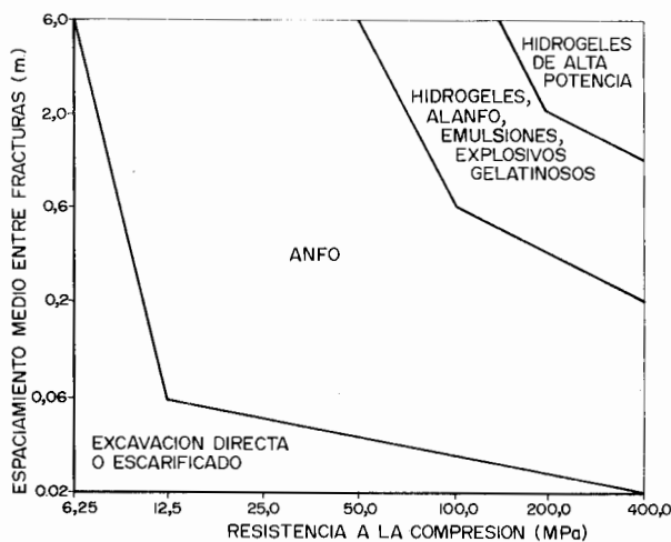
Figura 12.3. Selección de explosivos en función de las propiedades geomecánicas de los macizos rocosos (Brady y Brown, 1985).
