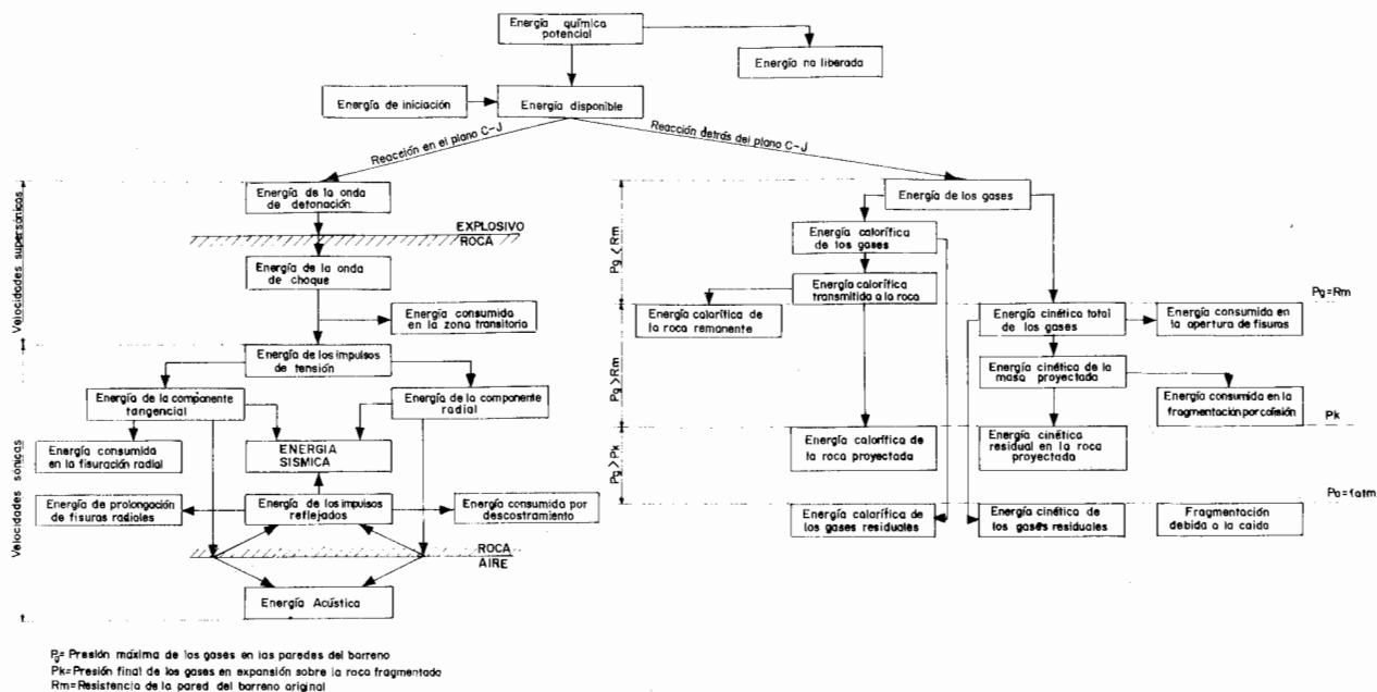
Figura 16.9. Modelo de distribución de la energía del explosivo en una voladura.
