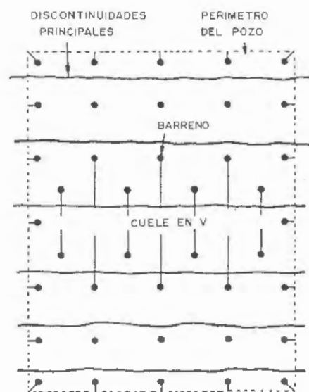
Figura 17.6. Pozo rectangular con cuele en V.
