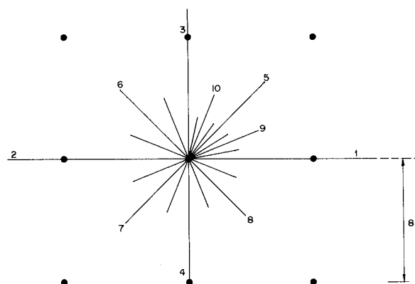
Figura 32.12. Esquema de grietas producidas por una carga de explosivo en una roca homogénea con un esquema cuadrado «B = S».
