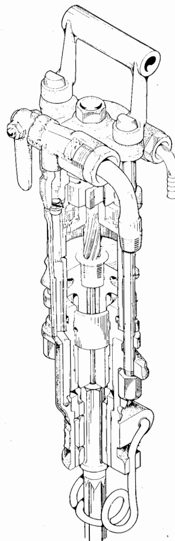
Figura 2.36. Perforadora de mano (Gardner-Denver).
