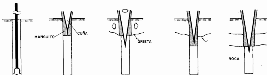
Figura 29.5. Fragmentación de bolos con cuña hidráulica.
