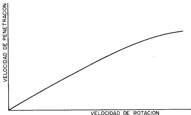
Figura 4.17. Efecto de la velocidad de rotación sobre la velocidad de penetración.
