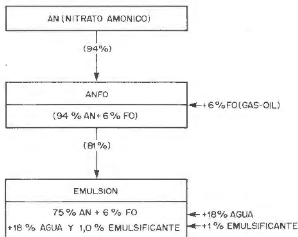
Figura 11.13. Composición básica de una emulsión.
