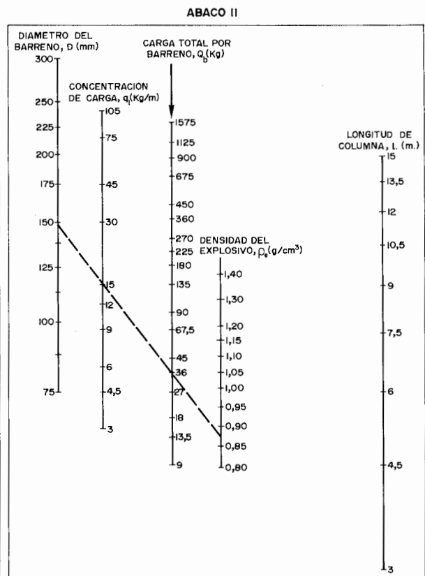
Figura 20.6. Abaco II.
