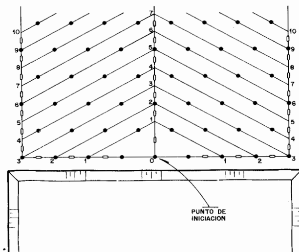
Figura 21.5. Esquema triangular con secuencia de encendido en «V1».
