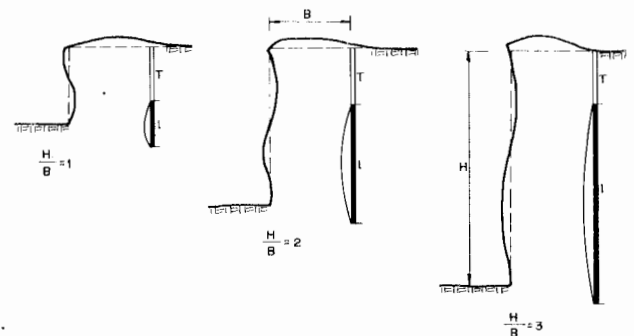
Figura 19.5. Estados de flexión de un banco con distintas relaciones H/B (Ash).
