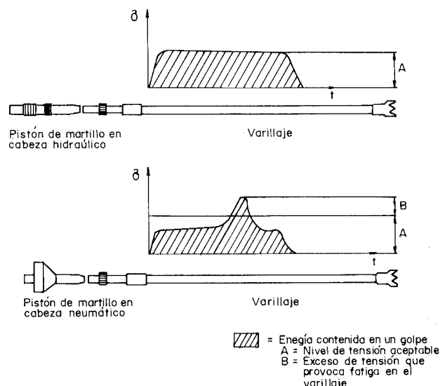
Figura 2.9. Ondas de choque en martillos hidráulicos y neumáticos.
