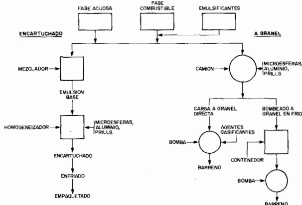
Figura 11.14. Esquema de producción de emulsiones.
