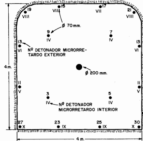
Figura 22.23. Doble cuele cráter usando barrenos centrales de 200 mm.
