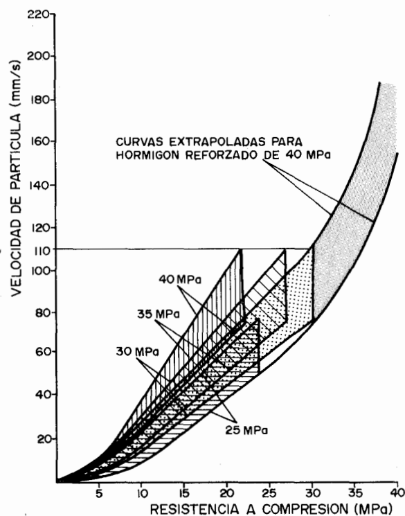
Figura 33.46. Niveles de vibración admisibles según la resistencia del hormigón.
