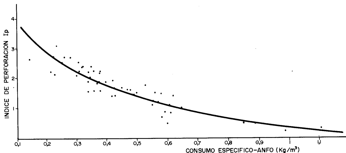
Figura 18.16. Correlación entre el índice «Ip» y el consumo específico (L. Jimeno).
