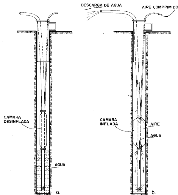
Figura 15.13. Bomba neumática.
