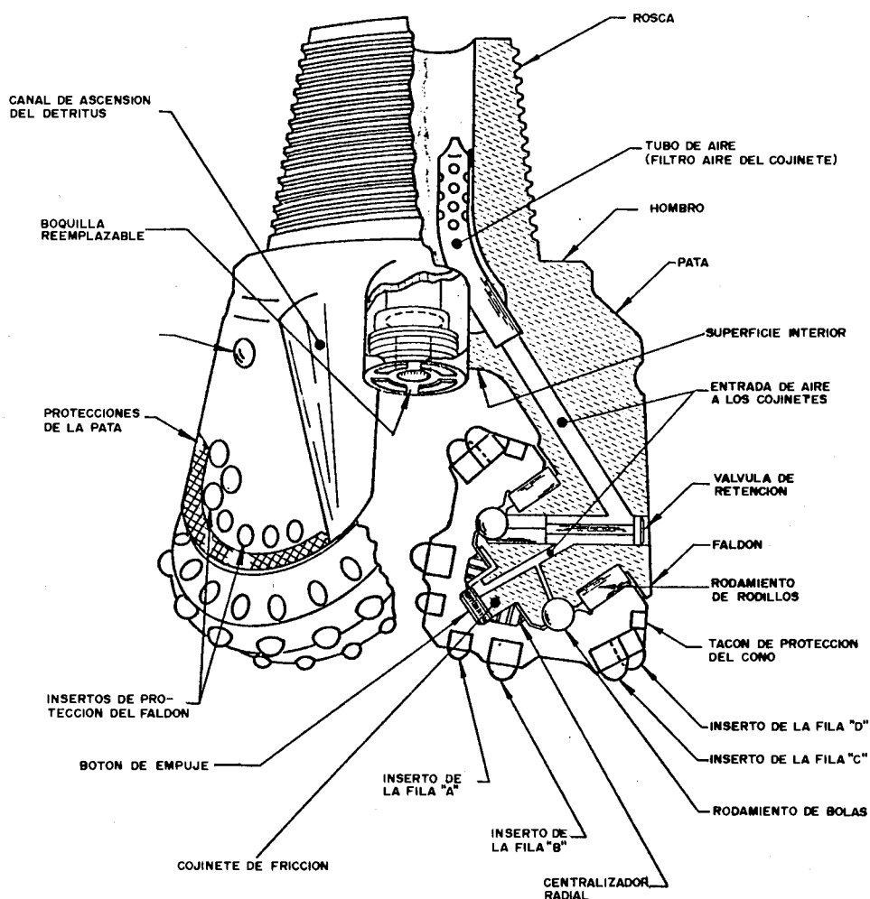
Figura 5.1. Esquema de tricono (Smith-Gruner).
