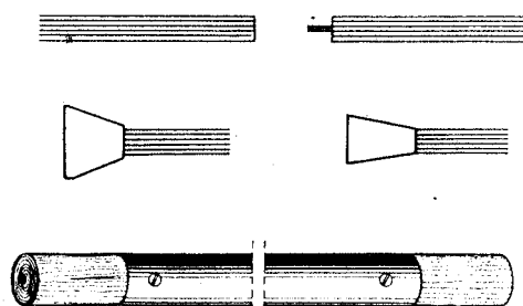
Figura 13.27. Atacadores.
