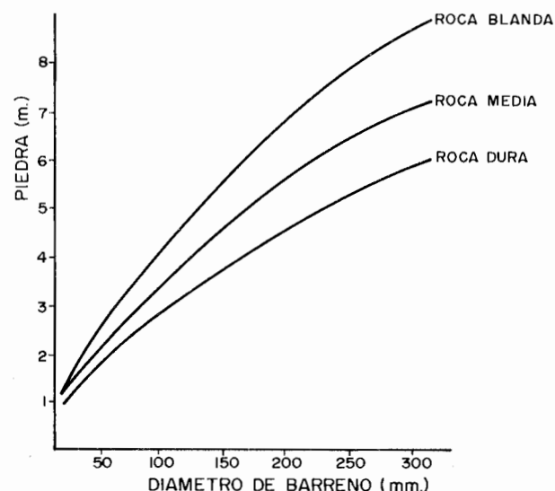
Figura 19.11. Dimensión de la piedra en función del diámetro de perforación.
