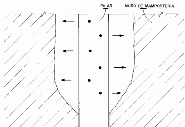
Figura 31.20. Rozas abiertas en tabiques adosados a un pilar.
