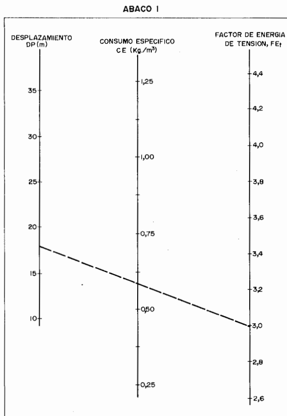
Figura 20.5. Abaco I.
