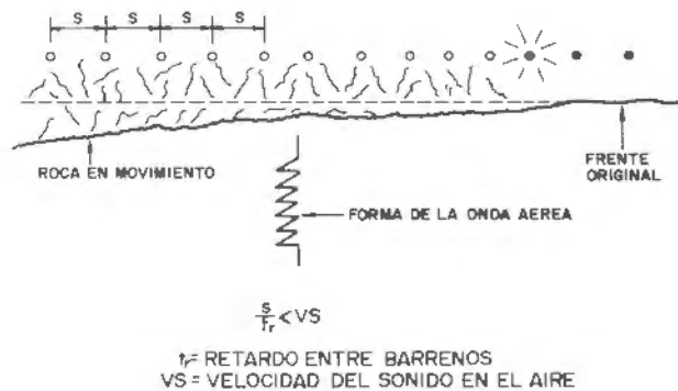
Figura 33.50. Progresión de una voladura a lo largo de un frente y simulación de la onda aérea.
