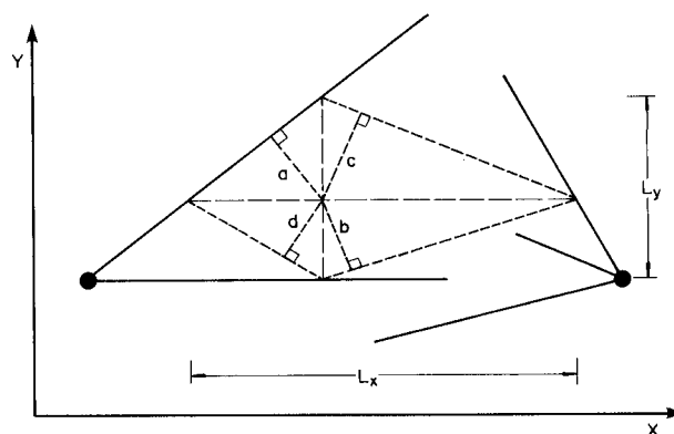
Figura 32.13. Determinación del tamaño del bloque.
