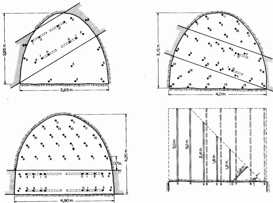
Figura 22.28. Voladuras en galerías con capas de carbón.
