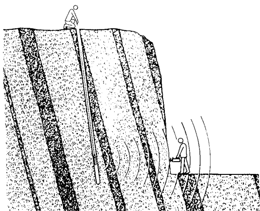
Figura 13.29. Equipo de medida de la piedra.
