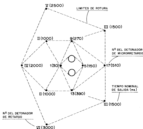
Figura 27.20. Secuencia recomendada en un cule de barrenos paralelos.
