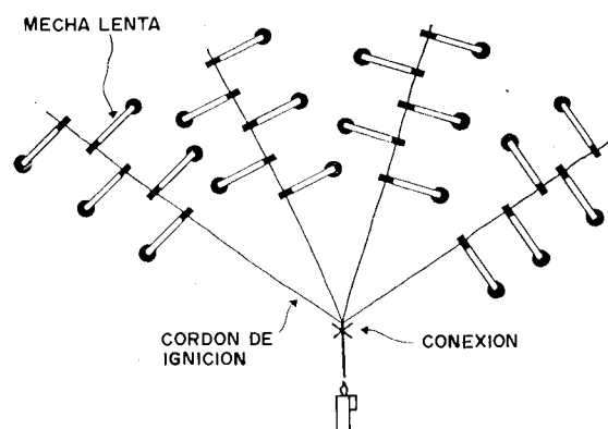
Figura 13.10. Sistema de encendido rápido de mecha de seguridad.
