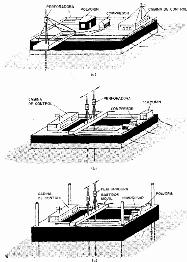
Figura 26.1. Tipos de pontonas flotantes y plataforma autoelevable.
