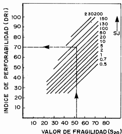
Figura 2.43. Ábaco de cálculo del D.R.I.
