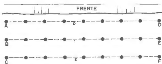
Figura 19.17. Voladura con un frente libre.
