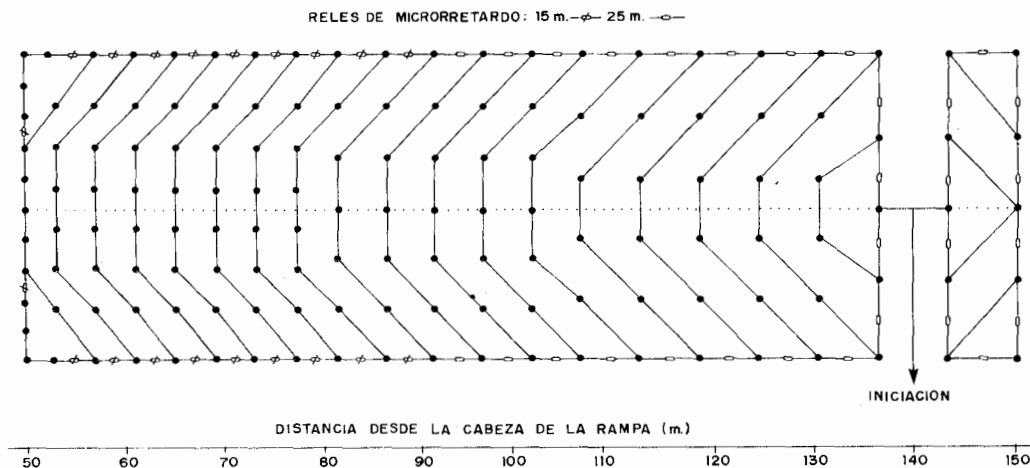
Figura 21.13. Secuencia de encendido con relés de microrretardo en una voladura en rampa.
