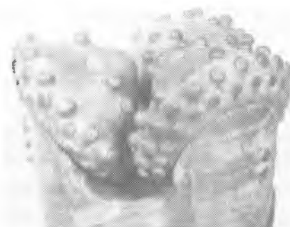
Foto 5.9. Desgaste de faldón (Hughes Tool Co).
