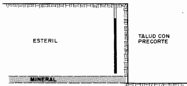
Figura 20.3. Comparación de dos frentes sin y con precorte activo.
