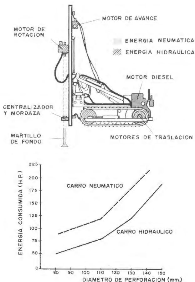
Figura 2.33. Ahorro de energía en perforadoras neumáticas con martillo en fondo y accionamientos hidráulicos.
