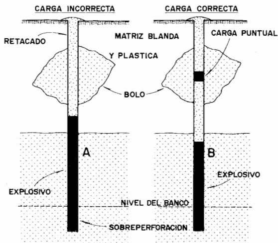
Figura 18.12. Fragmentación de bolos dentro de matrices de material plástico (Hagan y Reid).
