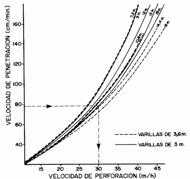
Figura 2.45. Velocidades de perforación obtenidas para diferentes alturas de banco considerando unos tiempos de 5 min. en el desplazamiento y emboquille y 1,9 min. en la maniobra de varillas.
