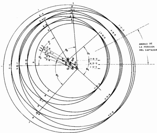
Figura 33.7. Direcciones preferentes de cooperación de ondas en una voladura múltiple (Wiss y Linehan).
