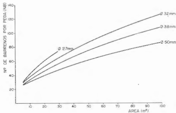
Figura 22.18. Número de barrenos por pega en función del área.
