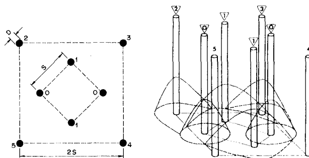
Figura 23.18. Esquema de voladura en chimenea con el método «VCR».
