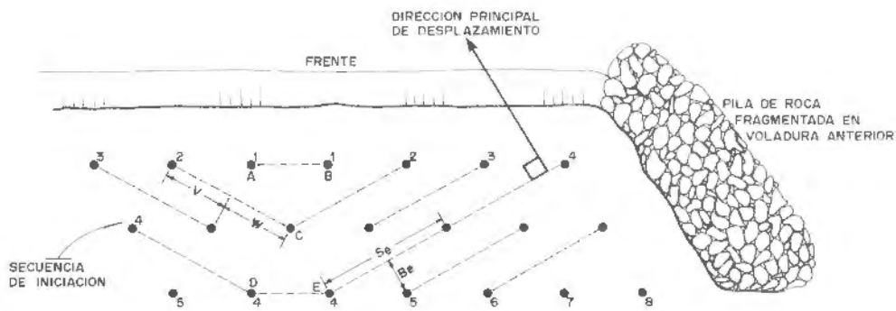
Figura 19.16. Disparo de voladuras con un frente cubierto.
