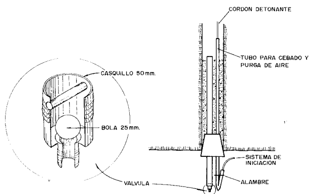
Figura 15.10. Cierre de madera con válvula antirretorno.
