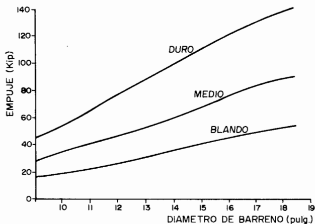
Figura 4.22. Empuje sobre la boca en función del diámetro y del tipo de roca (1 Kip = 4,448 KN).
