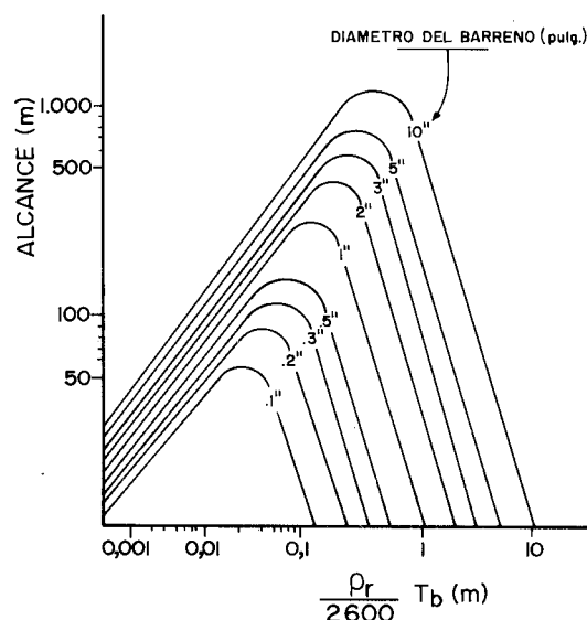
Figura 34.2. Alcances máximos de las proyecciones en función del tamaño de los fragmentos y diámetro de los barrenos (Lundborg y otros).
