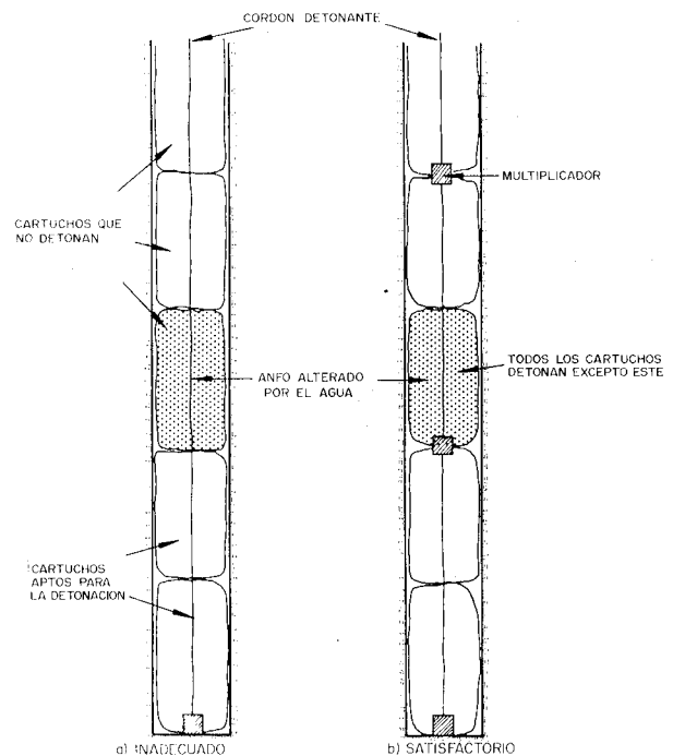
Figura 14.6. Colocación de multiplicadores en columna de explosivo formada por cartuchos de ANFO.
