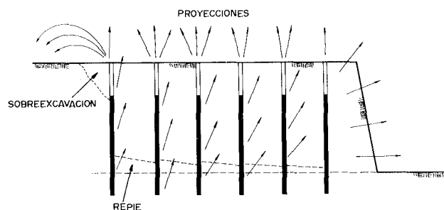
Figura 27.18. Efectos negativos en una voladura múltiple con pequeño retardo entre filas.
