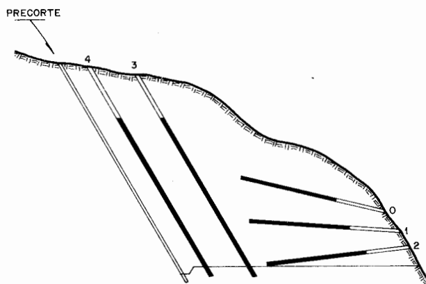
Figura 21.8. Secuencia de encendido en sección con barrenos verticales y zapateras.
