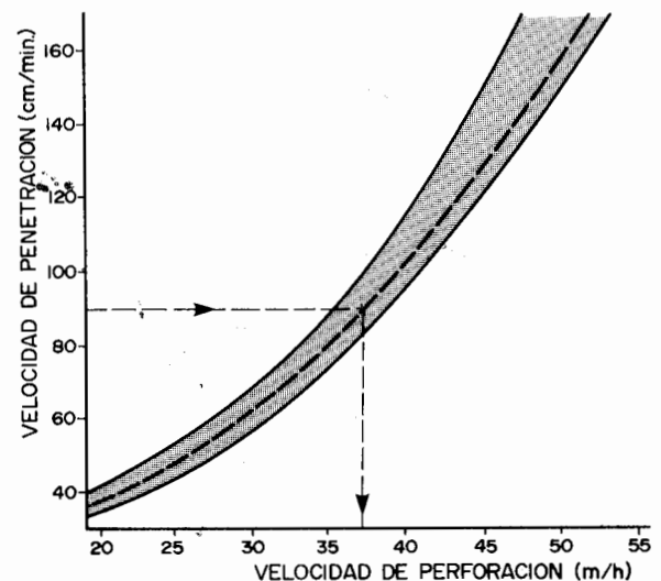
Figura 2.46. Velocidades medidas de perforación en el avance mecanizado de túneles y galerías.
