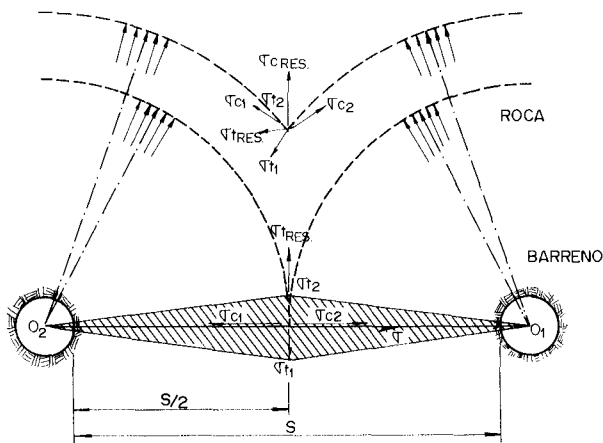
Figura 25.2. Estado de tensiones generado por la superposición de las ondas de choque producidas por el disparo simultáneo de dos cargas.
