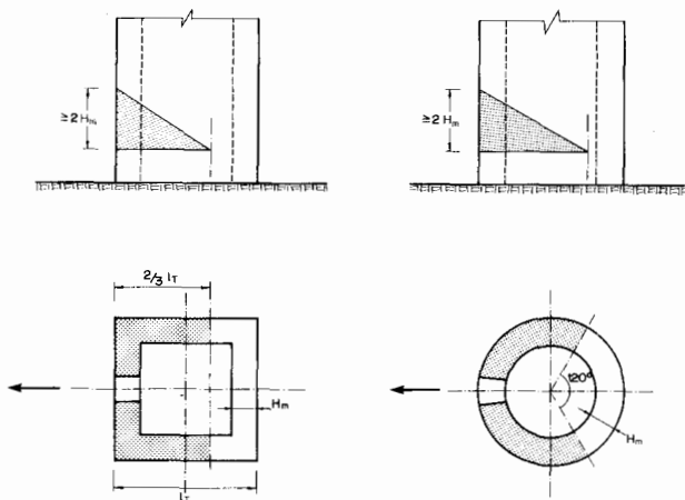
Figura 31.13. Demolición de torres de sección cuadrada y circular.
