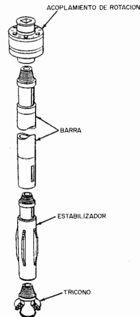
Figura 4.9. Sarta de perforación.
