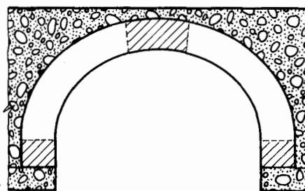
Figura 31.15. Voladura de una bóveda por partes.
