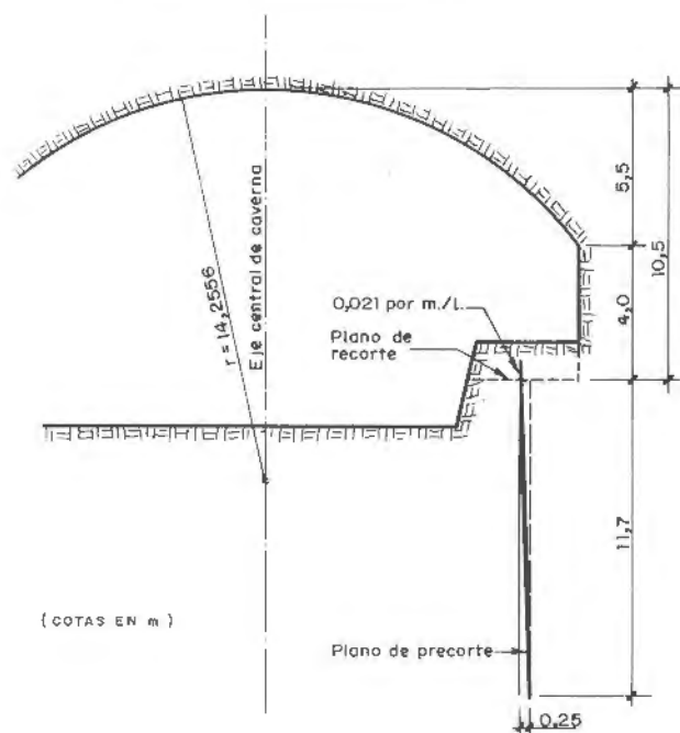
Figura 24.22. Detalle de cámara con viga carril apoyando en roca. (Cortesía de Iberduero, S. A.).
