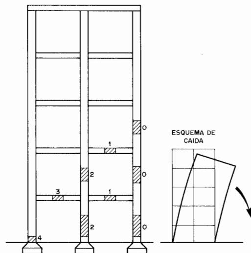
Figura 31.21. Demolición de un edificio con caída en una dirección.
