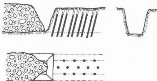
Figura 21.9. Excavación de una zanja.
