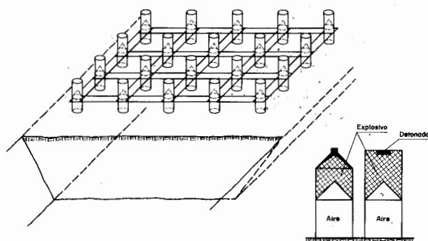
Figura 26.10. Utilización de cargas huecas en voladuras submarinas.
