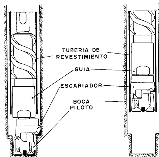
Figura 7.3. Método ODEX (Atlas Copco).
