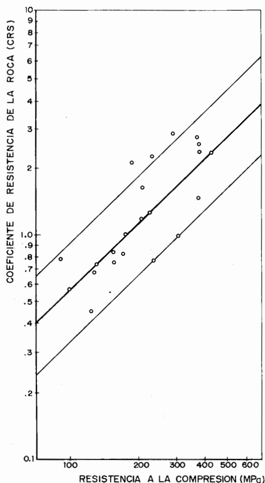
Figura 2.39. Relación entre la Resistencia a la Compresión y el Coeficiente de Resistencia de la Roca.
