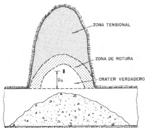
Figura 24.4. Dimensiones de las cavidades creadas por cargas esféricas con frentes invertidos (Lang).
