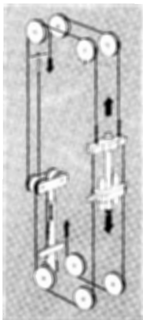
Figura 4.6. Sistema de empuje por Cilindro Hidráulico (Ingersoll-Rand).
