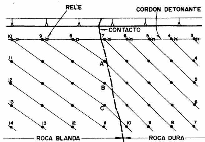
Figura 17.2. Cambio de esquema recomendado. B = B' S \neq S' .
