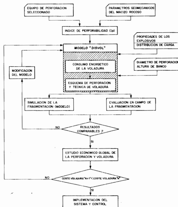
Figura 18.20. Estructura del modelo de optimización de costes (L. Jimeno).
