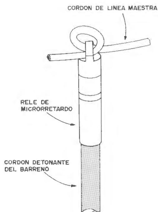
Figura 13.7. Relé de microrretardo en barreno.
