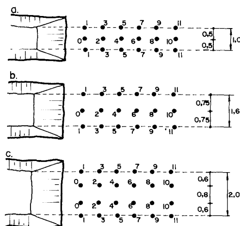
Figura 21.10. Secuencias de encendido.
