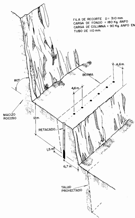
Figura 25.4. Ejemplo de voladura de recorte.
