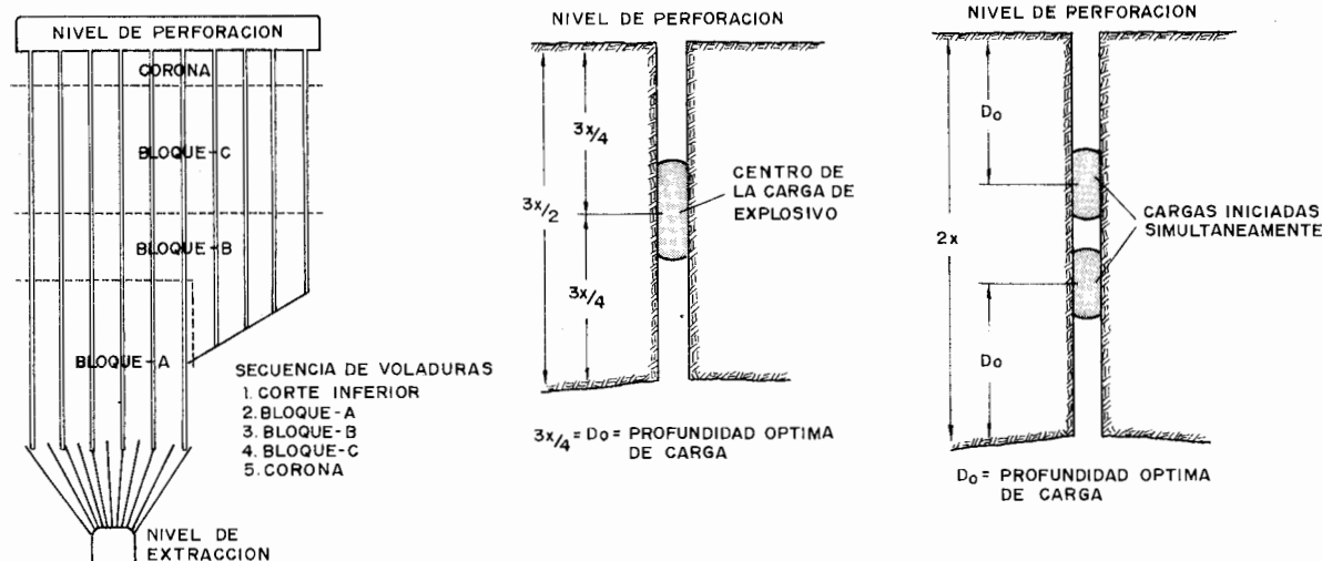
Figura 24.10. Disposición de las cargas de explosivo en el pilar corona.
