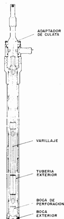
Figura 7.1. Método OD (Atlas Copco).
