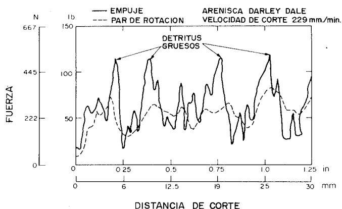
Figura 6.3. Curvas de Desplazamiento - Fuerza de una boca de corte.
