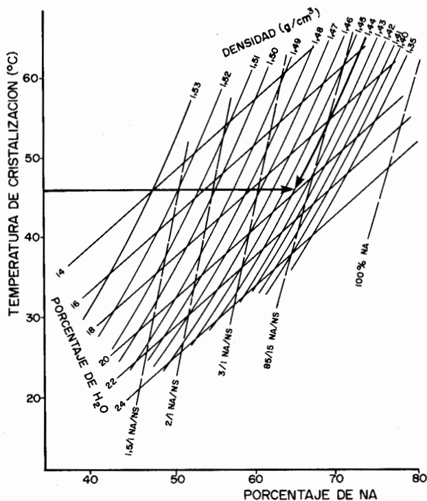
Figura 11.11. Temperatura de cristalización del sistema NA/NS/AGUA según la composición y densidad.
