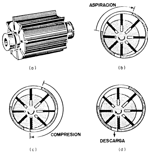
Figura 8.3. Compresor de paletas.
