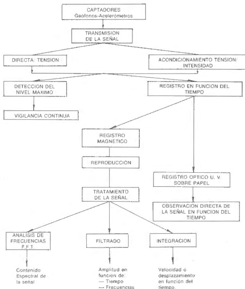
Figura 33.15. Esquema general de registro y análisis de las vibraciones.
