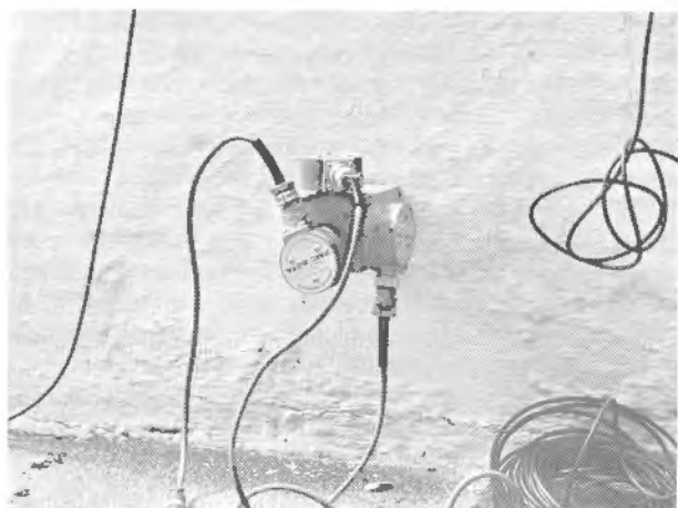
Foto 33.3. Estación de registro triaxial constituida por tres acelerómetros.
