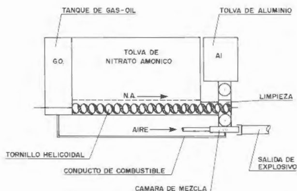
Figura 15.7. Depósitos de un camión de mezcla y carga.
