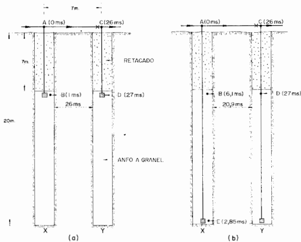
Figura 14.10. Menor probabilidad de cortes con cebado en fondo.
