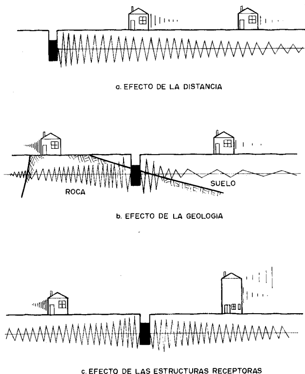
Figura 33.4. Modificación de las vibraciones al propagarse por terrenos de diferente estructura y características.
