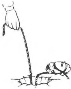
Figura 35.13. Comprobar el ascenso del explosivo durante la carga.
