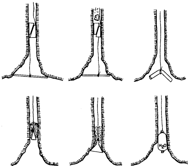
Figura 24.7. Sistemas de cierre de los barrenos (Mitchell).
