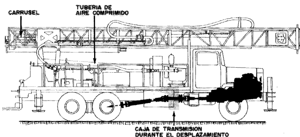
Figura 4.3. Esquema de accionamiento de una perforadora diesel con un motor único.
