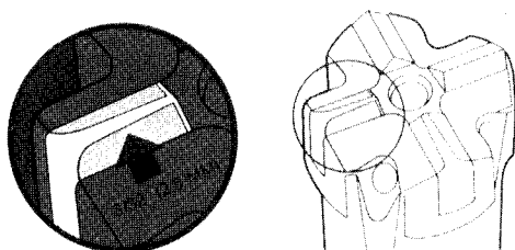
Figura 3.19. Desgaste del filo de las pastillas.
