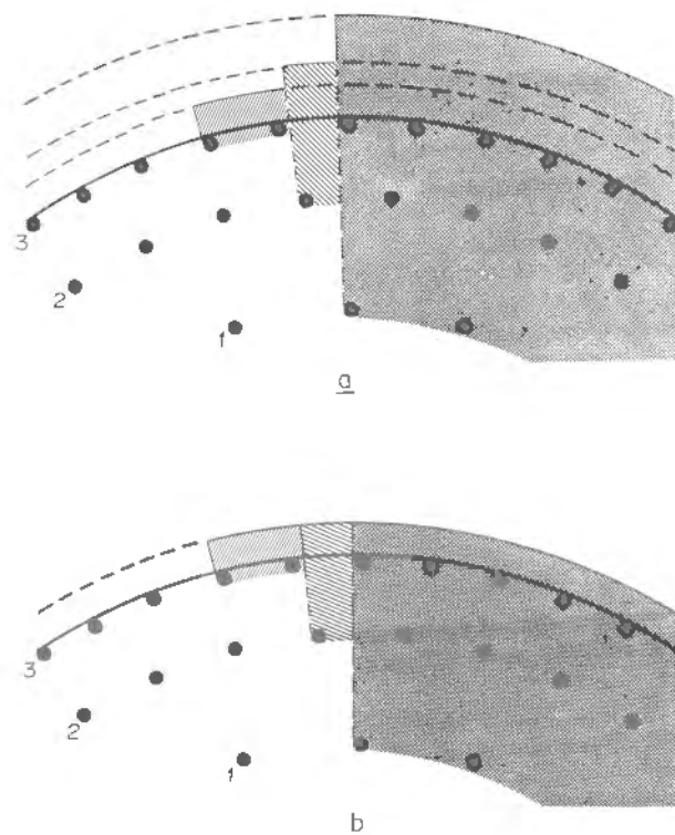
Figura 25.23. a) Cargas incorrectas. b) Cargas correctas (Holmberg y otros).
