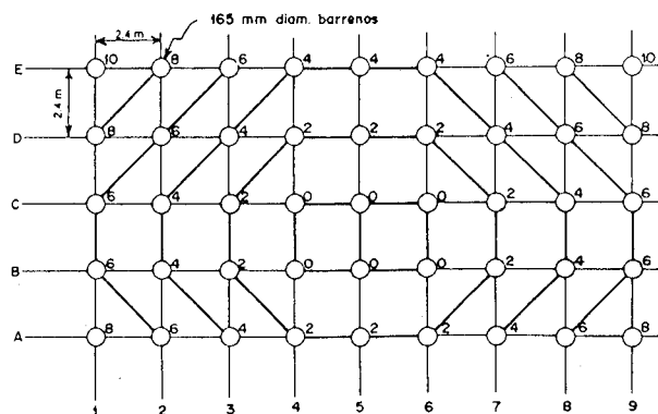
Figura 24.9. Ejemplo de secuencia de encendido.
