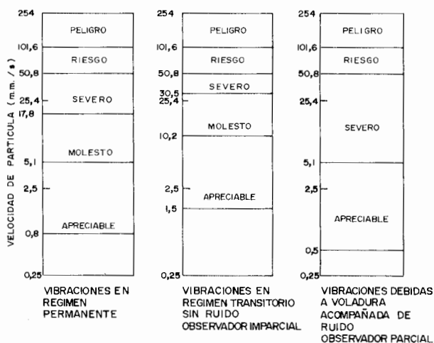
Figura 33.40. Respuesta humana a las vibraciones según vayan acompañadas o no de ruidos (Oriard).
