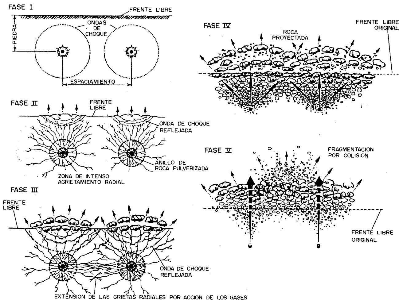
Figura 16.8. Resumen de mecanismos de rotura.
