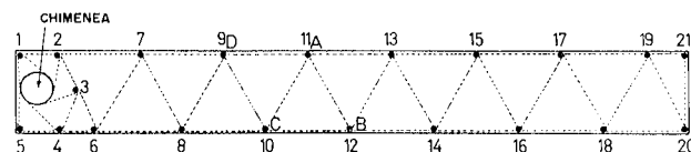
Figura 24.13. Esquema de perforación y encendido en el corte lateral o principio de sección.
