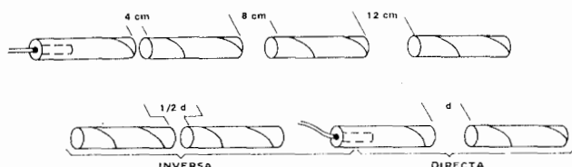
Figura 10.7. Ensayo de transmisión por simpatía.
