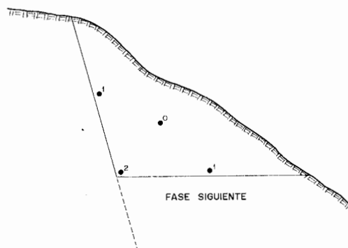
Figura 21.3. Apertura de pistas de acceso para posteriores excavaciones a media ladera.
