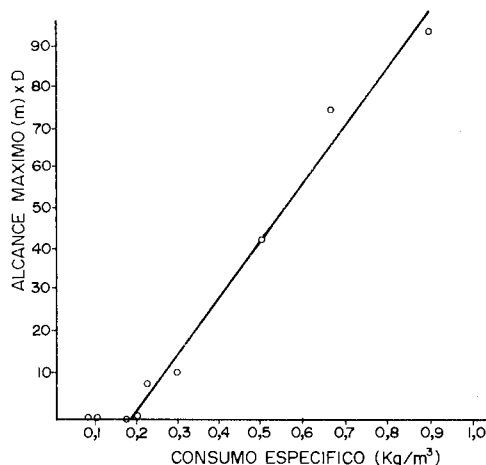
Figura 34.3. Alcances máximos en las voladuras en banco en función de los consumos específicos de explosivo (Lundborg y otros).
