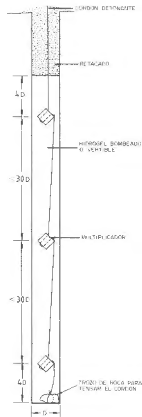
Figura 14.7. Iniciación de hidrógeles o emulsiones verticales o bombeables.
