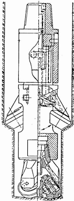
Figura 4.13. Sistema de ensanche de barrenos.
