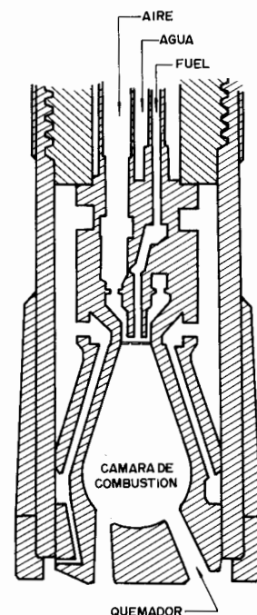
Figura 7.14. Sección de un quemador.
