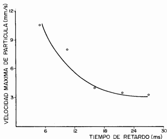
Figura 33.8. Influencia del intervalo de retardo en el nivel máximo de vibración.
