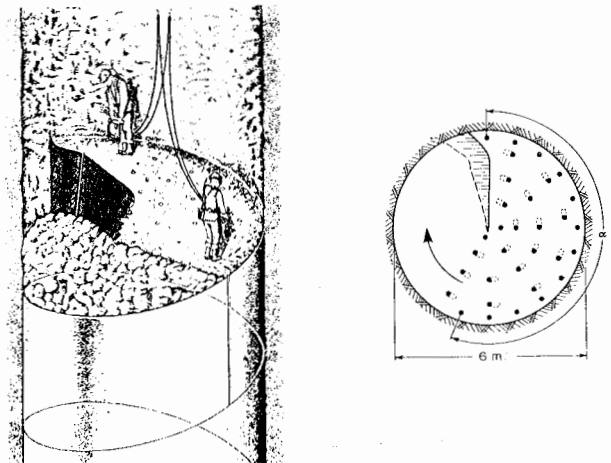
Figura 23.2. Método de espiral.
