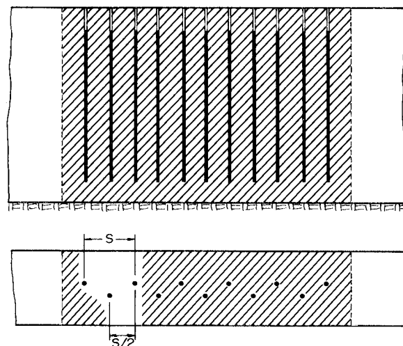
Figura 31.3. Voladura de un muro alto y estrecho.
