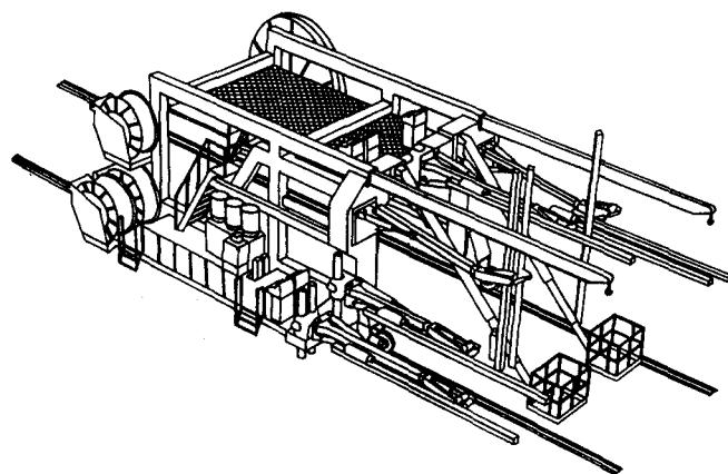
Figura 2.24. Jumbo de tipo pórtico (Tamrock).
