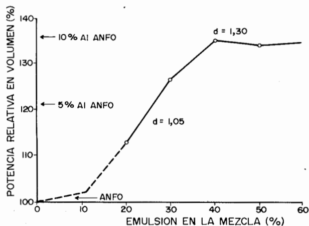
Figura 11.17. Variación de la potencia y densidad de un ANFO Pesado según el porcentaje de emulsión (Bamptfield y Morrey, 1984).
