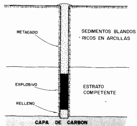
Figura 18.8. Distribución de carga en estrato duro con zona de alteración.
