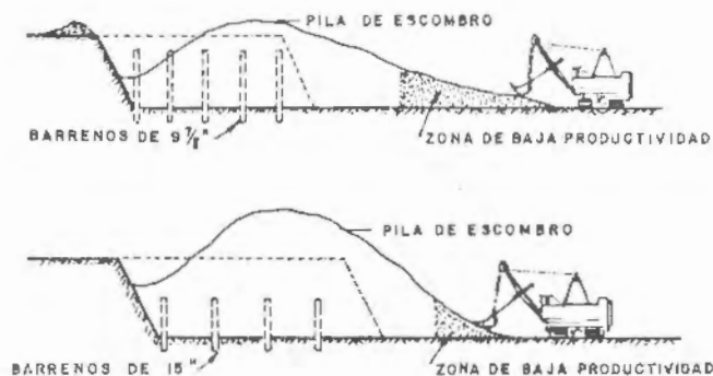
Figura 19.3. Zonas de baja productividad para excavadoras de cables.
