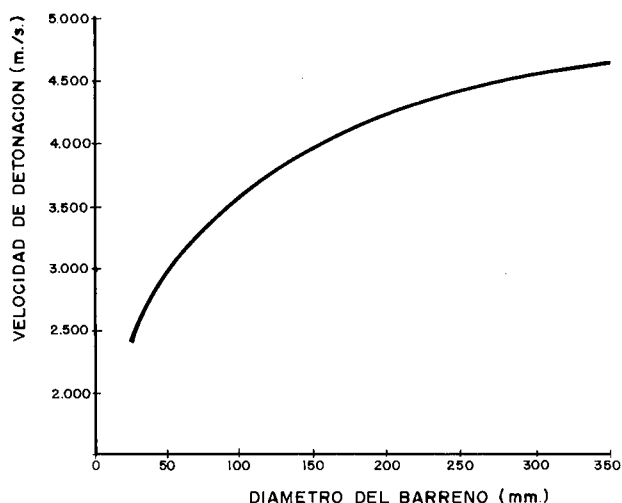
Figura 11.7. Influencia del diámetro de la carga sobre la velocidad de detonación.
