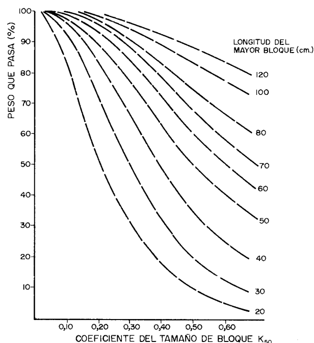
Figura 32.9. Curvas granulométricas teóricas del material volado para diferentes valores de « K_{50} ».
