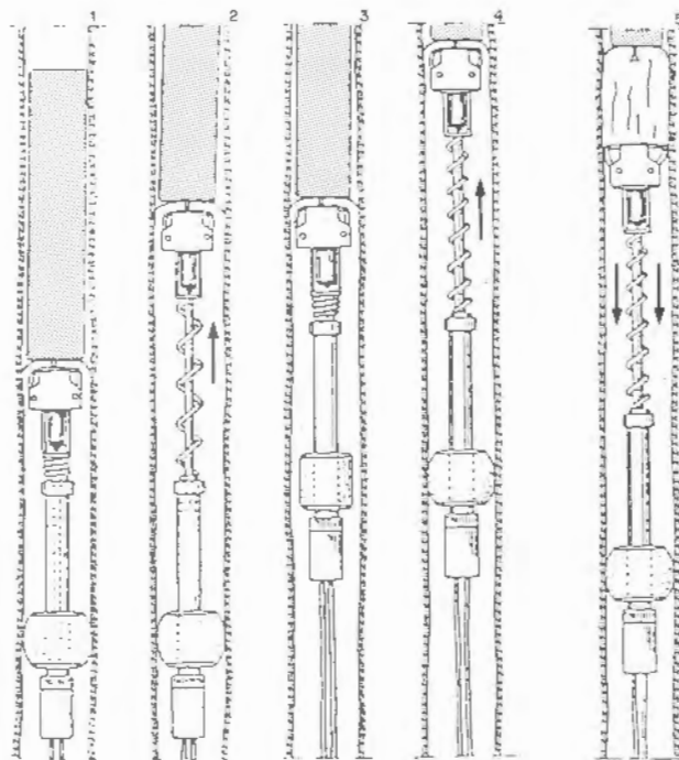
Figura 15.2. Cargador de cartuchos «Half-Pusher» (Nitro-Nobel).
