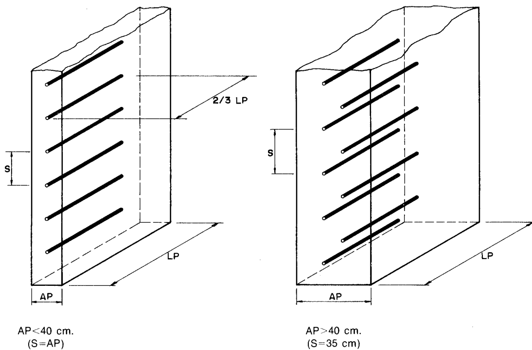
Figura 31.4. Voladura de pilares de hormigón.
