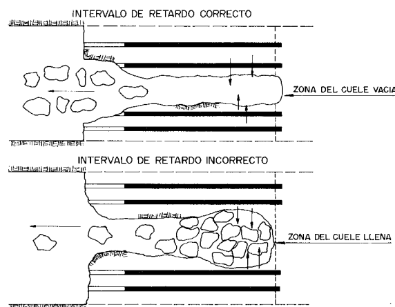
Figura 27.21. Efecto del tiempo de retardo de los barrenos del cule sobre el rendimiento de la voladura en túnel.
