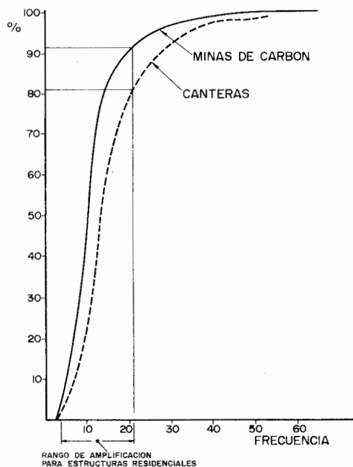
Figura 33.3. Frecuencias de vibración predominantes en minas de carbón y canteras (Ball, M. J., 1981).
