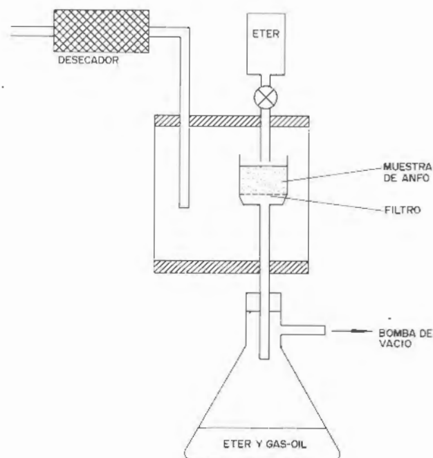
Figura 11.3. Procedimiento de laboratorio para medir el porcentaje de gas-oil.
