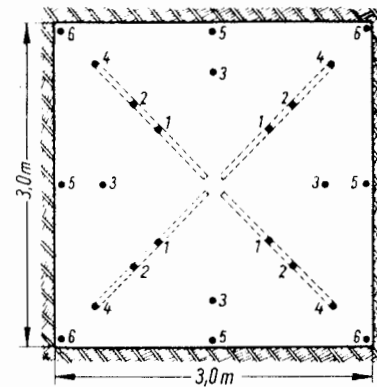
Figura 23.11. Esquema de perforación y secuencia de encendido en una chimenea con el método manual.
