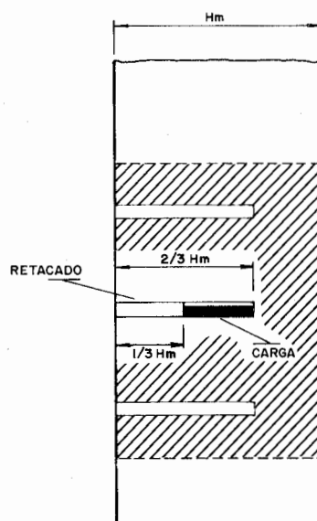
Figura 31.1. Sección transversal de un muro y geometría de las cargas.
