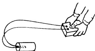
Figura 35.16. Comprobación de detonadores eléctricos.
