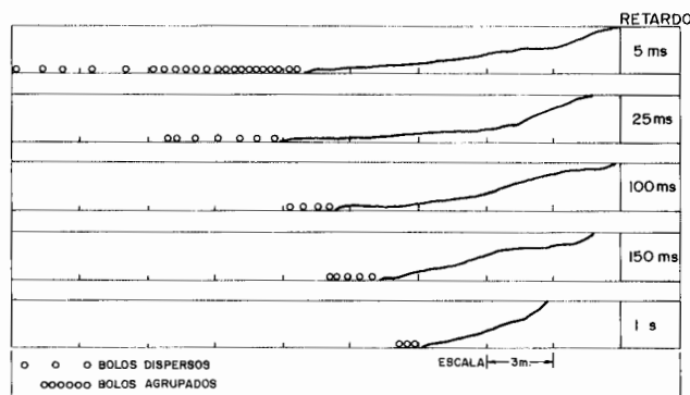
Figura 27.22. Efecto del retardo sobre el desplazamiento y forma de la pila de escombros (Du Pont).
