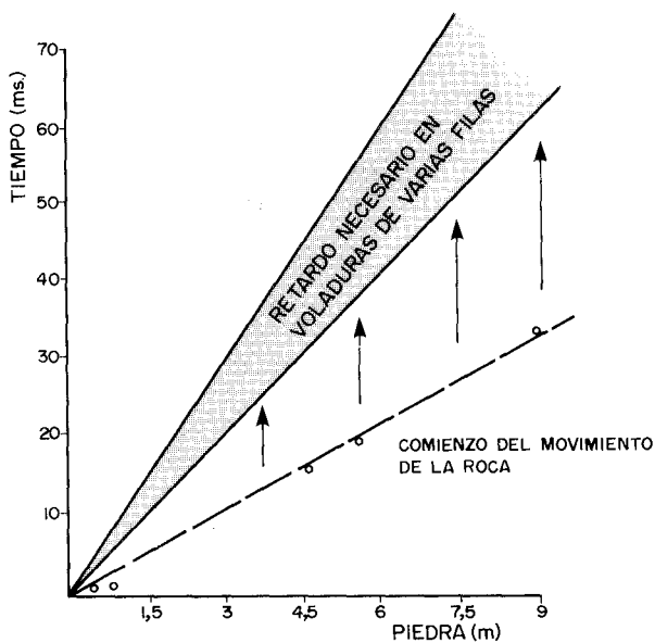
Figura 27.14. Tiempos de comienzo del movimiento del frente para distintos esquemas en roca dura (Bauer).
