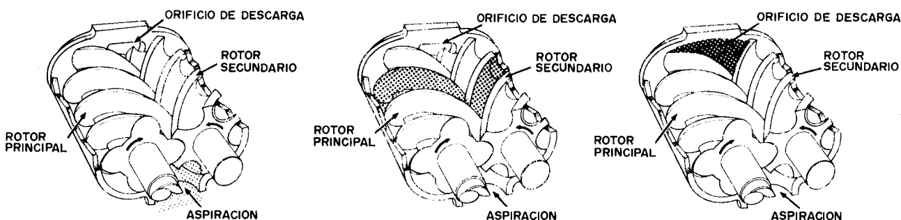
Figura 8.1. Principio de funcionamiento de un compresor de tornillo.
