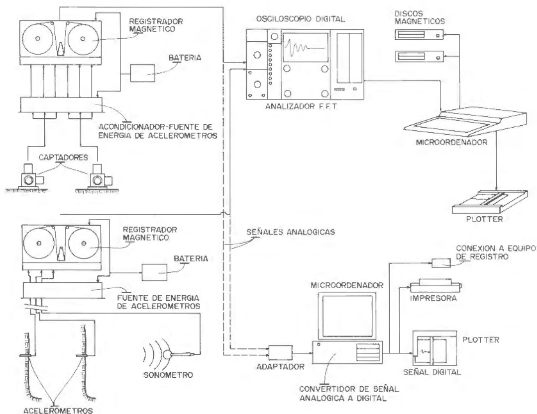
Figura 33.18. Cadenas de instrumentación para registro y análisis de vibraciones y onda aérea.
