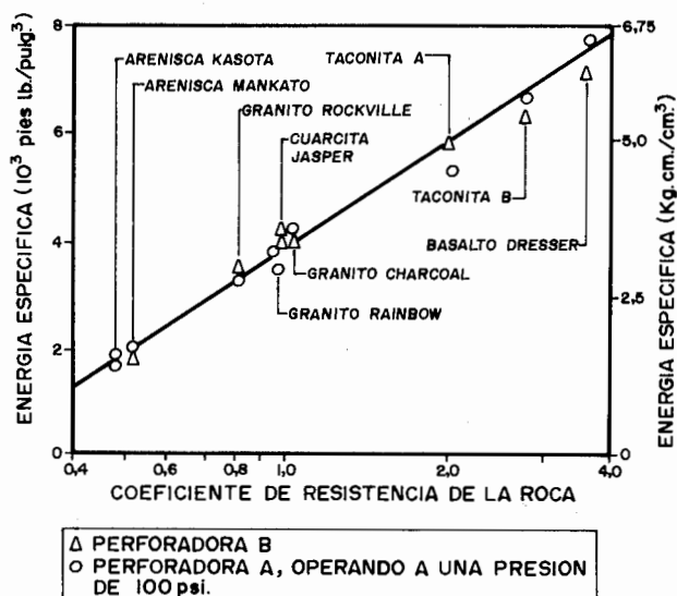
Figura 2.40. Relación entre el Coeficiente de Resistencia de la Roca y la Energía Específica.
