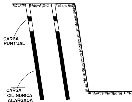
Figura 19.20. Empleo de cargas puntuales en la zona de retacado.
