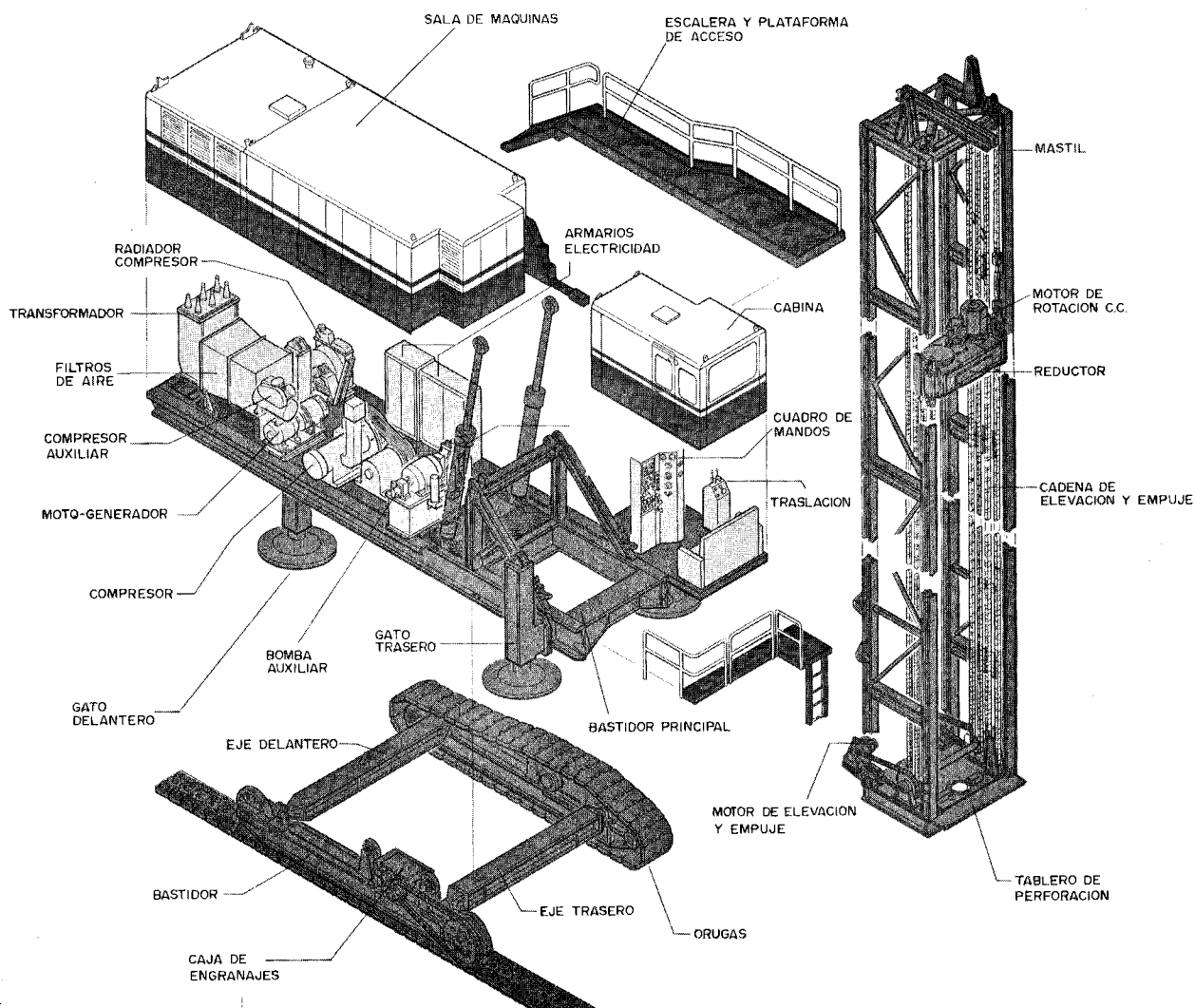
Figura 4.1. Componentes principales de una perforadora rotativa de accionamiento eléctrico (Marion).
