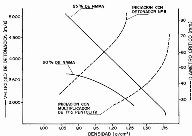
Figura 11.12. Influencia de la densidad de los hidrógeles sobre la velocidad de detonación y sensibilidad.
