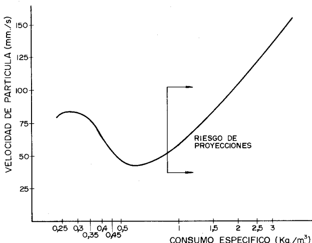
Figura 33.5. Influencia del consumo específico de explosivo en la intensidad de vibración.
