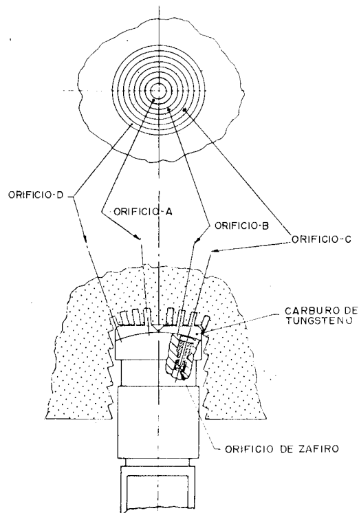
Figura 7.18. Boca de perforación con cuatro orificios.
