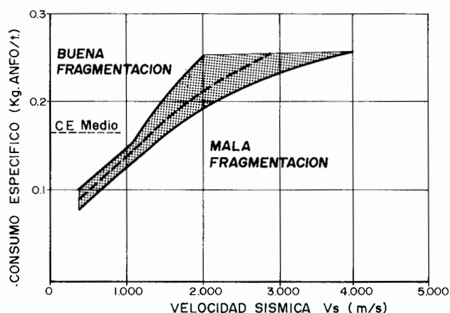
Figura 18.4. Correlación entre velocidad sísmica y consumo específico de explosivo.
