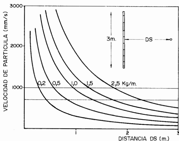
Figura 25.19. Velocidades de partícula en función de las concentraciones lineales de carga y distancias (Holmberg y otros).
