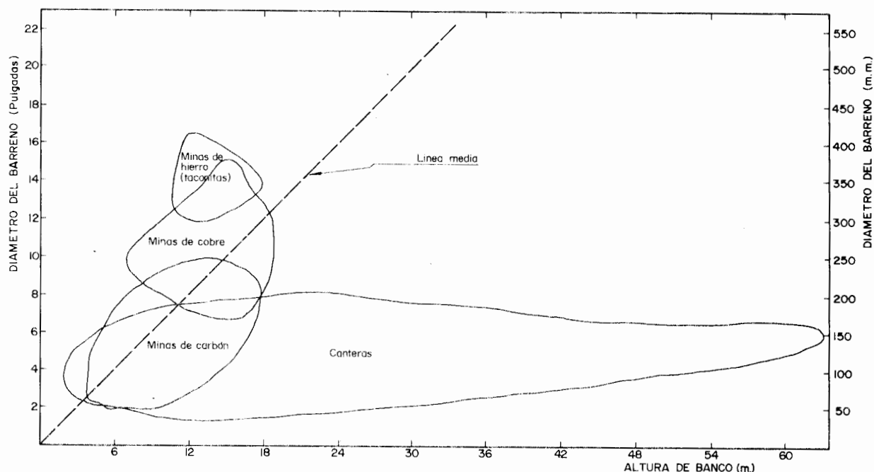
Figura 19.6. Diámetro de perforación vs. Altura de banco.
