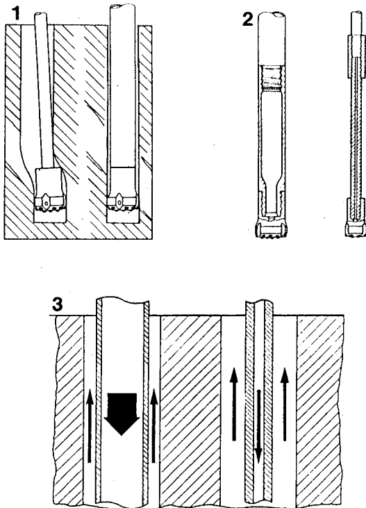
Figura 3.8. Tubos de perforación (Tamrock).
