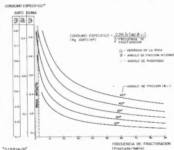
Figura 17.5. Correlación entre la frecuencia de fracturación y el consumo específico de explosivo.
