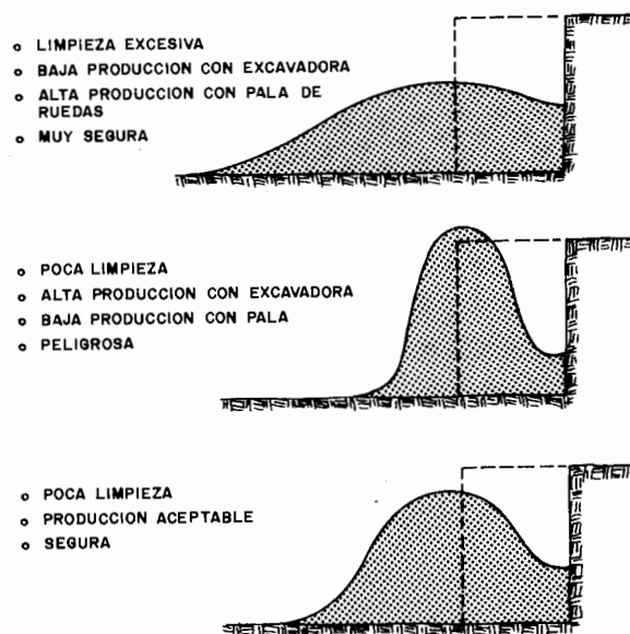
Figura 19.25. Perfiles de la pila de roca volada.
