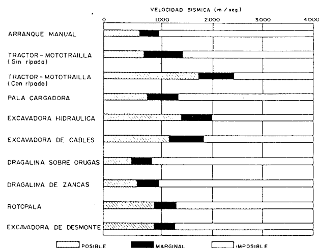
Figura 21.16. Campos de aplicación económica de equipos de arranque en función de las velocidades sísmicas.
