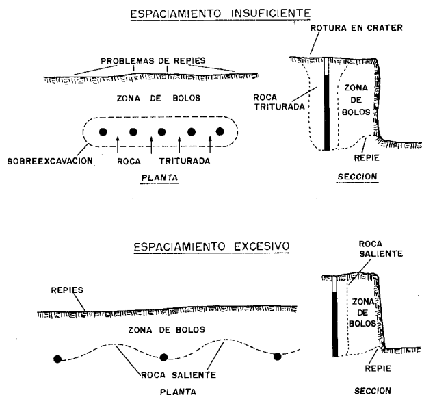
Figura 19.12. Influencia del espaciamiento en una voladura en banco (Dick y otros).
