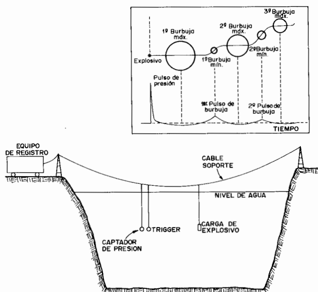
Figura 10.4. Voladuras subacuáticas para la determinación de la energía de un explosivo.
