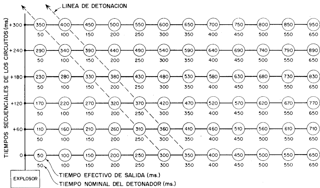
Figura 13.19. Voladura múltiple disparada con explosor secuencial.
