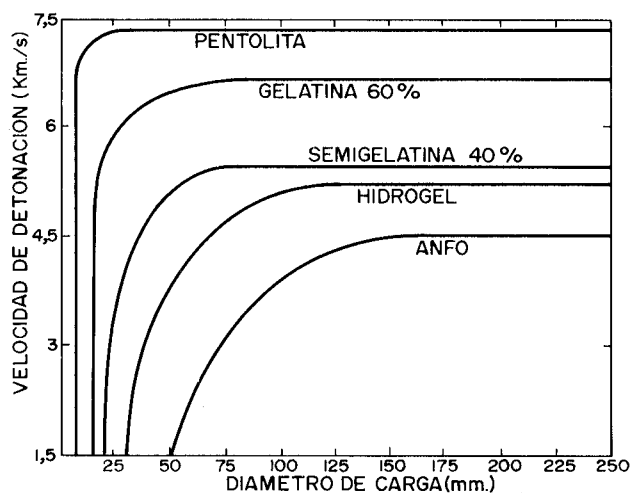
Figura 10.5. Influencia del diámetro de la carga sobre la velocidad de detonación (Ash, 1977).
