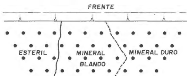
Figura 18.10. Voladura en un tajo con tres materiales de características diferentes (Hagan y Reid).
