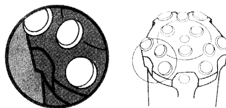
Figura 3.16. Desgaste de botones.
