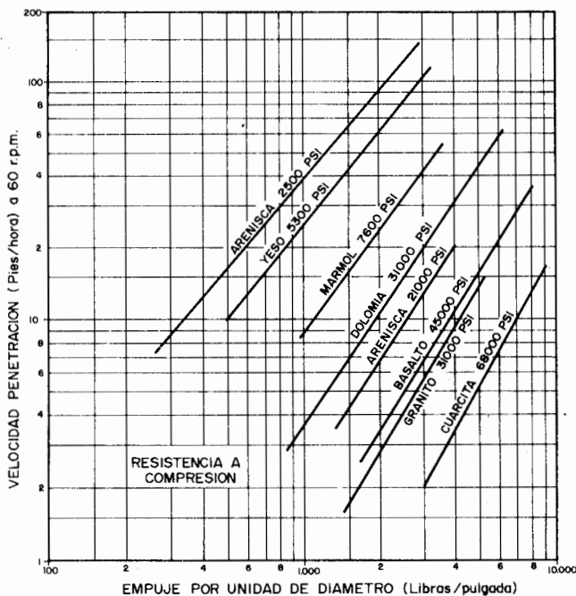
Figura 4.25. Nomograma de Velocidades de Penetración.
