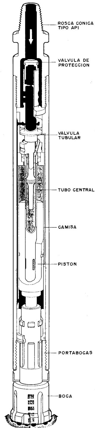
Figura 2.12. Martillo en fondo (Atlas Copco).
