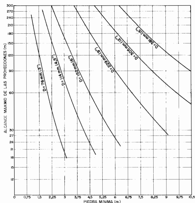
Figura 34.4. Alcances máximos de proyecciones procedentes de frentes verticales en bancos de caliza con explosivos tipo ANFO.
