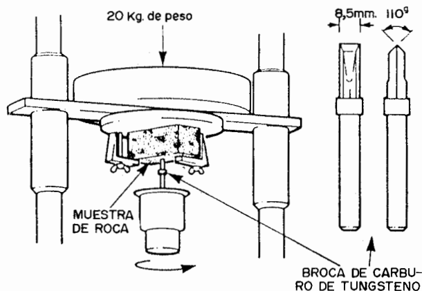
Figura 2.42. Ensayo de perforabilidad.
