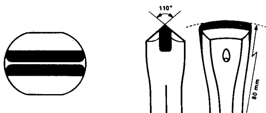
Figura 3.27. Afilado de barrenas integrales.
