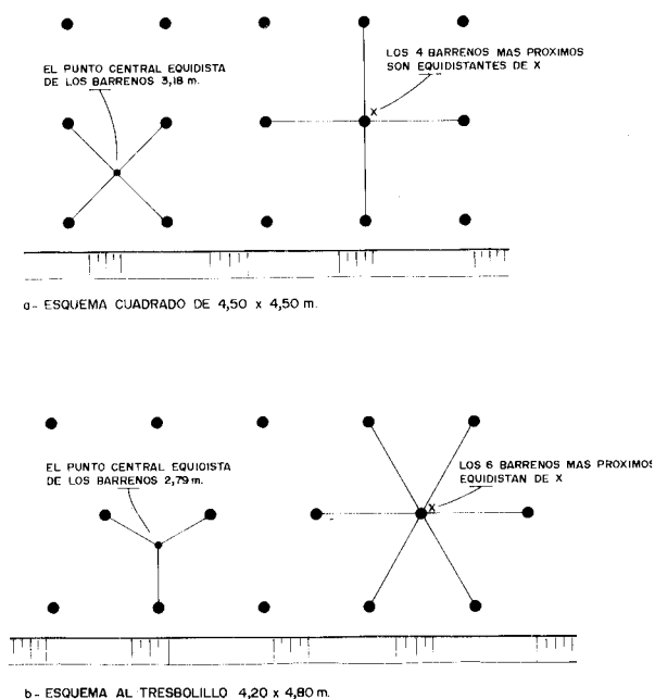
Figura 19.13. Comparación de un esquema cuadrado (a) y al tresbolillo (b).
