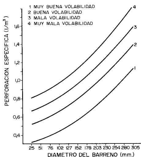
Figura 19.26. Perforación Específica de cuatro tipos de roca en bancos de 12 m de altura.
