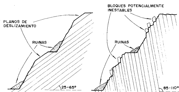
Figura 25.7. Discontinuidades con rumbo paralelo al plano de excavación.
