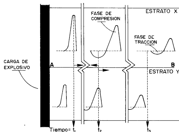
Figura 16.6. Fracturación por cizallamiento (Hagan).
