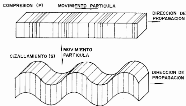
Figura 33.11. Ondas de Compresión-P y Cizallamiento-S.
