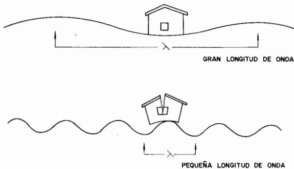
Figura 33.35. Interacción entre las edificaciones y el terreno según la longitud de onda característica.
