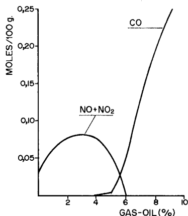
Figura 11.4. Humos producidos por diferentes porcentajes de gas-oil.
