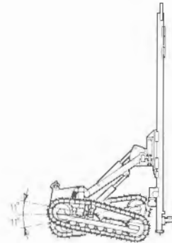
Figura 2.31. Movimiento oscilante de las orugas (Atlas Copco).
