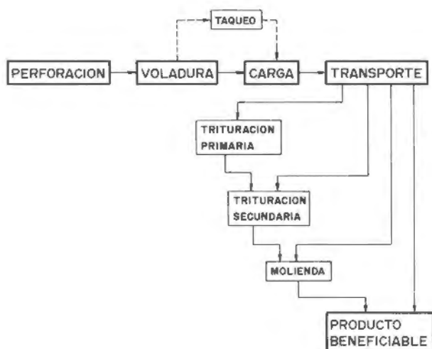
Figura 32.1. Diagrama del ciclo minero.
