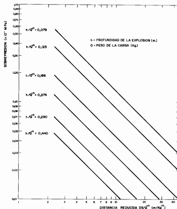
Figura 26.9. Sobrepresión aérea en voladuras subacuáticas con cargas suspendidas.
