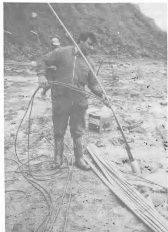
Foto 25.3. Colocación de la carga de fondo y el cordón de alto gramaje en un barreno de contorno.
