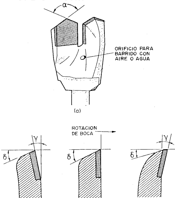
Figura 6.7. Ángulos característicos de un útil de corte (Fish y Barker, 1956).
