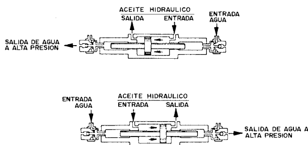
Figura 7.17. Equipo multiplicador de presión.
