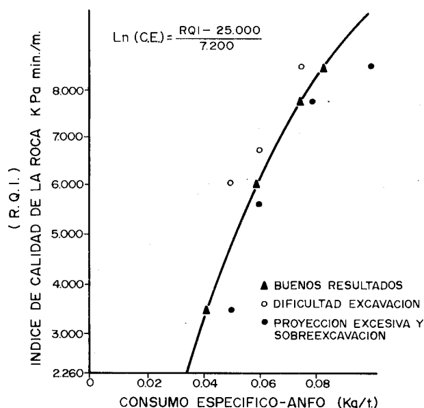
Figura 18.14. Correlación entre el «R.Q.I.» y el consumo específico (Leighton).
