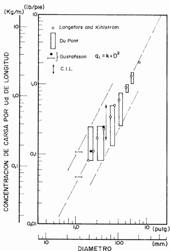
Figura 25.20. Relación entre la carga lineal de explosivo y los diámetros de perforación en voladuras de precorte y re-corte (Mellor).
