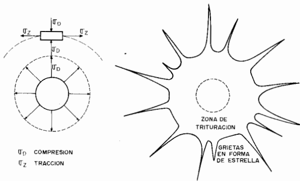
Figura 16.2. Agrietamiento radial.
