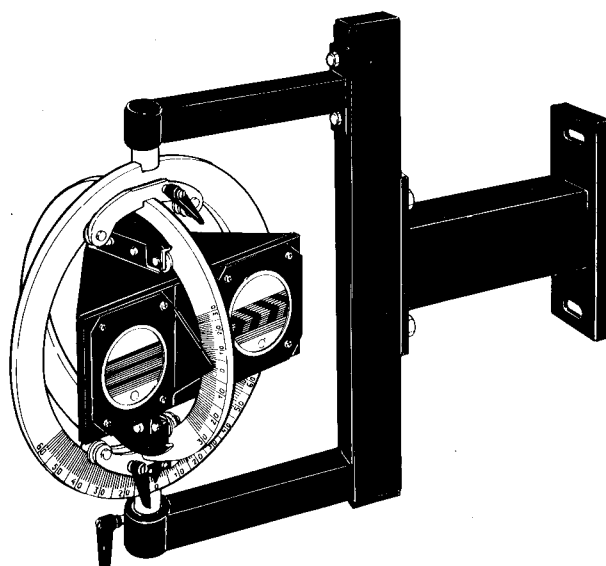
Figura 2.38. Inclinómetro.
