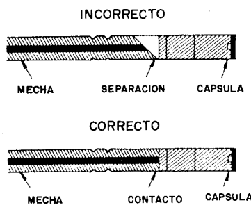
Figura 13.9. Iniciación con mecha lenta y detonador convencional.
