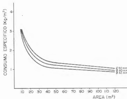
Figura 22.17. Consumo específico en función del área del túnel y diámetro de los barrenos.
