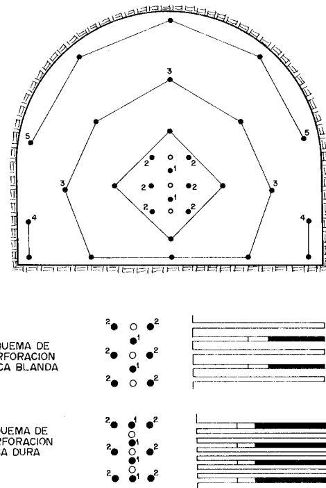
Figura 22.22. Cuele Sueco.
