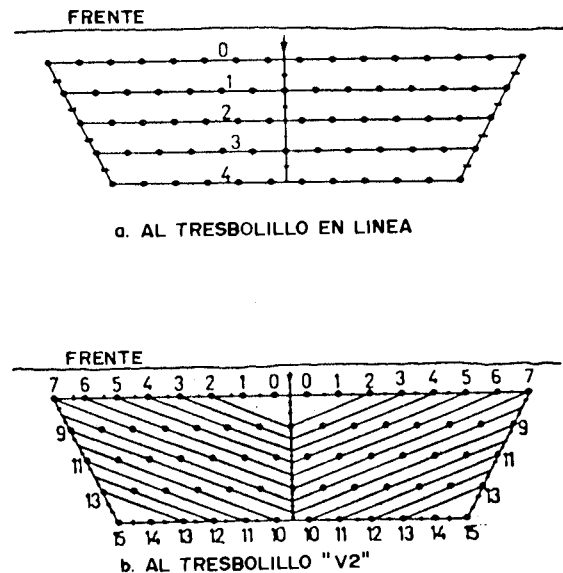
Figura 33.48. Voladuras múltiples con el mismo número de barrenos y diferentes duraciones.
