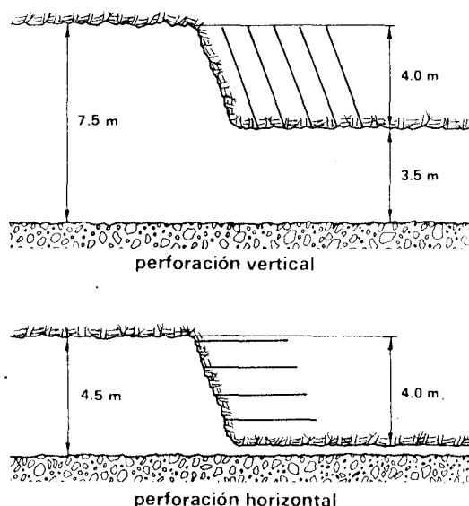
Figura 24.19. Sistemas de perforación y voladura.
