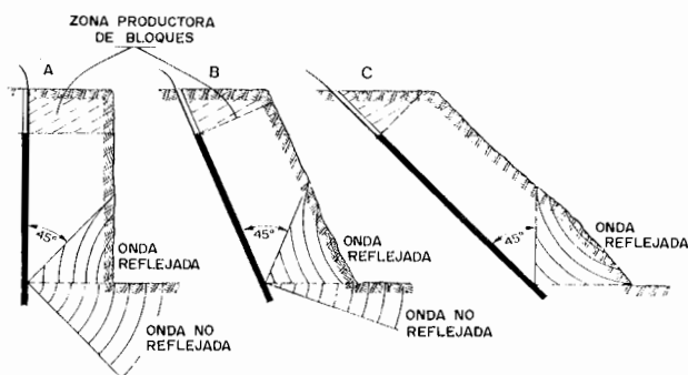
Figura 19.8. Ventajas de los barrenos inclinados.
