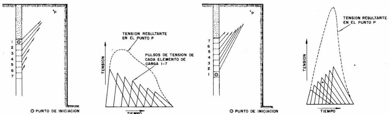
Figura 14.12. Diferentes posiciones del iniciador con cebado en cabeza (Hagan, 1974).
