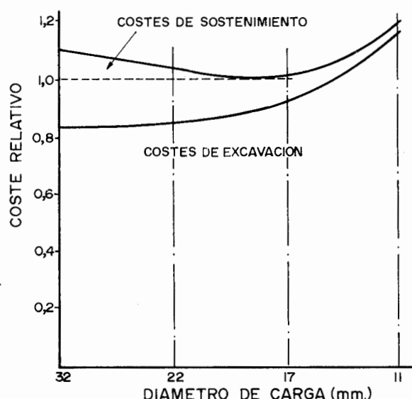
Figura 25.15. Influencia del diámetro de la carga sobre los costes de excavación y sostenimiento (Larsson y otros).
