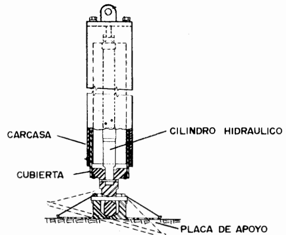
Figura 4.14. Gato hidráulico.
