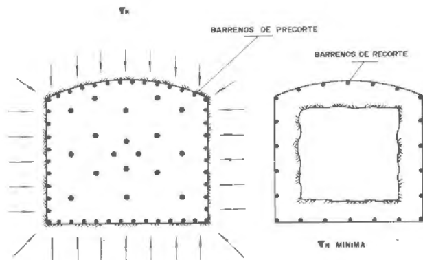
Figura 25.9. Eliminación de tensiones mediante una excavación piloto y realización parcial de un recorte (Calder y Bauer).
