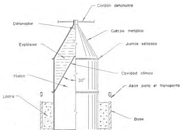
Figura 26.11. Esquema de carga hueca.
