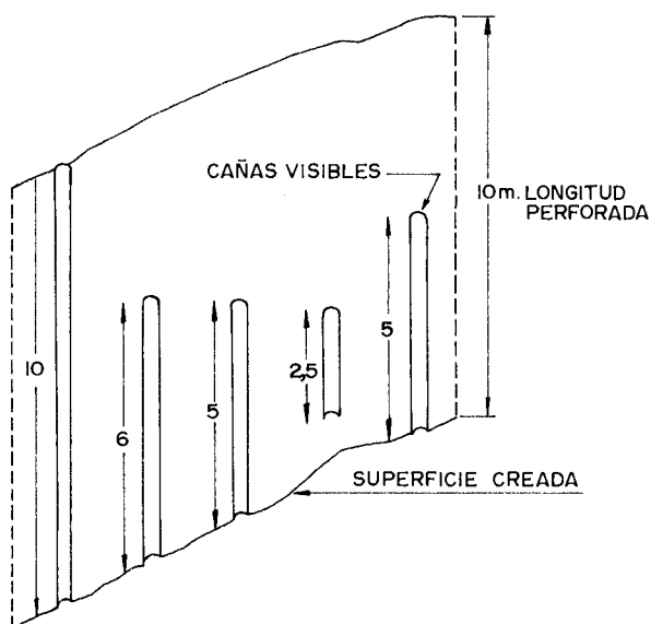
Figura 25.28. Ejemplo de cálculo del Factor de Cañas Visibles. «FCV».
