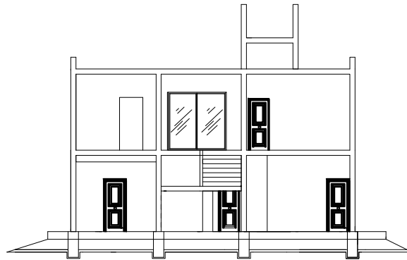
CORTE A-A
