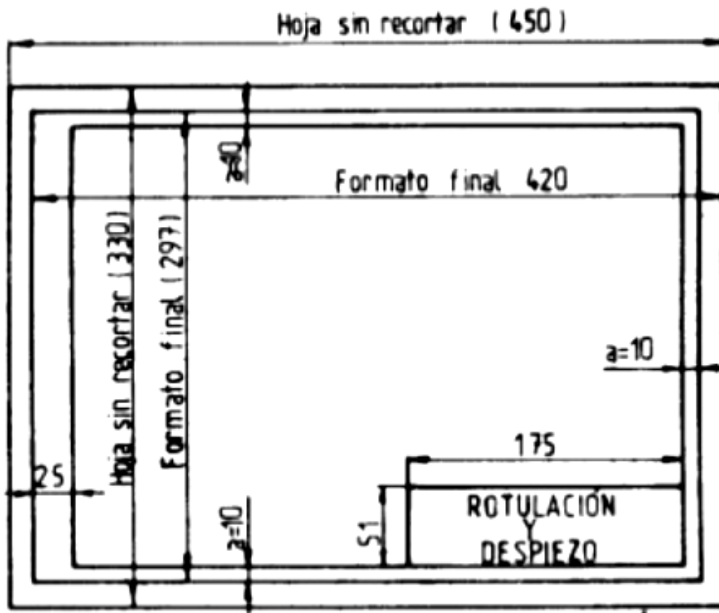
Figura 5 Ejemplo de formato A3
