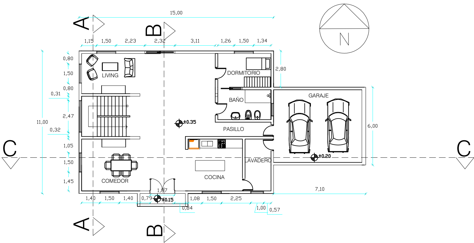
PLANTA BAJA ESCALA 1:100
