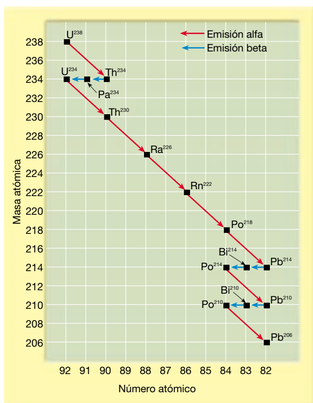
◀ Figura 9.10 El isótopo más común del uranio ( \text{U-238} ) constituye un ejemplo de serie de desintegración radiactiva. Antes de alcanzar el producto final estable ( \text{Pb-206} ), se producen muchos isótopos diferentes como etapas intermedias.
