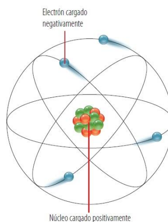
Figura 2. Modelo atómico de Rutherford, en el cual los electrones giran alrededor del núcleo del átomo.
