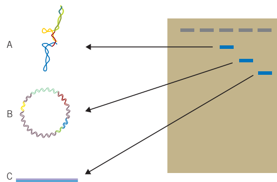
Figura 12-5. Perfil electroforético de un plásmido. Aunque la molécula de ADN (en este caso un plásmido) tenga la misma longitud en pb, puede demostrar diversos patrones de corrimiento electroforético según la conformación de la estructura. A) Plásmido superenrollado. B) Plásmido circular. C) Plásmido linealizado.
