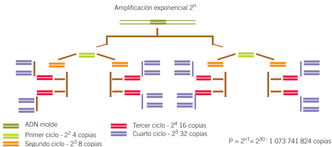
Figura 16-5. Amplificación exponencial del producto de PCR. La amplificación del producto de PCR sigue la fórmula P = (2)^n T , donde: P = número de moléculas producto del PCR; n = número de ciclos; T = número de copias inicial de la molécula molde. En cada ciclo se duplica la cantidad de producto inicial, por lo que el número de moléculas producto del PCR aumenta exponencialmente conforme avanza la reacción.
