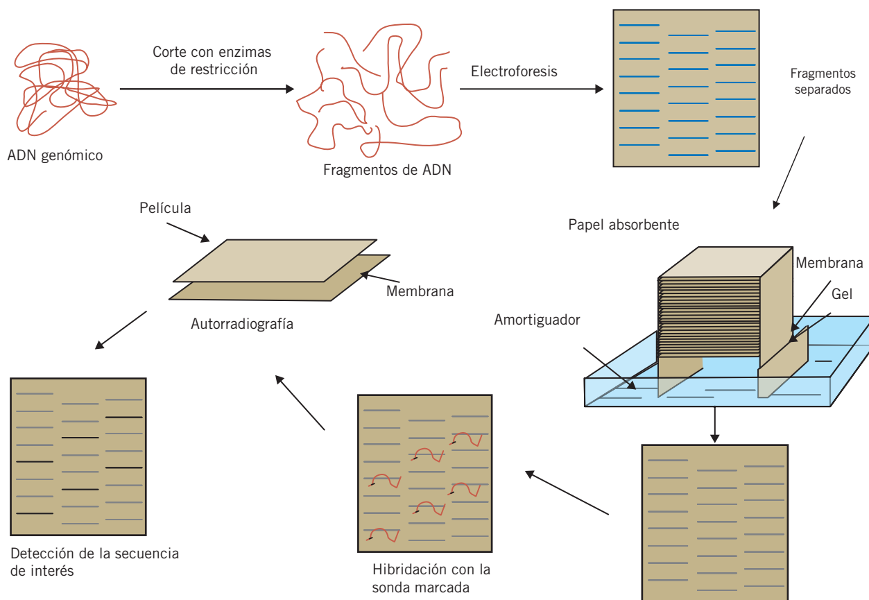
Figura 15-1. Esquema representativo de cada uno de los pasos involucrados en la técnica de Southern blot. Obtención del ADN genómico y digestión con enzimas de restricción, electroforesis, transferencia, hibridación específica con una sonda y detección de la secuencia de interés.
