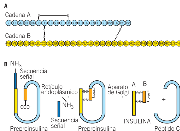
Figura 22-1. Insulina. A) Estructura de la insulina. B) Formación de la insulina humana madura a partir de la preinsulina.
