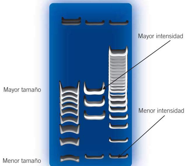
Figura 12-10. Movilidad de fragmentos de ADN. La imagen muestra fragmentos de ADN de mayor a menor tamaño (parte superior hacia parte inferior) visualizados con un agente intercalante. Se aprecia cómo la intensidad de la banda observada es variable, lo que indica grosso modo cuál fragmento se encuentra en mayor cantidad y cuál en menor.
